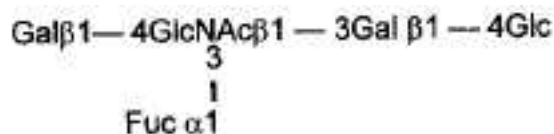
Figure 40 : Structure de LNFPIII (Thomas et coll., 2003)
