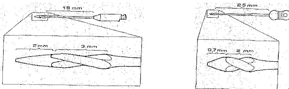
Fig. 4.8. Représentation schématique des instruments rotatifs et manuels Noter la longueur inhabituelle de la pointe mousse (D'après CAMPS et MACOUIN) (15)
