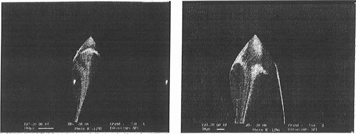
Fig. 5.7. Pointe des HERO 6 et 4 % Notez les rainures dues à l'usure
