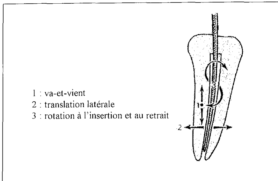
Fig. 4.10. Mouvements des limes endosonores au cours de la préparation canalaire (D'après LAURICHESSE et coll.) (51)
