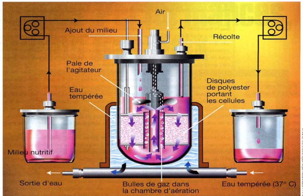
Figure n°5 : procédé Celli-Gen Plus (Emery et al., 1998)
