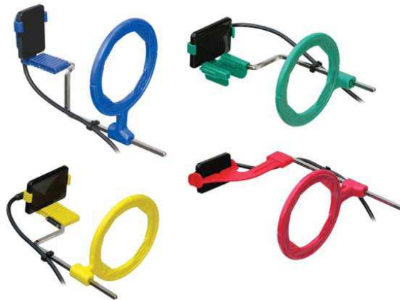
Fig.36 : Angulateurs pour capteur numérique [59]
