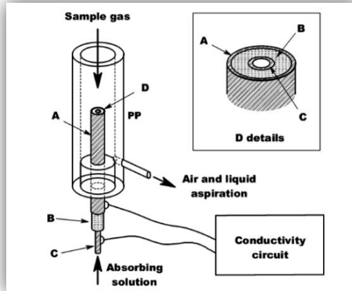
Figure 28. Schéma explicatif du capteur (D'après Toda et al. 2006 [75])
