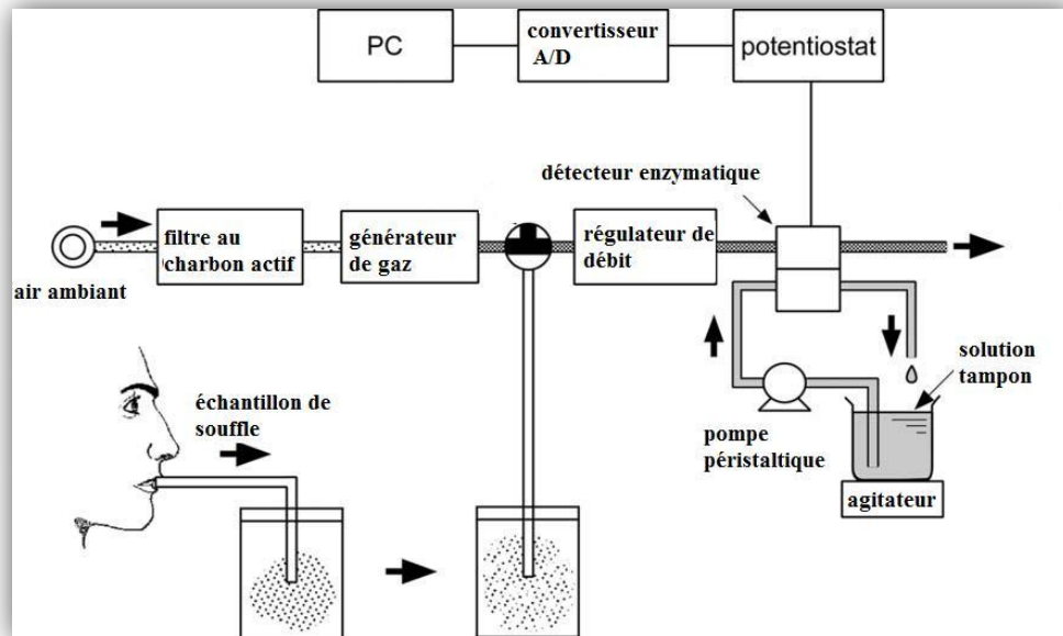
Figure 24. Diagramme schématique du bio-détecteur enzymatique à base de MAO-A (D'après Minamide et al. 2005 [70])
