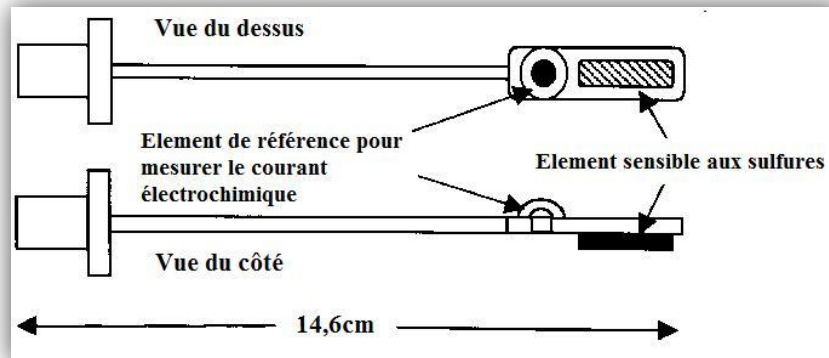
Figure 22. Diagramme de la sonde linguale à sulfures (D'après Morita et al. 2001 [66])
