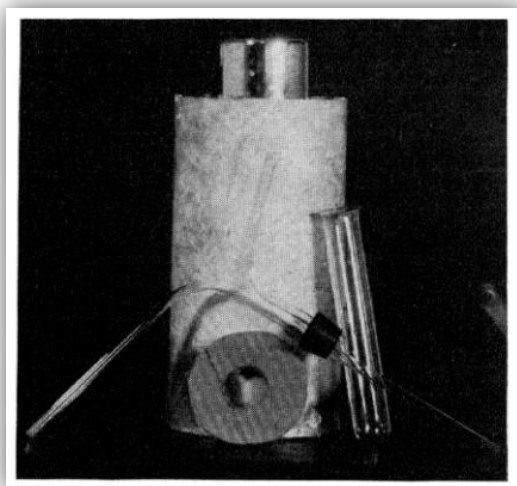
Figure 29. Cryo-osmoscope (D'après Brening et al. 1939 [11])
