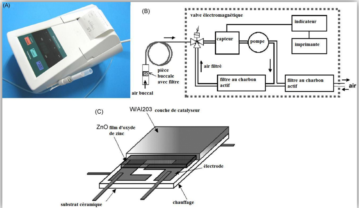
Figure 23. Diagramme schématique de Breathtron® (D'après Tanda et al. 2007 [67])
