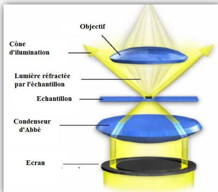
Figure 36. Schéma de fonctionnement d'un microscope optique à fond noir
