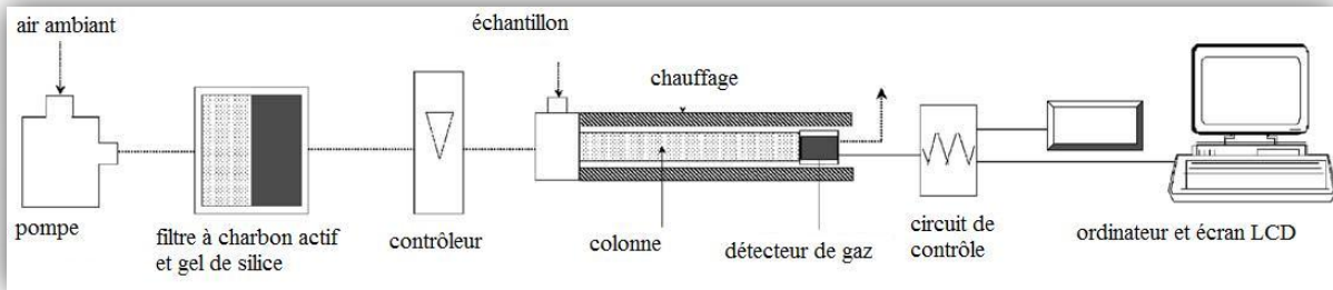
Figure 16. Schéma du détecteur (D'après Hanada et al. 2003 [63])
