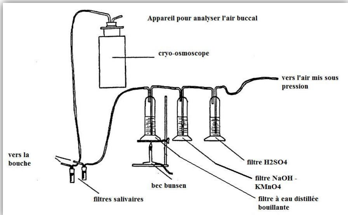
Figure 30. Schéma explicatif du cryo-osmoscope (D'après Brening et al. 1939 [11])
