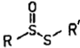
Figure 31 : Structure générale des thiosulfates
