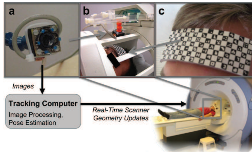
FIGURE 1.7 – Méthode de suivi de mouvement à base d'une seule caméra et d'un marquer codé[11]
