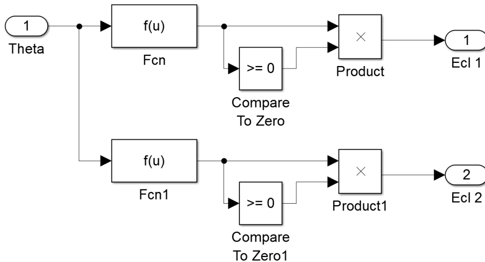
FIGURE 4.3: Bloc éclairement
