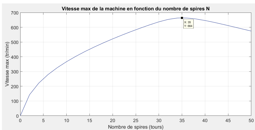
FIGURE D.3: Évolution de la vitesse max en fonction du nombre de spires N [2V - 380mA](304 K)
