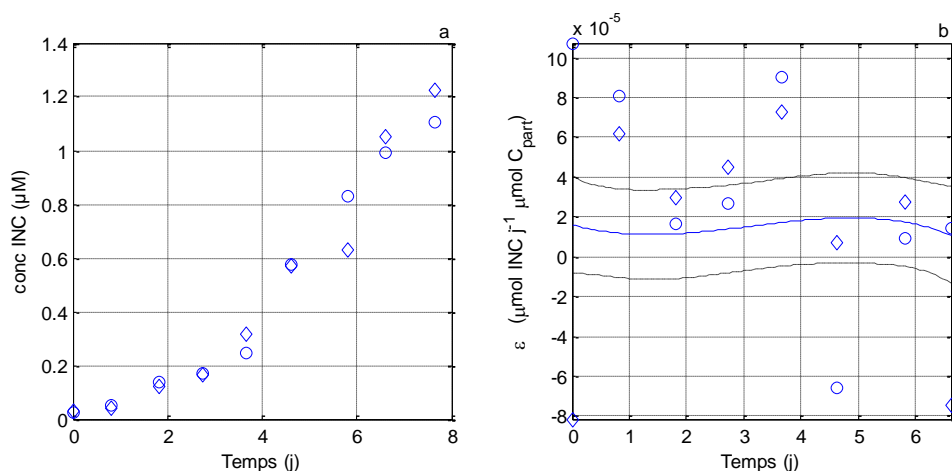
FIGURE 16 : Evolution des variables mesurées au cours des cultures en P limitant des réplicats 1 (○) et 2 (◇). (a) concentration de l'inconnu ( \mu\text{M} ) ; (b) Taux d'excrétion du composé inconnu ; (--) intervalle de confiance à 95 %
