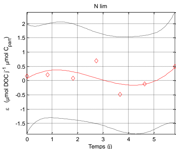
FIGURE 10 : Taux d'excrétion du carbone organique dissous en azote limitant; en rouge : réplicat (2) en N limitant; (--) intervalle de confiance à 95 %
