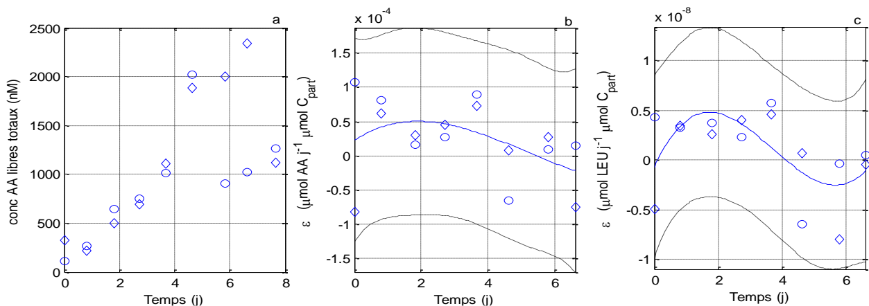
FIGURE 14 : Evolution des variables mesurées au cours des cultures limitées par le P des répliquats 1 (o) et 2 (◇). (a) concentration en acides aminés libres totaux ; (b) Taux d'excrétion des acides aminés libres ; (c) Taux d'excrétion de la leucine ; (--) intervalle de confiance à 95 %
