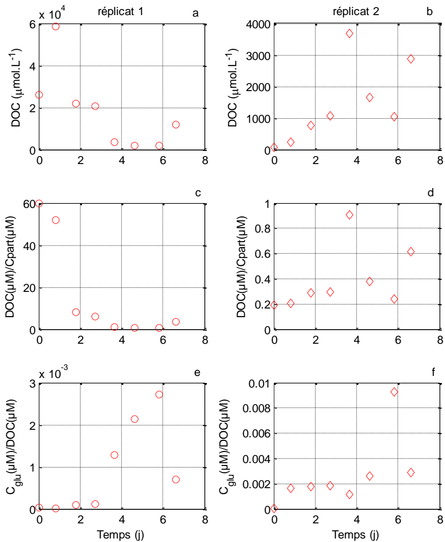
FIGURE 9 : Evolution des variables mesurées au cours des cultures limitées par le N des réplicats 1 (o) et 2 (d). (a), (b) carbone organique dissous ; (c), (d) DOC/Carbone particulaire ; (e), (f) Carbone glucidique dissous/carbone organique dissous
