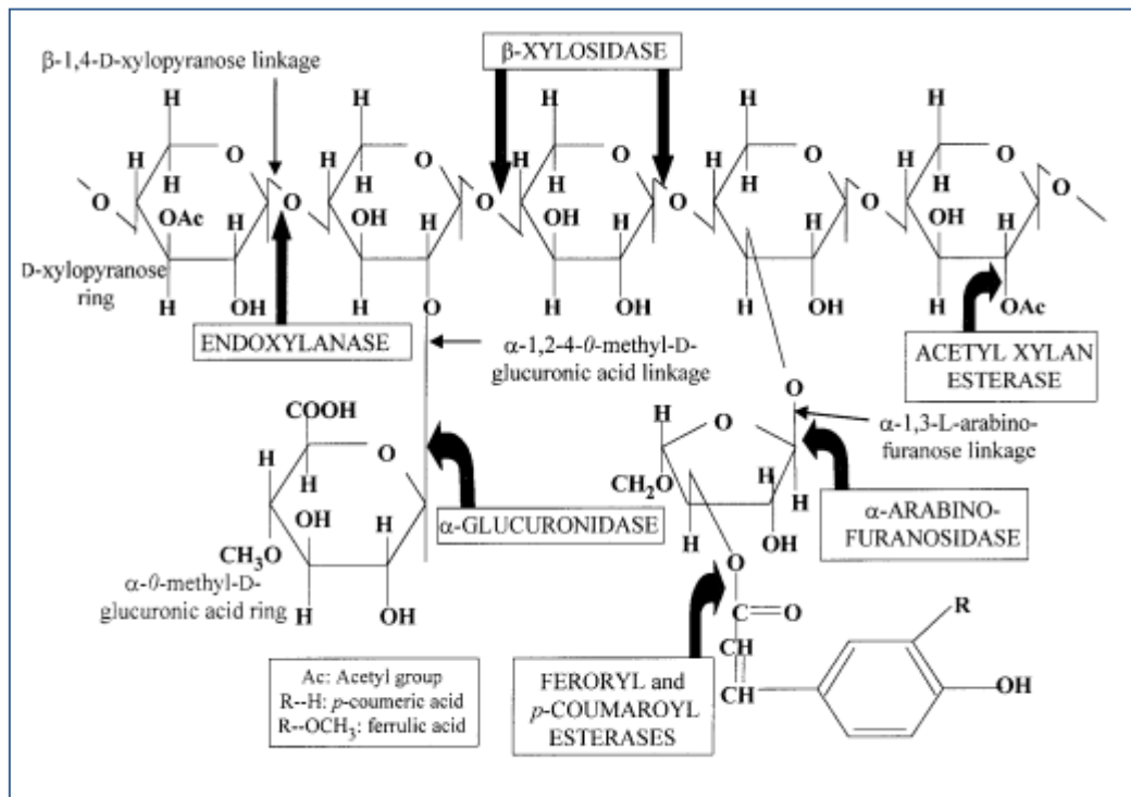
Figure 4: Structure hypothétique de xylanes avec les sites de coupe par les différentes xylanases (Q. K. Beg, 2001)
