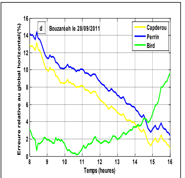
Figure (5d) : Err moy relative au global horizontal
