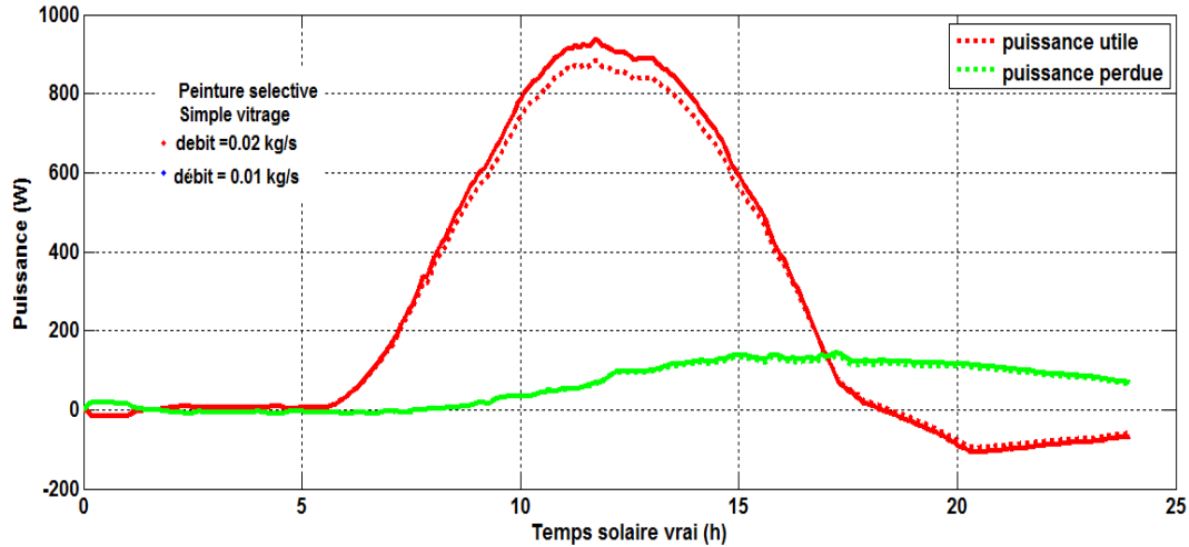
Figure (6-34) : Effet du débit du fluide caloporteur sur l'évolution des différentes puissances mises en jeu dans le capteur
