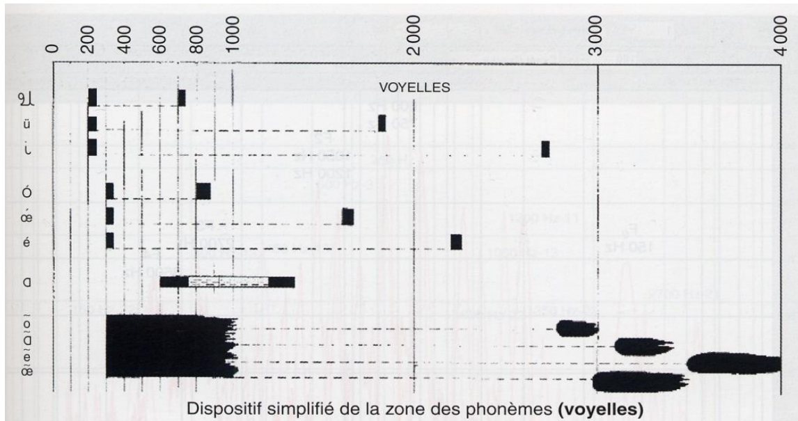
Figure 4 : Acougramme phonétique de Mme Borel- Maisonny [1]
