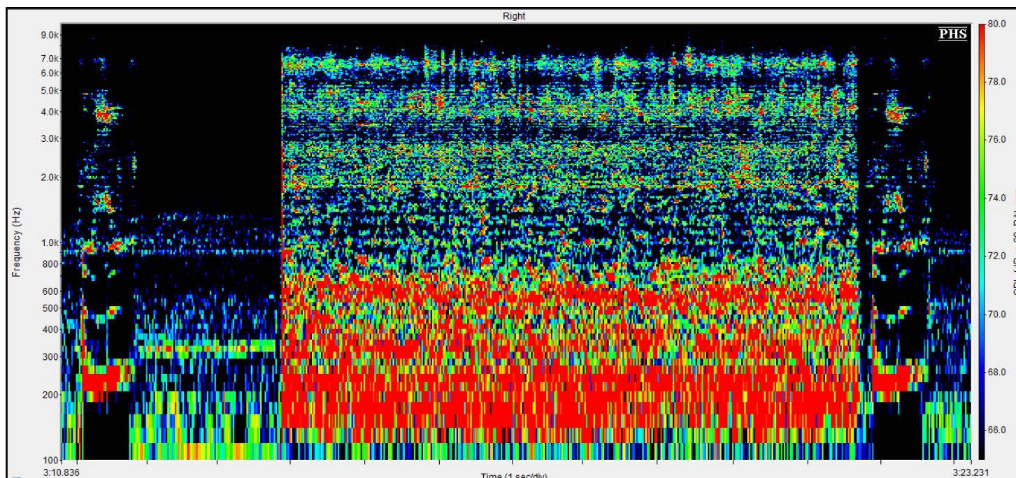
Figure n°250 : Spectrogramme du logatome « ouzo » 5 s de silence, puis 5 s de bruit de restaurant puis 0,1 s de silence et de nouveau le logatome « ouzo » émis à 70 dB à l'azimut 0°, avec un RSB de 0 dB, obtenu avec la compression Syllabic
