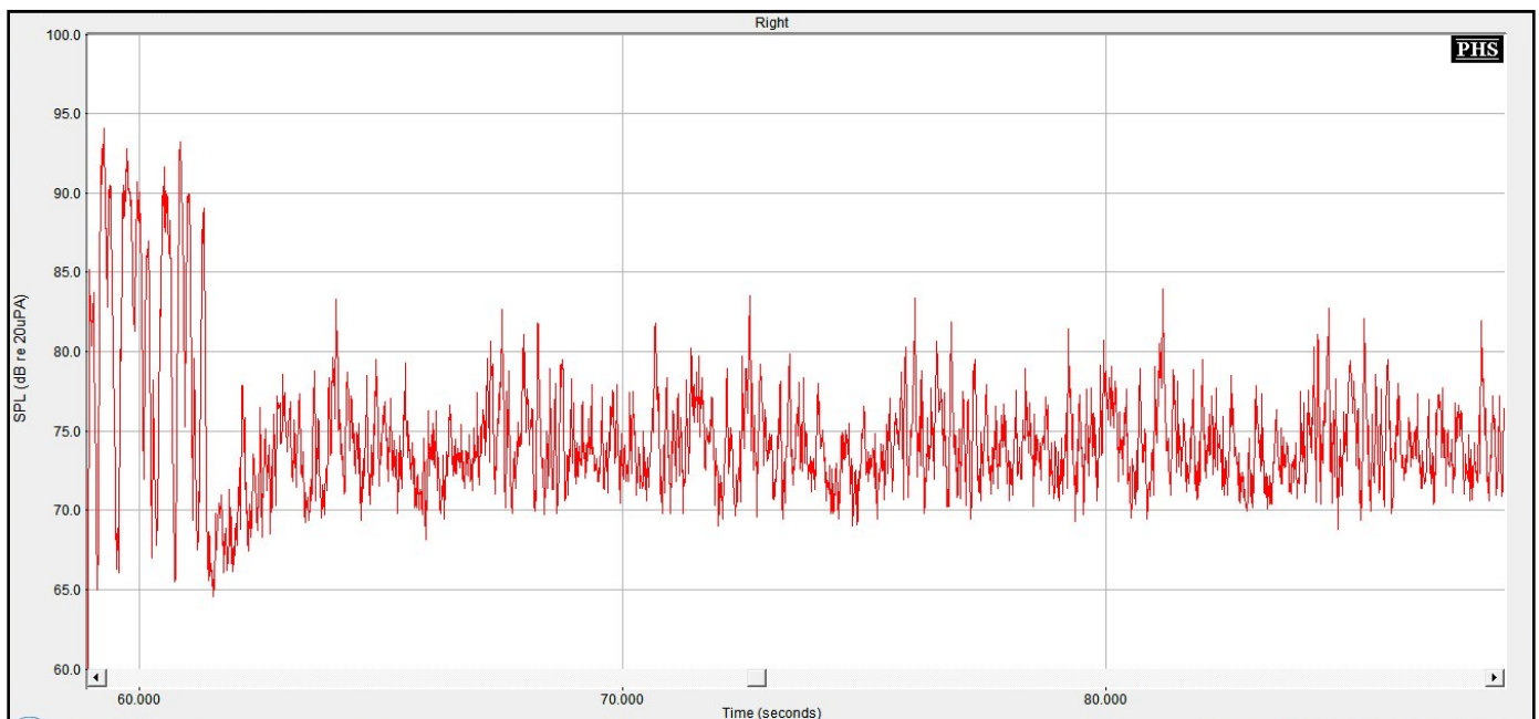
Figure n°94 : Zoom de la représentation temporelle du bruit de restaurant émis à 55 dB et d'un signal de parole de 15 s à voix forte, provenant tous deux de l'azimut 0°, obtenu avec le programme P2, Dual et Ck à 20 dB, Réducteur de bruit réglé par bandes
