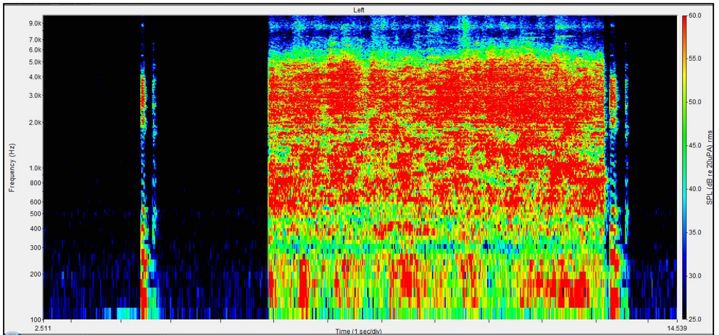
Figure n°195 : Spectrogramme du mot « pipe », 5 s de silence, puis 5 s de bruit de cris d'enfants puis 0,1 s de silence et de nouveau le mot « pipe » émis à 70 dB à l'azimut 0°, avec un RSB de 0 dB, obtenu oreille nue du KEMAR
