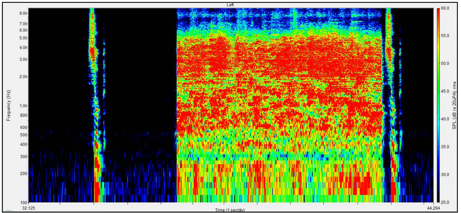
Figure n°201 : Spectrogramme du mot « soupe », 5 s de silence, puis 5 s de bruit de cris d'enfants puis 0,1 s de silence et de nouveau le mot « soupe » émis à 70 dB à l'azimut 0°, avec un RSB de 0 dB, obtenu oreille nue du KEMAR
