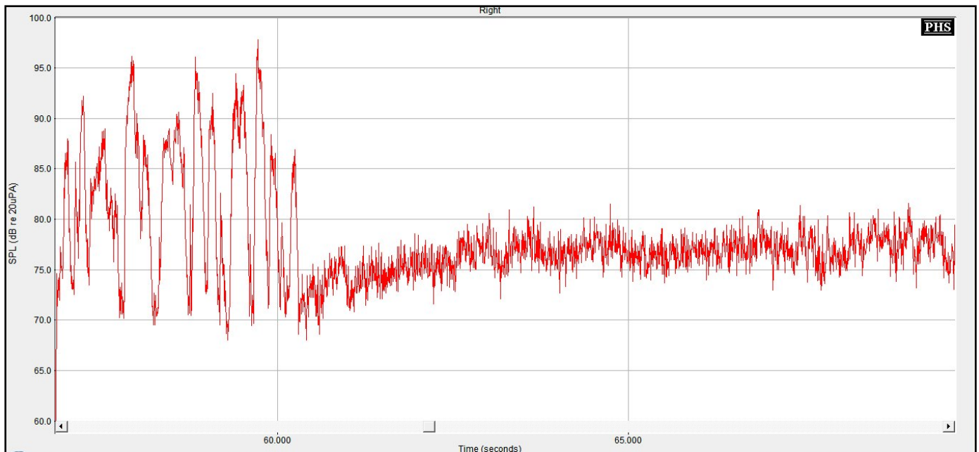
Figure n°307 : Zoom de la représentation temporelle du bruit de rame de métro émis à 55 dB et d'un signal de parole de 15 s à voix forte, provenant tous deux de l'azimut 0°, obtenu avec le programme P1, Dual et Ck dégressifs, Réducteur de bruit réglé au maximum
