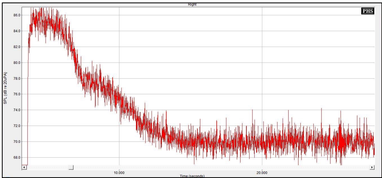
Figure n°144 : Représentation temporelle de l'action du réducteur de bruit réglé en bande large au maximum sur un bruit blanc, émis à 60 dB SPL
