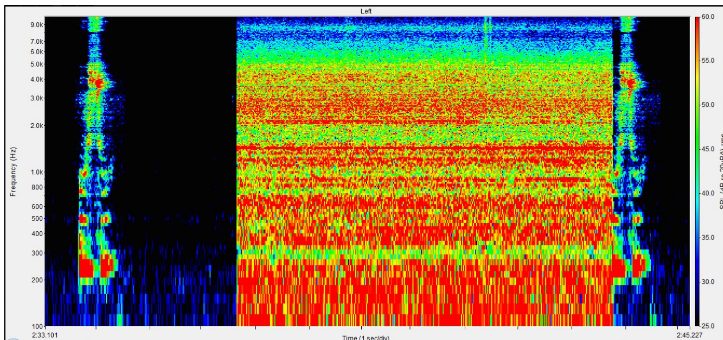
Figure n°279 : Spectrogramme du logatome « oussou » 5 s de silence, puis 5 s de bruit de rame de métro puis 0,1 s de silence et de nouveau le logatome « oussou » émis à 70 dB à l'azimut 0°, avec un RSB de 0 dB, obtenu oreille nue du KEMAR
