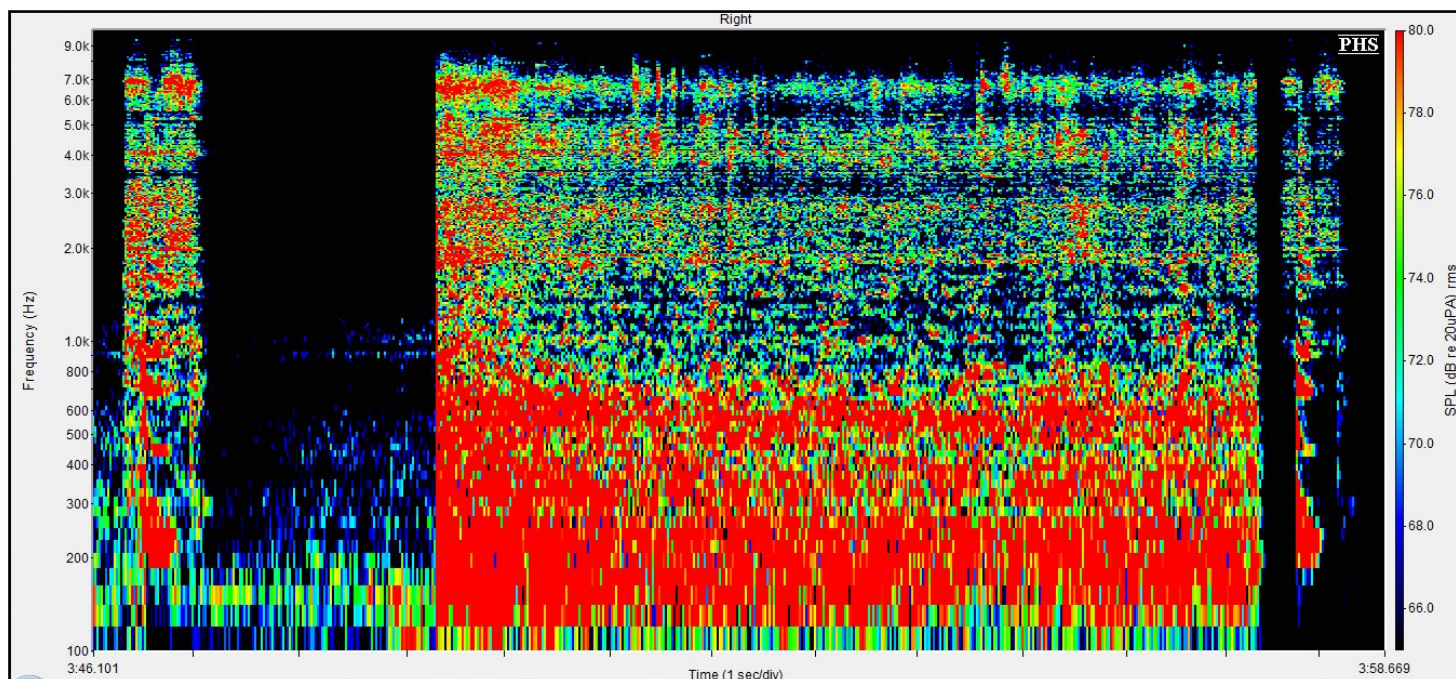
Figure n°257 : Spectrogramme du logatome «faf» 5 s de silence, puis 5 s de bruit de restaurant puis 0,1 s de silence et de nouveau le logatome « faf» émis à 70 dB à l'azimut 0°, avec un RSB de 0 dB, obtenu avec la compression Dual
