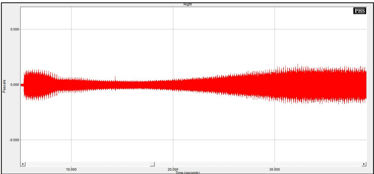
Figure n°130 : Représentation temporelle de l'action du réducteur de bruit réglé en bande large au maximum sur un son wobulé de 1000 Hz, émis à 50 dB SPL
