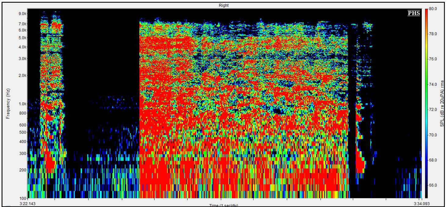
Figure n°224 : Spectrogramme du logatome « faf », 5 s de silence, puis 5 s de bruit de cris d'enfants puis 0,1 s de silence et de nouveau le logatome « faf » émis à 70 dB à l'azimut 0°, avec un RSB de 0 dB, obtenu avec la compression Dual
