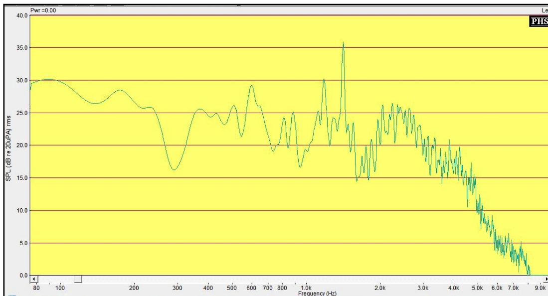
Figure n°19 : Spectre du bruit de rame de métro après moyennage (500)
