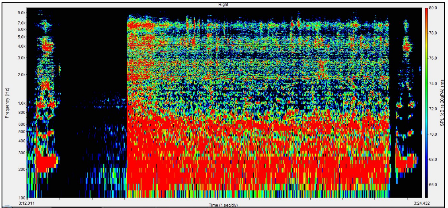
Figure n°251 : Spectrogramme du logatome « ouzo » 5 s de silence, puis 5 s de bruit de restaurant puis 0,1 s de silence et de nouveau le logatome « ouzo » émis à 70 dB à l'azimut 0°, avec un RSB de 0 dB, obtenu avec la compression Dual
