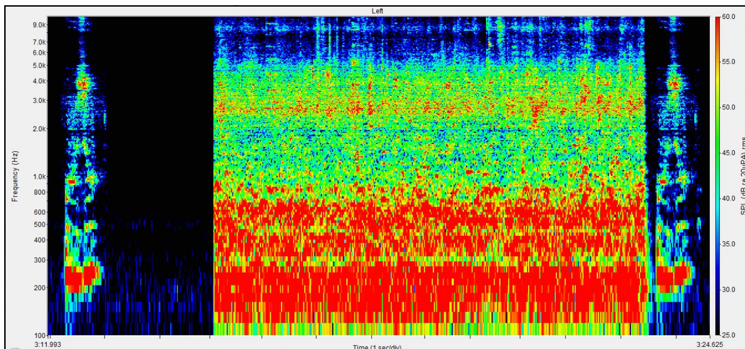
Figure n°249 : Spectrogramme du logatome « ouzo » 5 s de silence, puis 5 s de bruit de restaurant puis 0,1 s de silence et de nouveau le logatome « ouzo » émis à 70 dB à l'azimut 0°, avec un RSB de 0 dB, obtenu oreille nue du KEMAR
