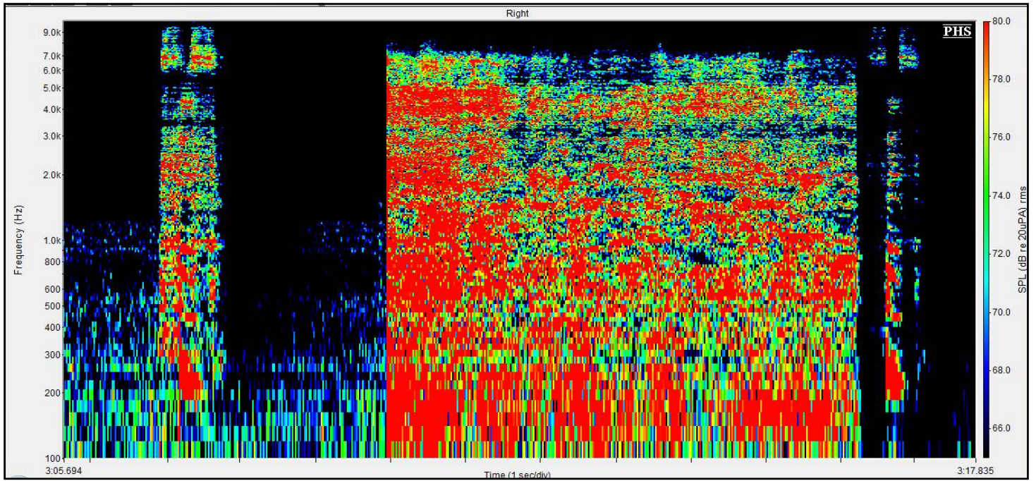
Figure n°221 : Spectrogramme du logatome « sasse », 5 s de silence, puis 5 s de bruit de cris d'enfants puis 0,1 s de silence et de nouveau le logatome « sasse» émis à 70 dB à l'azimut 0°, avec un RSB de 0 dB, obtenu avec la compression Dual
