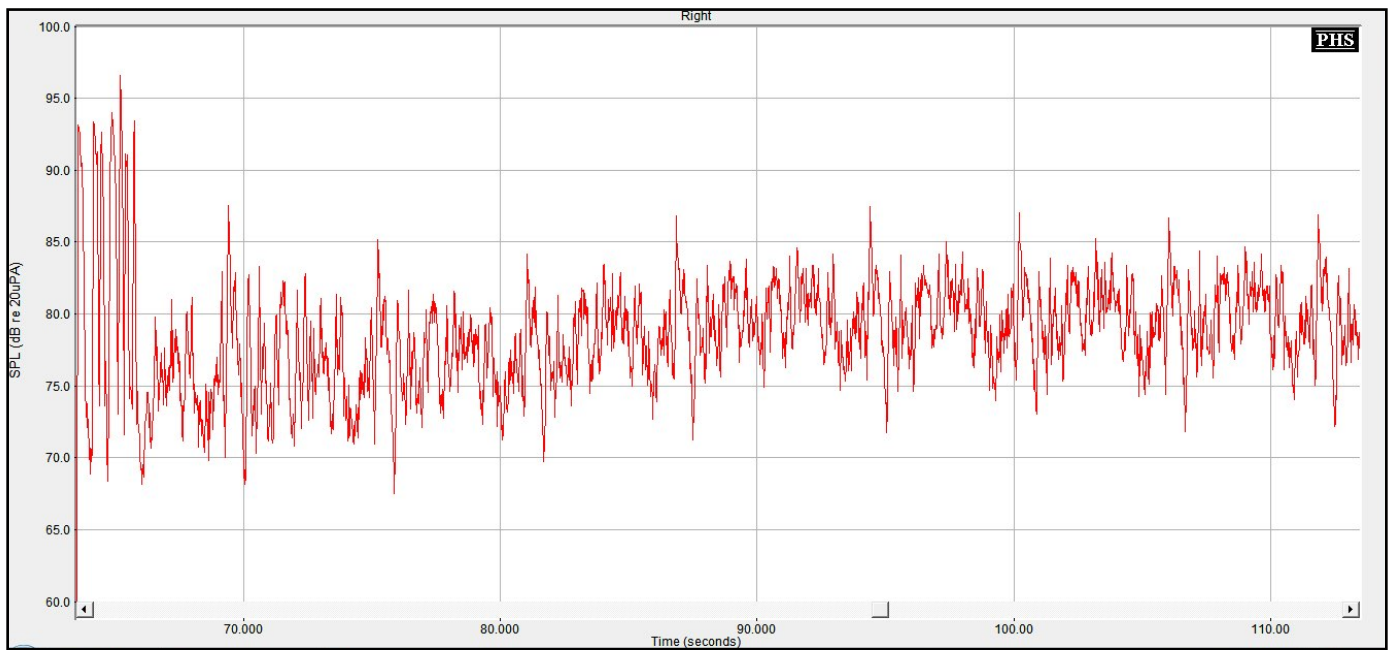
Figure n°98 : Zoom de la représentation temporelle du bruit de cris d'enfants émis à 55 dB et d'un signal de parole de 15 s à voix forte, provenant tous deux de l'azimut 0°, obtenu avec le programme P2, Dual et Ck à 20 dB, Réducteur de bruit réglé par bandes
