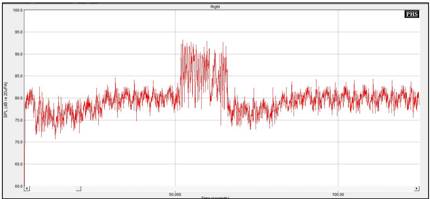
Figure n°99 : Représentation temporelle du bruit de cris d'enfants émis à 55 dB et d'un signal de parole de 15 s à voix forte, provenant tous deux de l'azimut 0°, obtenue avec le programme P3, Syllabic et Ck à 20 dB, Réducteur de bruit réglé par bandes
