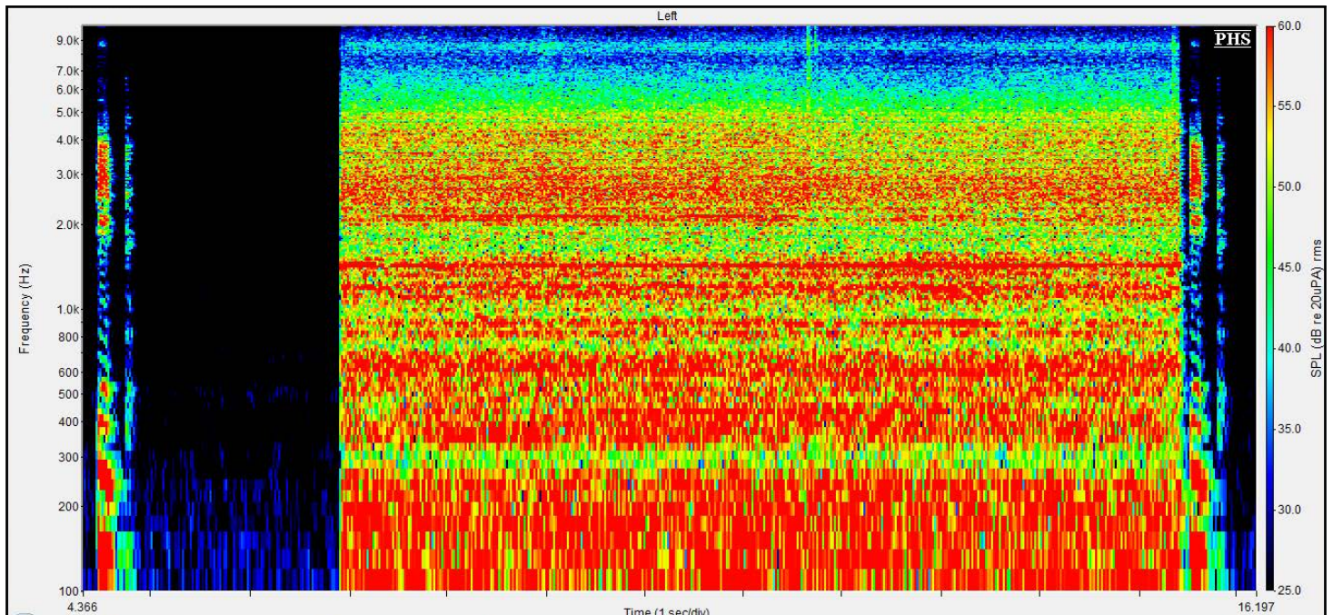
Figure n°261 : Spectrogramme du mot « pipe » 5 s de silence, puis 5 s de bruit de rame de métro puis 0,1 s de silence et de nouveau le mot « pipe » émis à 70 dB à l'azimut 0°, avec un RSB de 0 dB, obtenu oreille nue du KEMAR
