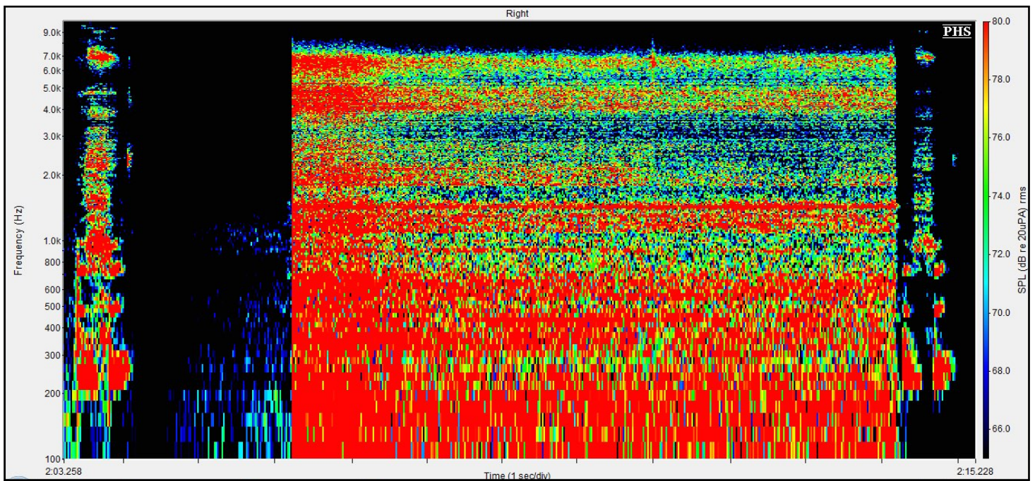
Figure n°278 : Spectrogramme du logatome « oufou » 5 s de silence, puis 5 s de bruit de rame de métro puis 0,1 s de silence et de nouveau le logatome « oufou » émis à 70 dB à l'azimut 0°, avec un RSB de 0 dB, obtenu avec la compression Dual
