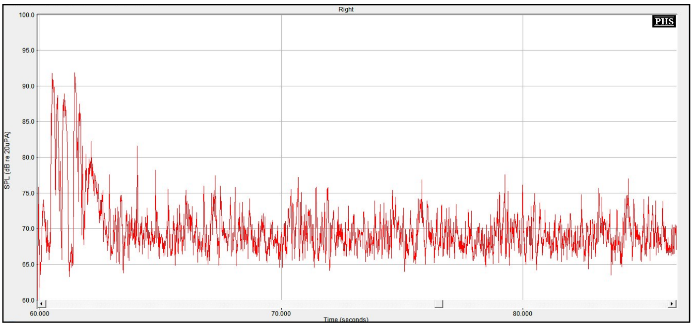
Figure n°108 : Zoom de la représentation temporelle du bruit de restaurant émis à 55 dB et d'un signal de parole de 15 s à voix forte, provenant tous deux de l'azimut 0°, obtenu avec le programme P3, Syllabic et Ck à 20 dB, Réducteur de bruit réglé au maximum
