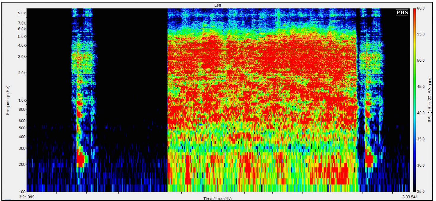
Figure n°222 : Spectrogramme du logatome « faf », 5 s de silence, puis 5 s de bruit de cris d'enfants puis 0,1 s de silence et de nouveau le logatome « faf» émis à 70 dB à l'azimut 0°, avec un RSB de 0 dB, obtenu oreille nue du KEMAR
