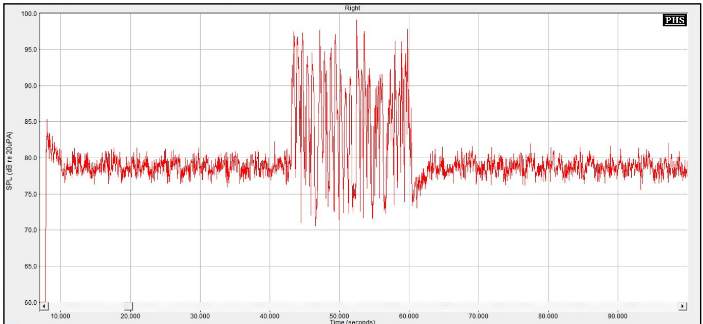
Figure n°306 : Représentation temporelle du bruit de rame de métro émis à 55 dB et d'un signal de parole de 15 s à voix forte, provenant tous deux de l'azimut 0°, obtenue avec le programme P1, Dual et Ck dégressifs, Réducteur de bruit réglé au maximum
