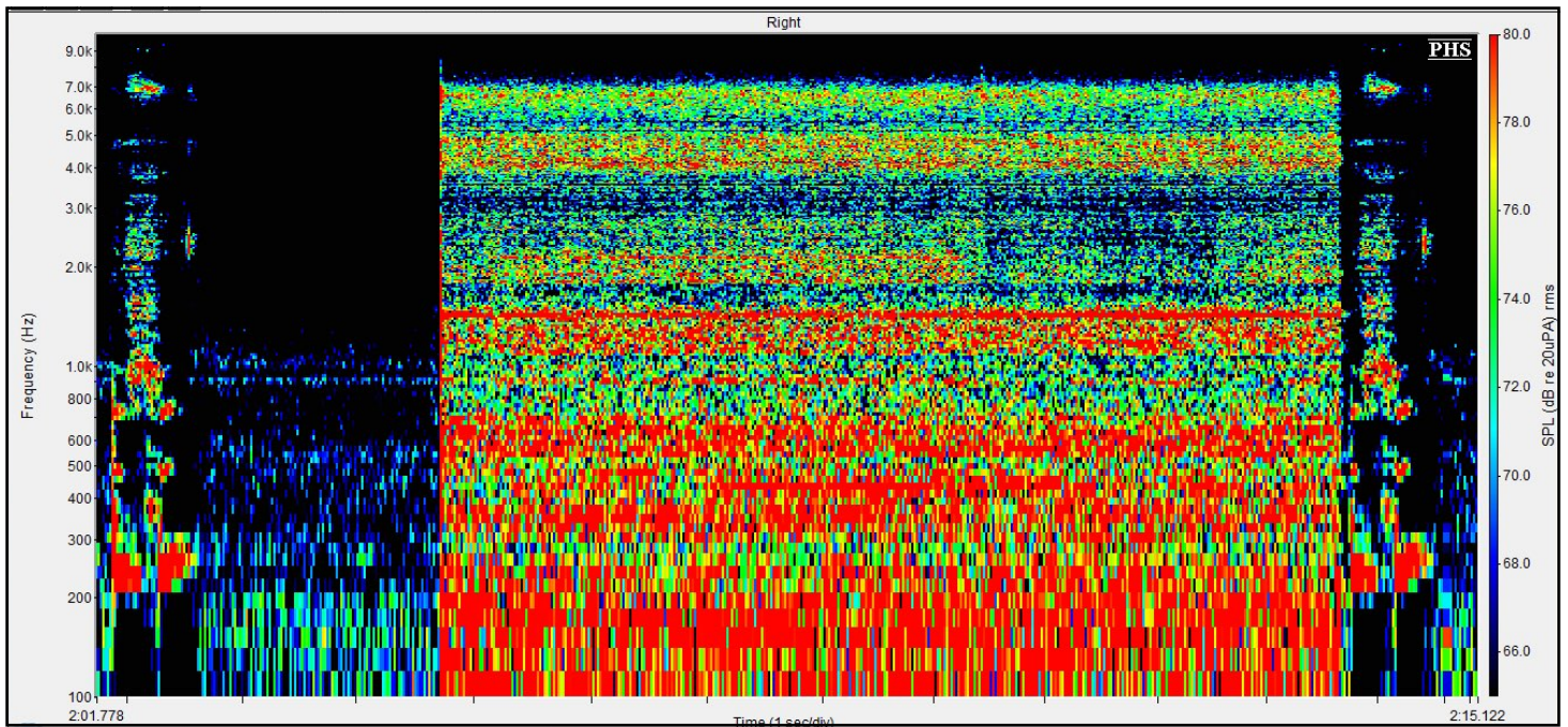
Figure n°277 : Spectrogramme du logatome « oufou » 5 s de silence, puis 5 s de bruit de rame de métro puis 0,1 s de silence et de nouveau le logatome « oufou » émis à 70 dB à l'azimut 0°, avec un RSB de 0 dB, obtenu avec la compression Syllabic
