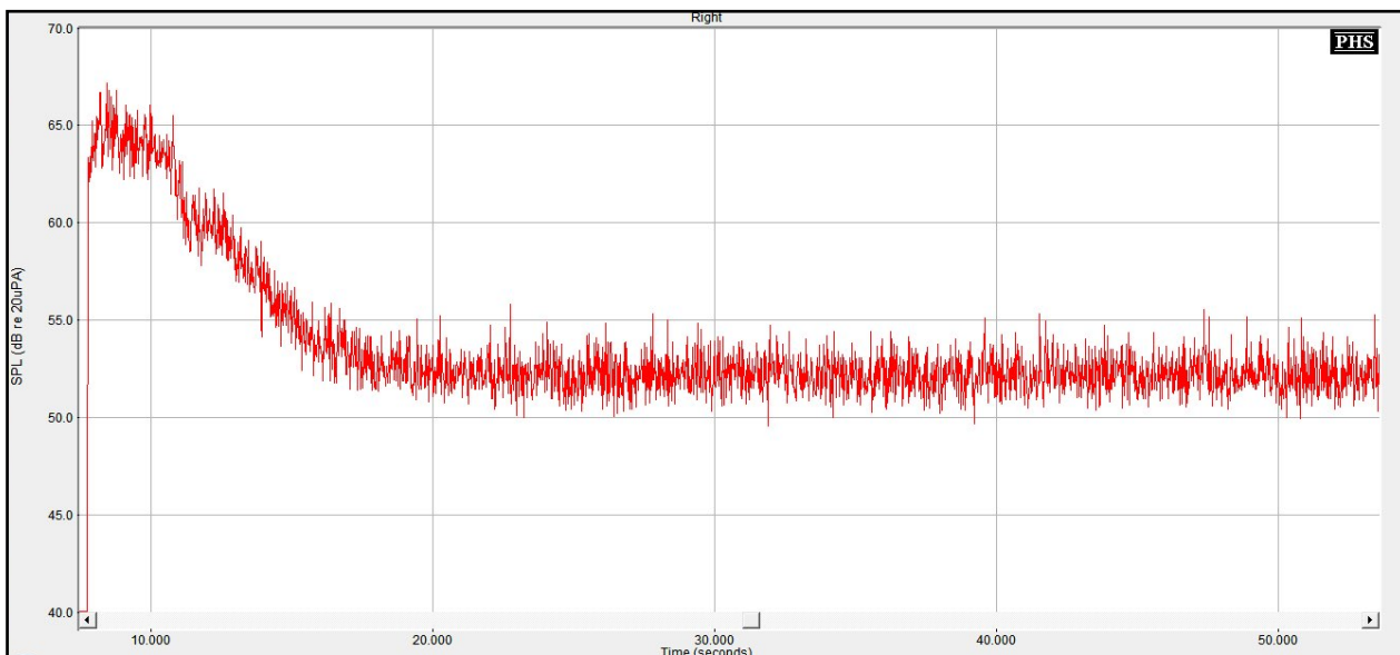
Figure n°150 : Représentation temporelle de l'action du réducteur de bruit réglé en bande large au maximum sur un bruit blanc émis à 55 dB SPL quand l'appareil possède un gain de 20 dB, un taux de compression de 1,5 et des Ck à 20 dB
