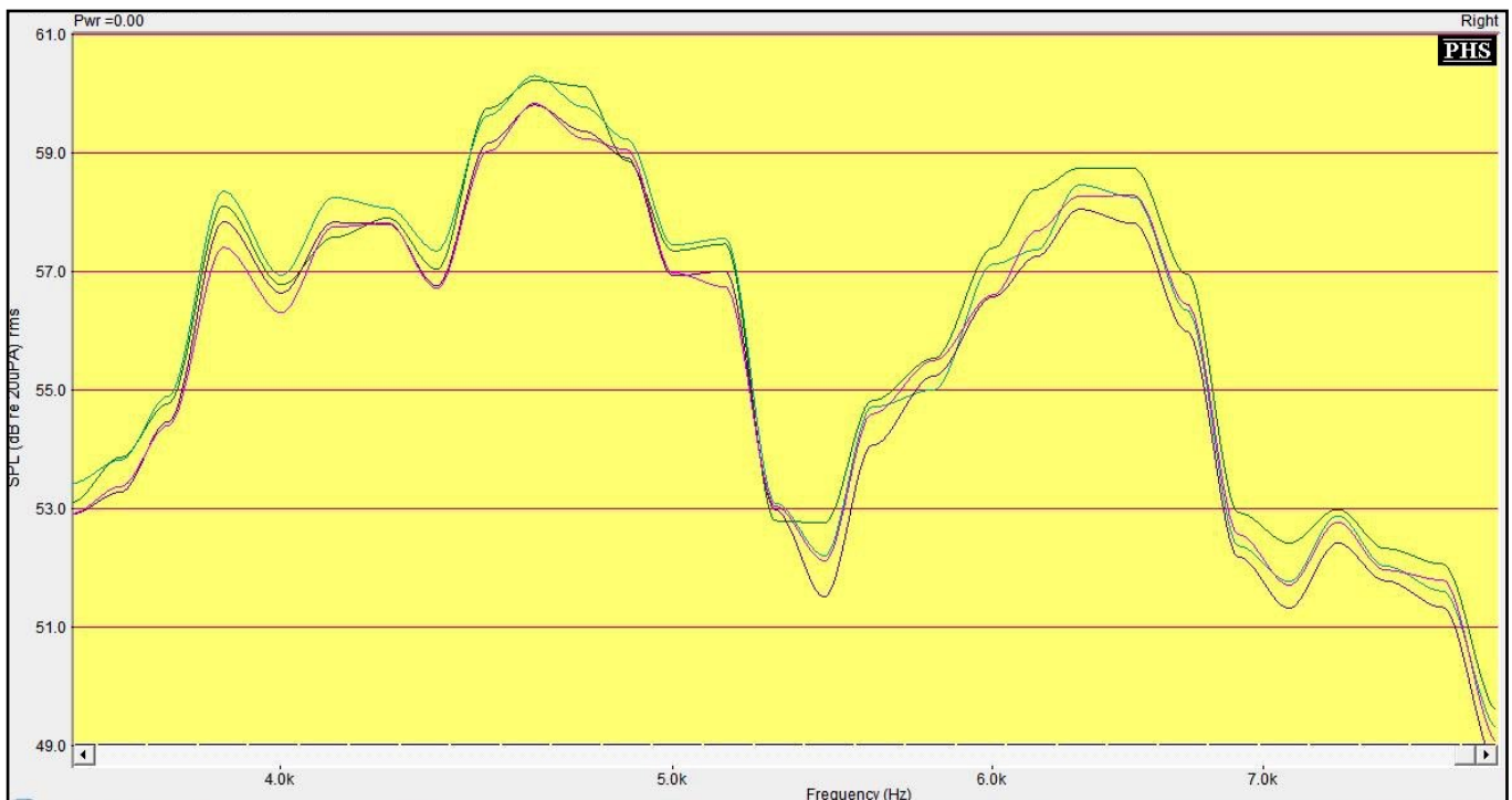
Figure n°169 : Zoom de 4000 à 8000 Hz, des spectres du bruit blanc obtenus avec les programmes P1 (vert), en P2 (bleu), en P3 (violet) et en P4 (rose)
