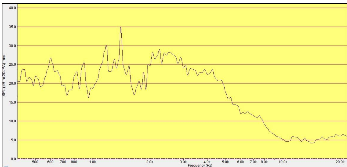
Figure n°50 : Spectre du bruit de rame de métro émis à 55 dB, obtenu à travers « l'oreille nue » de la tête artificielle du KEMAR
