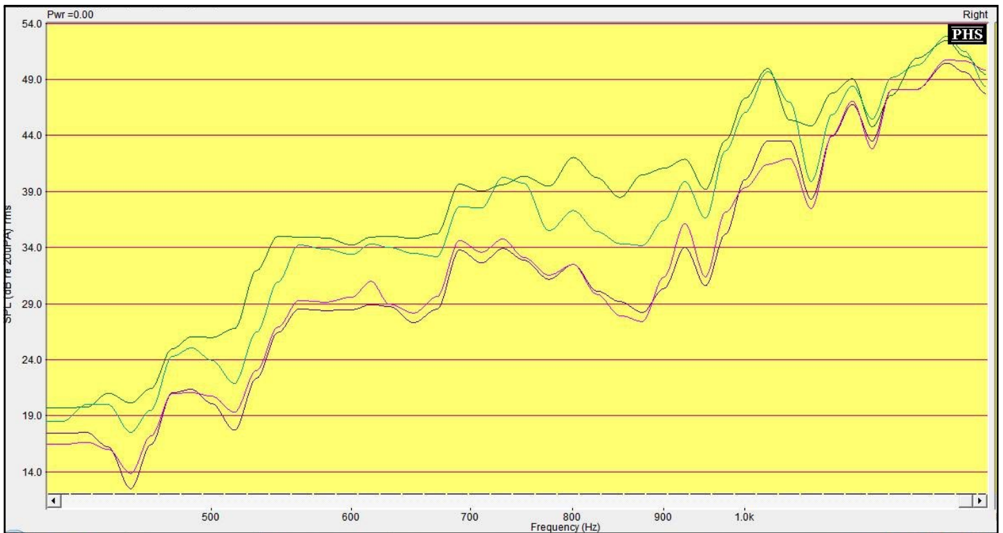
Figure n°63 : Zoom de 400 à 1500 Hz, des spectres du bruit de cris d'enfants obtenus avec les programmes P1 (vert), en P2 (bleu), en P3 (violet) et en P4 (rose)
