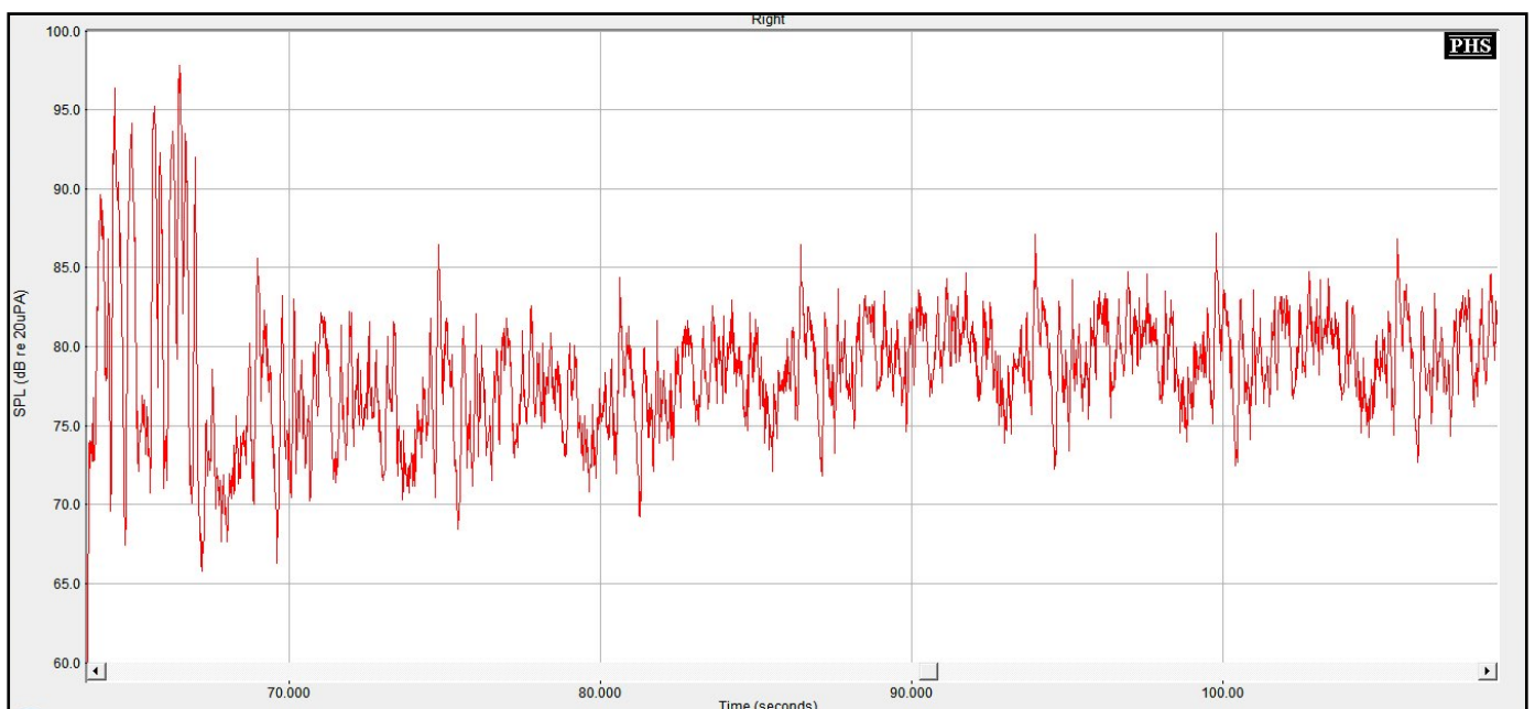
Figure n°303 : Zoom de la représentation temporelle du bruit de salle de jeux d'enfants émis à 55 dB et d'un signal de parole de 15 s à voix forte, provenant tous deux de l'azimut 0°, obtenu avec le programme P1, Dual et Ck dégressifs, Réducteur de bruit réglé par bandes
