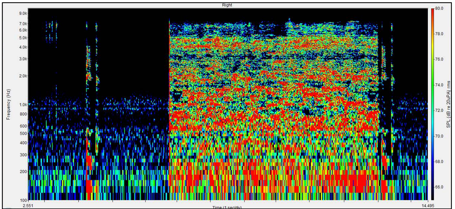
Figure n°196 : Spectrogramme du mot « pipe », 5 s de silence, puis 5 s de bruit de cris d'enfants puis 0,1 s de silence et de nouveau le mot « pipe » émis à 70 dB à l'azimut 0°, avec un RSB de 0 dB, obtenu avec la compression Syllabic
