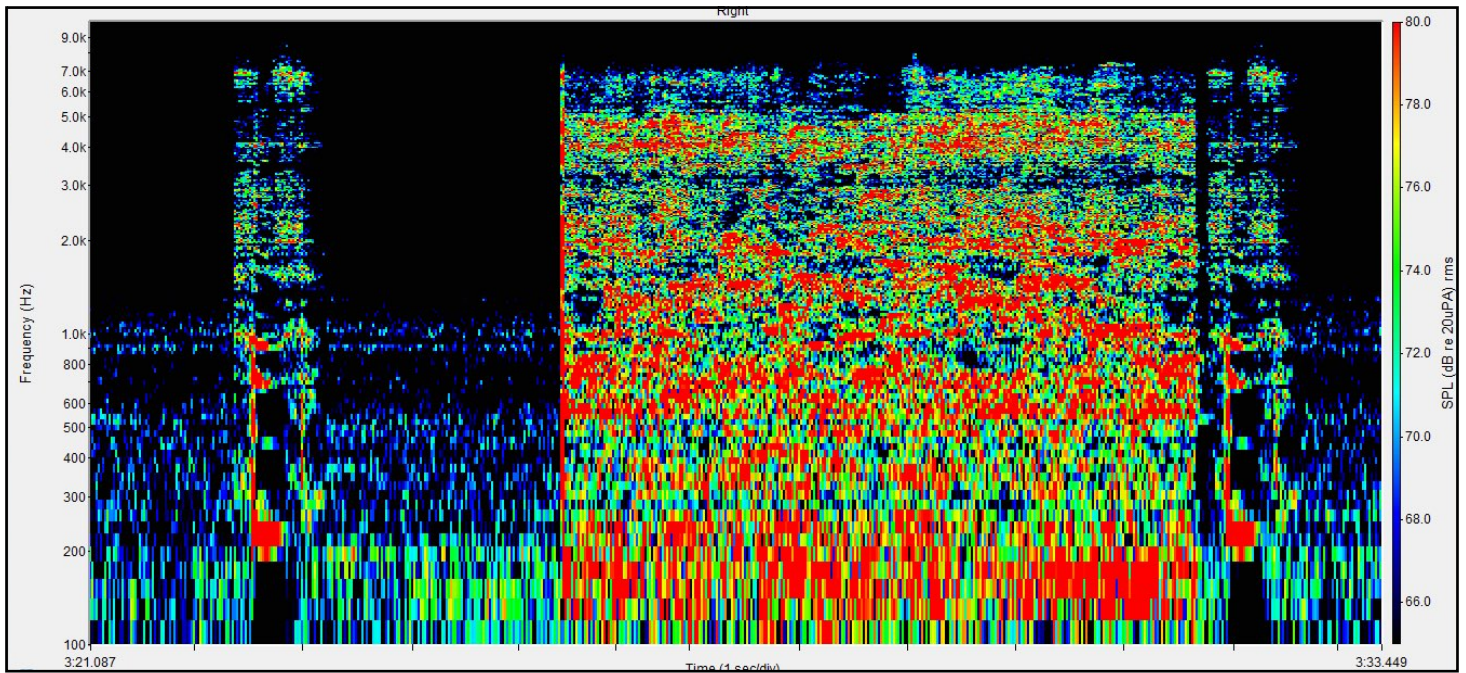
Figure n°223: Spectrogramme du logatome « faf », 5 s de silence, puis 5 s de bruit de cris d'enfants puis 0,1 s de silence et de nouveau le logatome « faf » émis à 70 dB à l'azimut 0°, avec un RSB de 0 dB, obtenu avec la compression Syllabic
