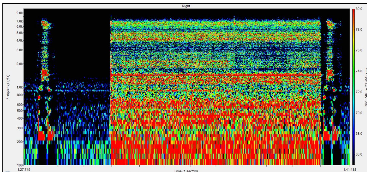
Figure n°274 : Spectrogramme du logatome « ouchou » 5 s de silence, puis 5 s de bruit de rame de métro puis 0,1 s de silence et de nouveau le logatome « ouchou » émis à 70 dB à l'azimut 0°, avec un RSB de 0 dB, obtenu avec la compression Syllabic
