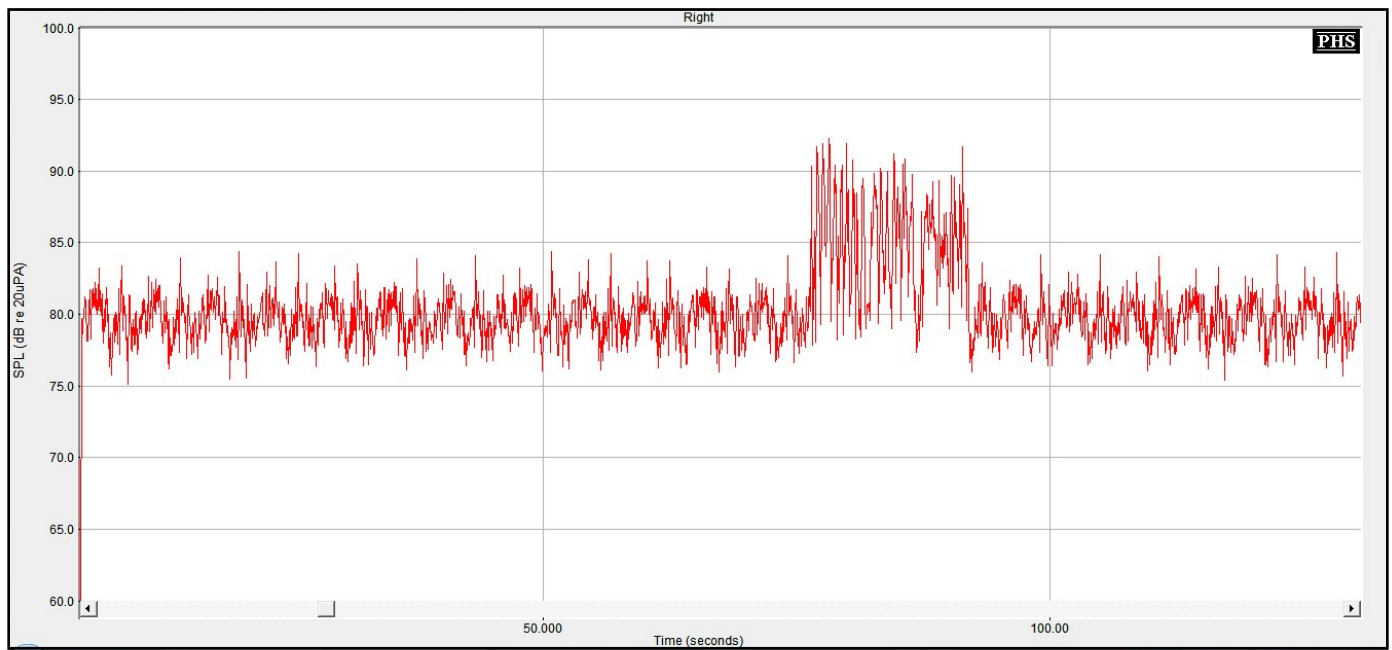
Figure n°326 : Représentation temporelle du bruit de salle de jeux d'enfants émis à 55 dB et d'un signal de parole de 15 s à voix forte, provenant tous deux de l'azimut 0°, obtenue avec le programme P4, Syllabic et Ck dégressifs, Réducteur de bruit réglé désactivé
