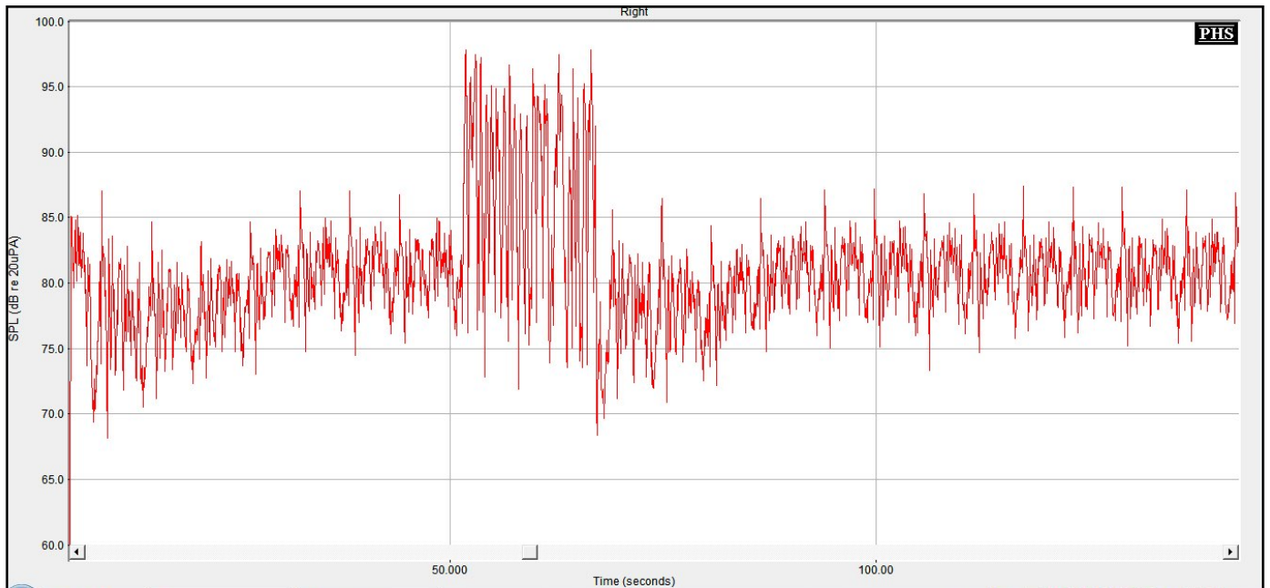
Figure n°302 : Représentation temporelle du bruit de salle de jeux d'enfants émis à 55 dB et d'un signal de parole de 15 s à voix forte, provenant tous deux de l'azimut 0°, obtenue avec le programme P1, Dual et Ck dégressifs, Réducteur de bruit réglé par bandes
