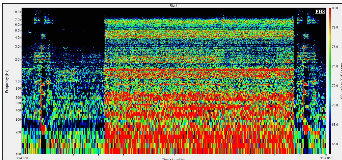
Figure n°286 : Spectrogramme du logatome « sasse » 5 s de silence, puis 5 s de bruit de rame de métro puis 0,1 s de silence et de nouveau le logatome « sasse » émis à 70 dB à l'azimut 0°, avec un RSB de 0 dB, obtenu avec la compression Syllabic
