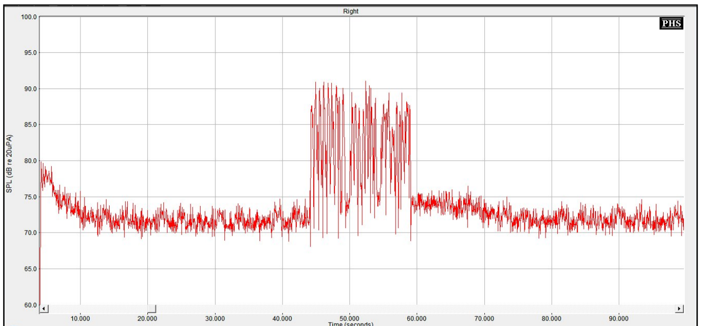
Figure n°103 : Représentation temporelle du bruit de rame de métro émis à 55 dB et d'un signal de parole de 15 s à voix forte, provenant tous deux de l'azimut 0°, obtenue avec le programme P3, Syllabic et Ck à 20 dB, Réducteur de bruit réglé au maximum
