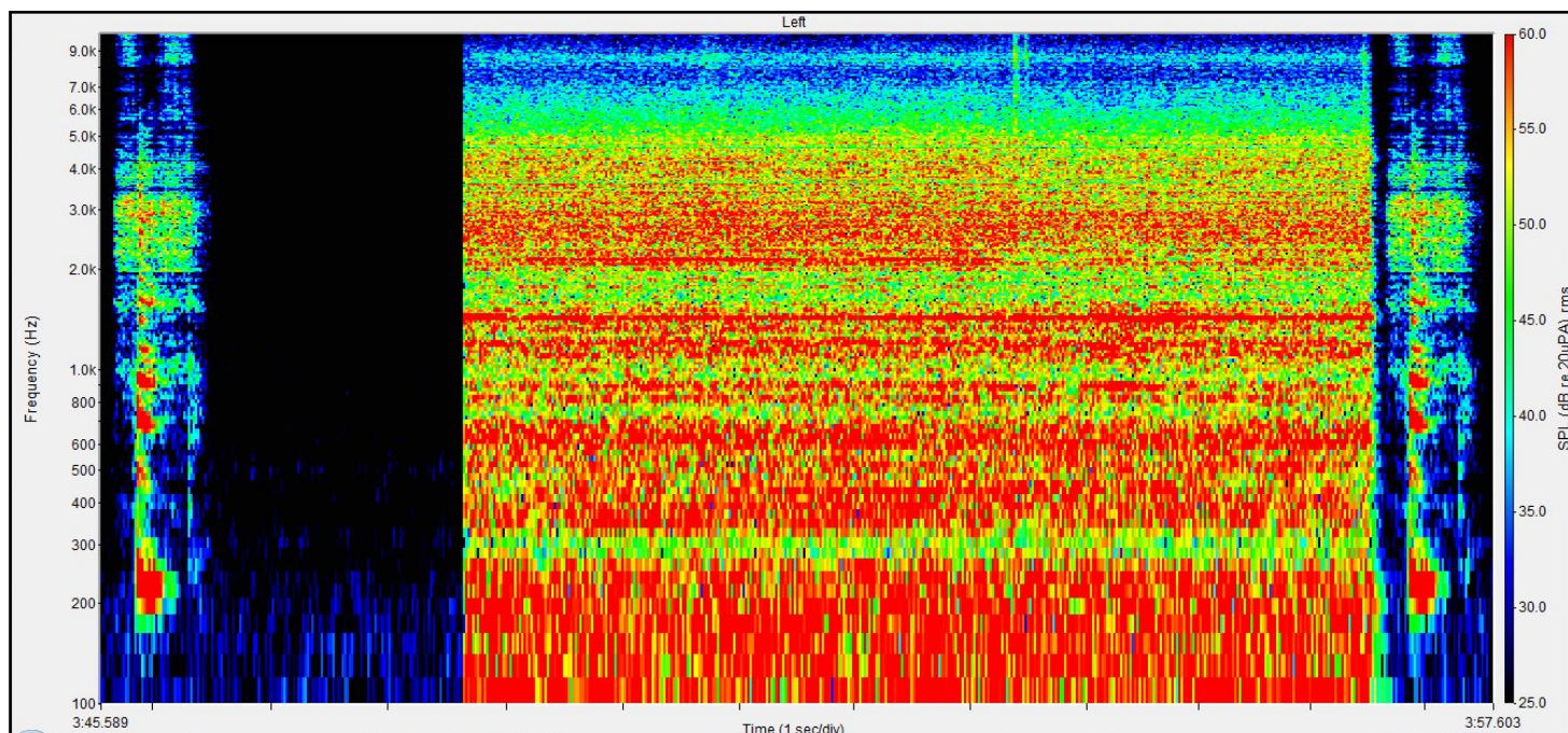
Figure n°288 : Spectrogramme du logatome « faf» 5 s de silence, puis 5 s de bruit de rame de métro puis 0,1 s de silence et de nouveau le logatome « fac » émis à 70 dB à l'azimut 0°, avec un RSB de 0 dB, obtenu oreille nue du KEMAR
