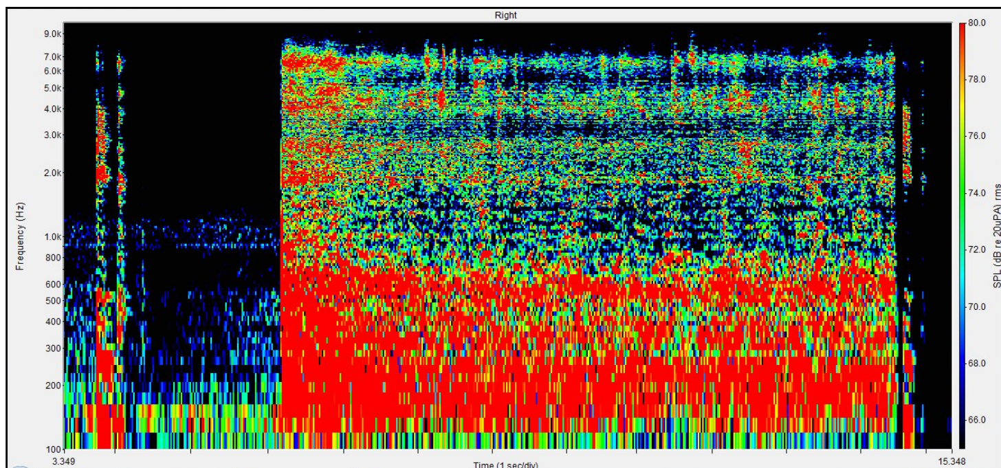
Figure n°230 : Spectrogramme du mot « pipe » 5 s de silence, puis 5 s de bruit de restaurant puis 0,1 s de silence et de nouveau le mot « pipe » émis à 70 dB à l'azimut 0°, avec un RSB de 0 dB, obtenu avec la compression Dual
