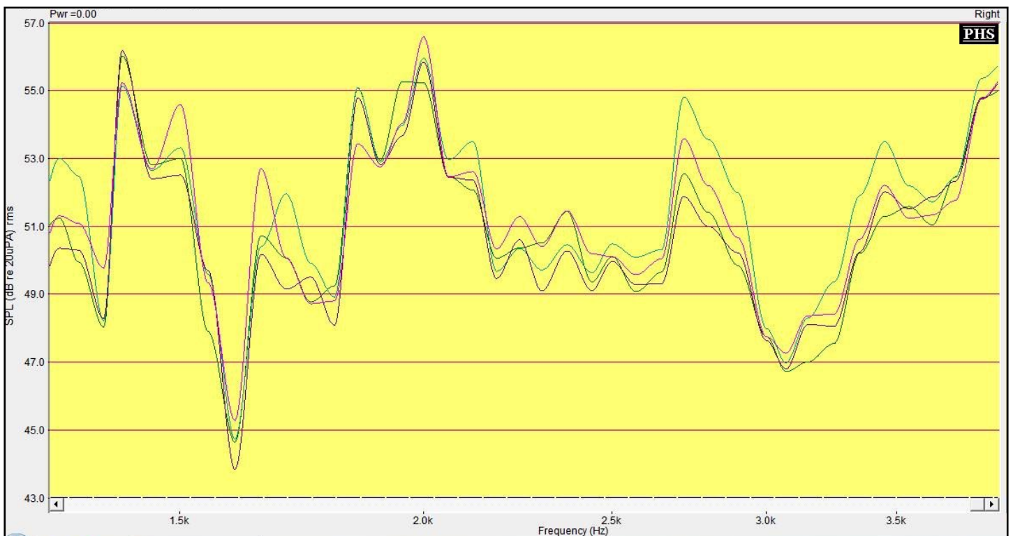
Figure n°64 : Zoom de 1500 à 4000 Hz, des spectres du bruit de cris d'enfants obtenus avec les programmes P1 (vert), en P2 (bleu), en P3 (violet) et en P4 (rose)
