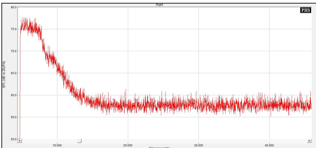
Figure n°151 : Représentation temporelle de l'action du réducteur de bruit réglé en bande large au maximum sur un bruit blanc émis à 55 dB SPL quand l'appareil possède un gain de 20 dB, un taux de compression de 1,5 et des Ck à 70 dB
