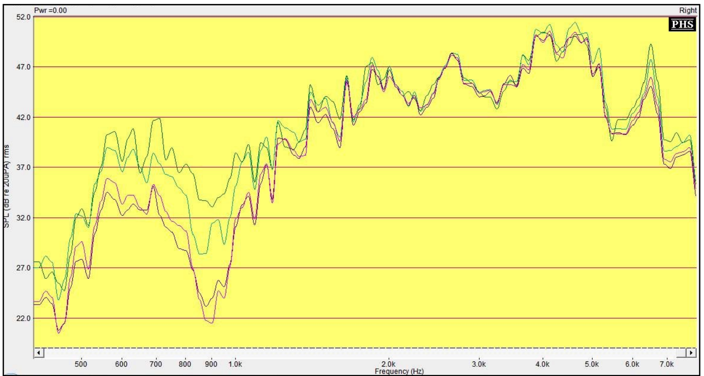
Figure n°59 : Spectres du bruit de restaurant obtenus avec les programmes P1 (vert), en P2 (bleu), en P3 (violet) et en P4 (rose)
