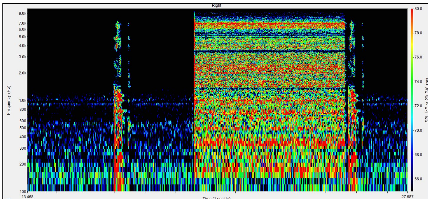
Figure n°175 : Spectrogramme du mot « râpe », 5 s de silence, puis 5 s de bruit blanc puis 0,1 s de silence et de nouveau le mot « râpe » émis à 70 dB à l'azimut 0°, avec un RSB de 0 dB, obtenu avec la compression Syllabic
