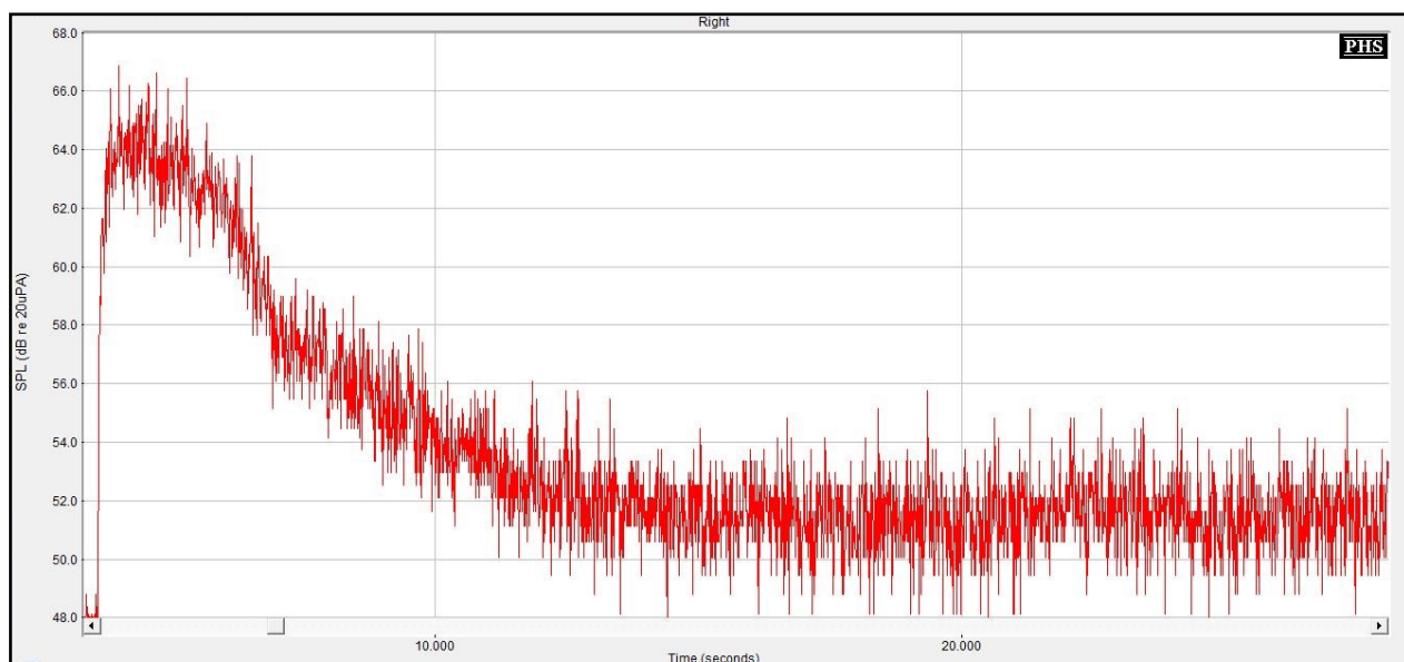
Figure n°35 : Représentation temporelle de l'action du réducteur de bruit réglé en bande large au maximum sur un bruit blanc, émis à 40 dB SPL
