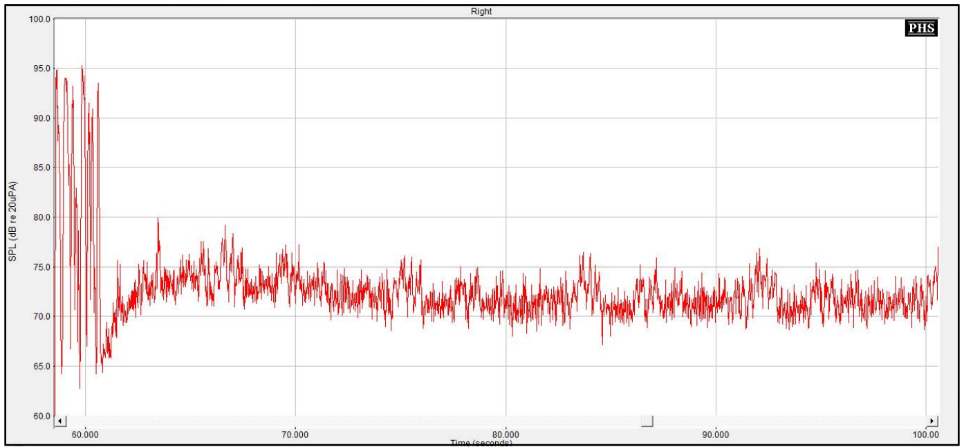
Figure n°102 : Zoom de la représentation temporelle du bruit de rame de métro émis à 55 dB et d'un signal de parole de 15 s à voix forte, provenant tous deux de l'azimut 0°, obtenu avec le programme P2, Dual et Ck à 20 dB, Réducteur de bruit réglé au maximum
