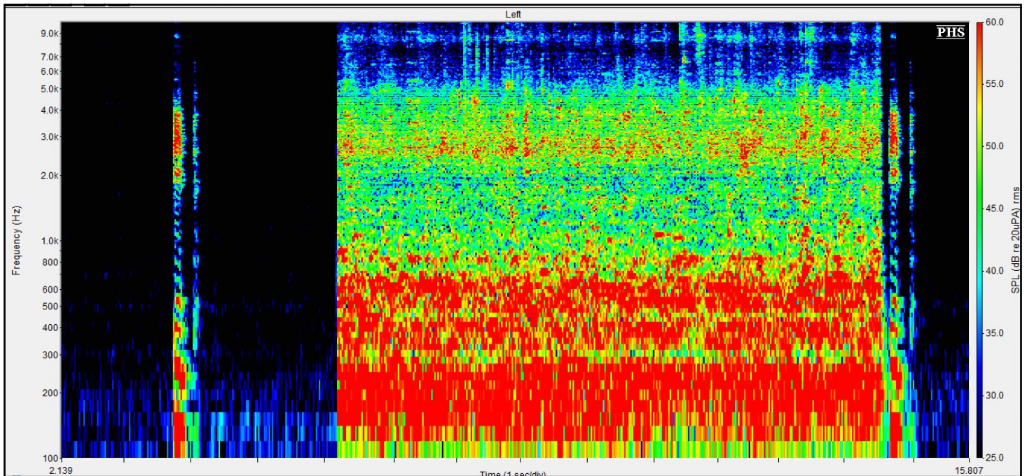
Figure n°228 : Spectrogramme du mot « pipe » 5 s de silence, puis 5 s de bruit de restaurant puis 0,1 s de silence et de nouveau le mot « pipe » émis à 70 dB à l'azimut 0°, avec un RSB de 0 dB, obtenu oreille nue du KEMAR
