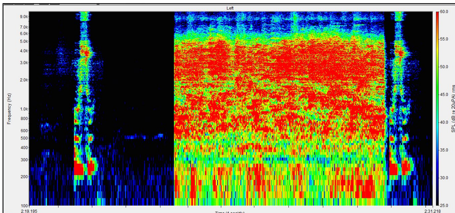
Figure n°213 : Spectrogramme du logatome « oussou », 5 s de silence, puis 5 s de bruit de cris d'enfants puis 0,1 s de silence et de nouveau le logatome « oussou » émis à 70 dB à l'azimut 0°, avec un RSB de 0 dB, obtenu oreille nue du KEMAR
