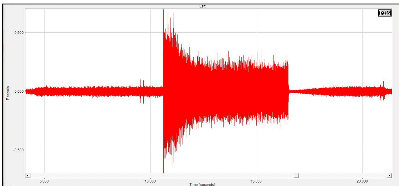
Figure n°165 : Représentation temporelle d'un bruit blanc émis de façon continue à 30, 60 puis 30 dB SPL, obtenue avec l'appareil réglé en Dual avec des seuils d'enclenchement à 20 dB, P2 du 2nd jeu de programmes
