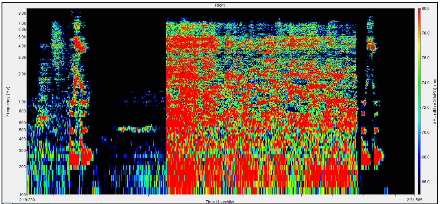
Figure n°215 : Spectrogramme du logatome « oussou », 5 s de silence, puis 5 s de bruit de cris d'enfants puis 0,1 s de silence et de nouveau le logatome « oussou » émis à 70 dB à l'azimut 0°, avec un RSB de 0 dB, obtenu avec la compression Dual
