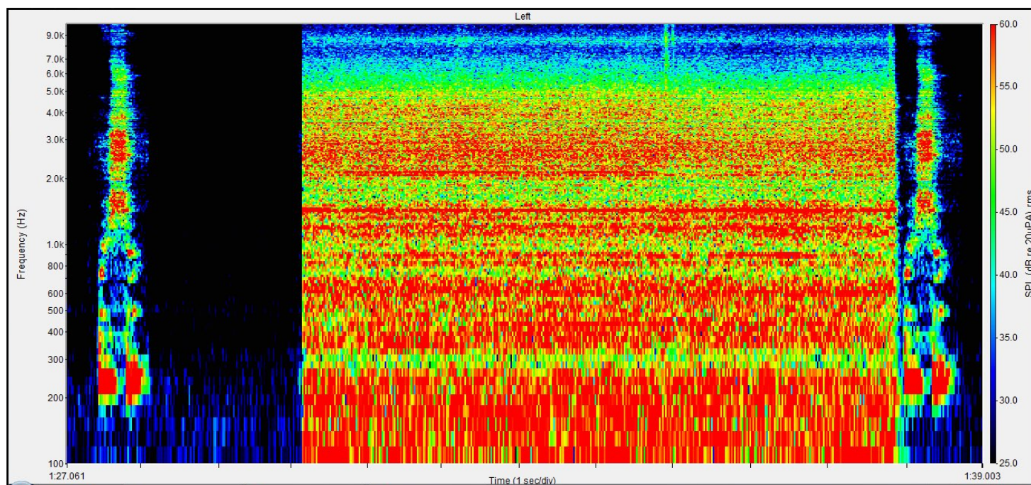
Figure n°273 : Spectrogramme du logatome « ouchou » 5 s de silence, puis 5 s de bruit de rame de métro puis 0,1 s de silence et de nouveau le logatome « ouchou » émis à 70 dB à l'azimut 0°, avec un RSB de 0 dB, obtenu oreille nue du KEMAR
