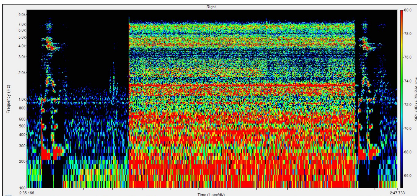
Figure n°280 : Spectrogramme du logatome « oussou » 5 s de silence, puis 5 s de bruit de rame de métro puis 0,1 s de silence et de nouveau le logatome « oussou » émis à 70 dB à l'azimut 0°, avec un RSB de 0 dB, obtenu avec la compression Syllabic
