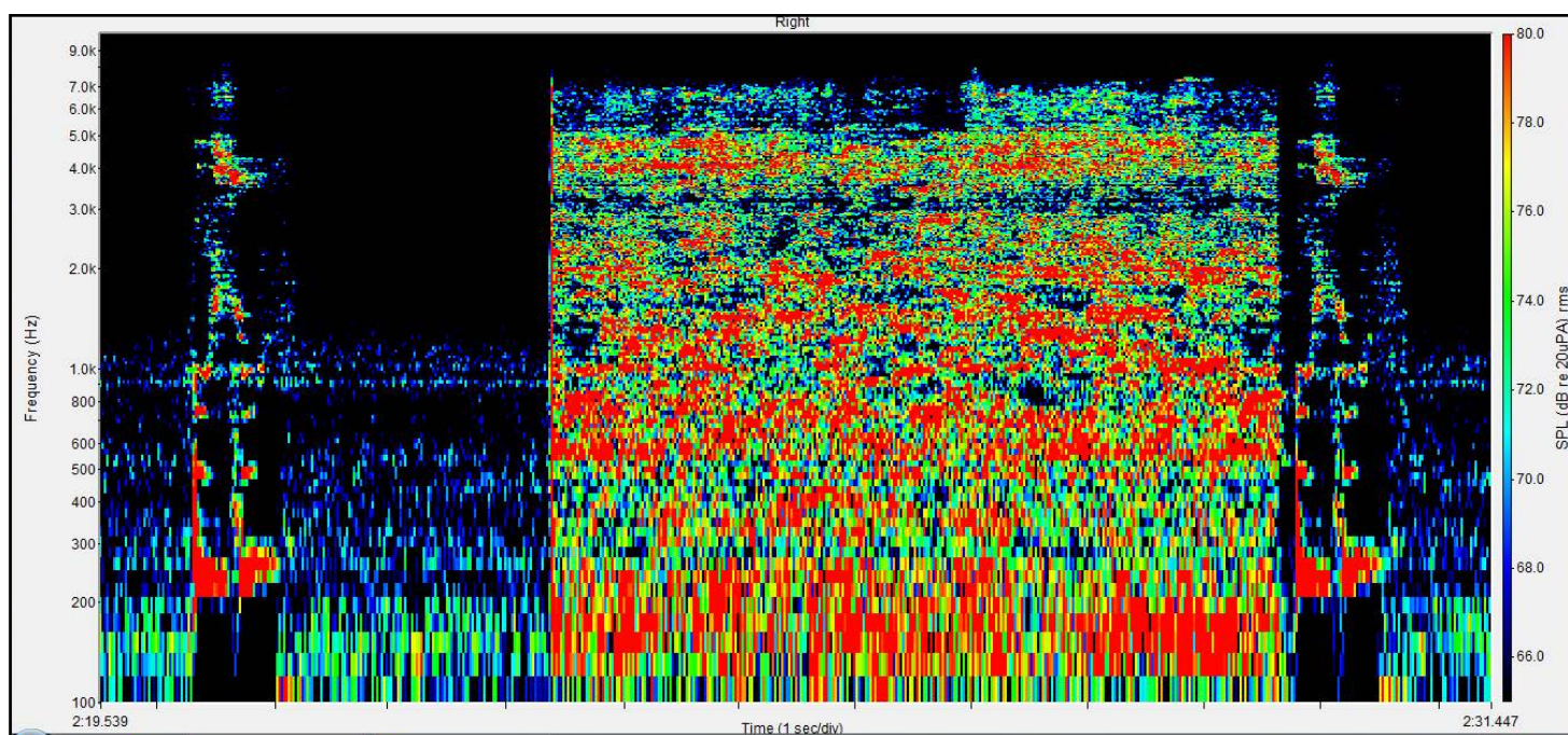
Figure n°214 : Spectrogramme du logatome « oussou », 5 s de silence, puis 5 s de bruit de cris d'enfants puis 0,1 s de silence et de nouveau le logatome « oussou » émis à 70 dB à l'azimut 0°, avec un RSB de 0 dB, obtenu avec la compression Syllabic
