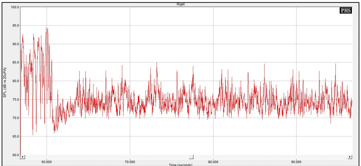
Figure n°311 : Zoom de la représentation temporelle du bruit de restaurant émis à 55 dB et d'un signal de parole de 15 s à voix forte, provenant tous deux de l'azimut 0°, obtenu avec le programme P1, Dual et Ck dégressifs, Réducteur de bruit réglé au maximum
