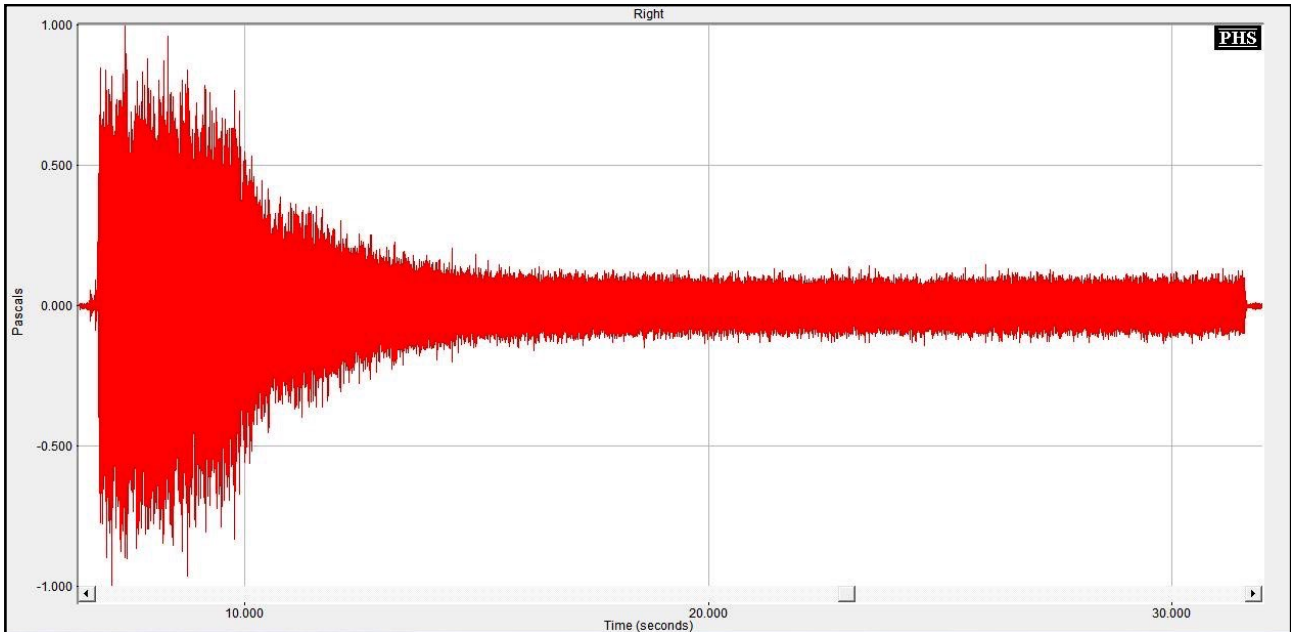
Figure n°122 : Représentation temporelle de l'action du réducteur de bruit réglé en bande large au maximum sur le bruit blanc
