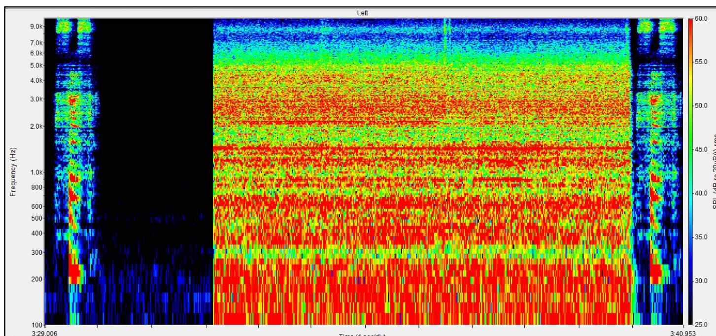
Figure n°285 : Spectrogramme du logatome « sasse » 5 s de silence, puis 5 s de bruit de rame de métro puis 0,1 s de silence et de nouveau le logatome « sasse » émis à 70 dB à l'azimut 0°, avec un RSB de 0 dB, obtenu oreille nue du KEMAR
