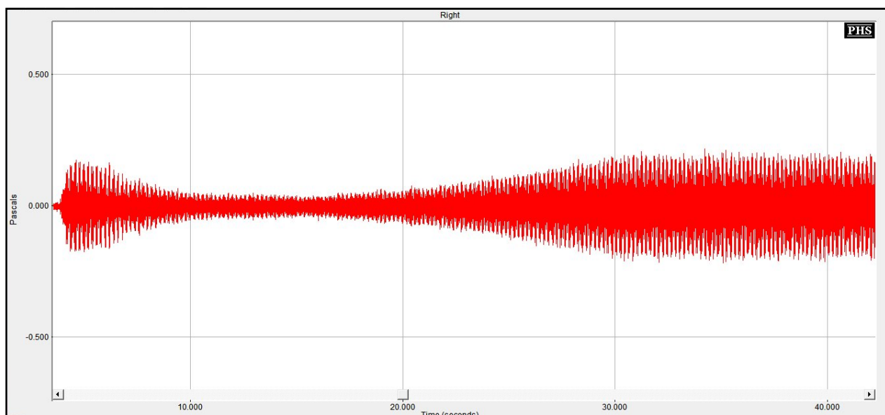
Figure n°128 : Représentation temporelle de l'action du réducteur de bruit réglé en bande large au maximum sur un son wobulé de 500 Hz, émis à 50 dB SPL
