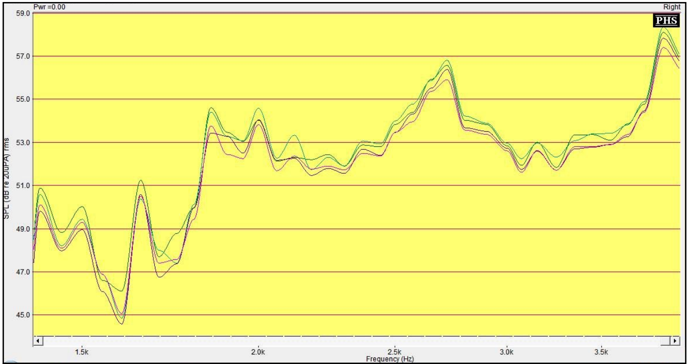
Figure n°168 : Zoom de 1500 à 4000 Hz, des spectres du bruit blanc obtenus avec les programmes P1 (vert), en P2 (bleu), en P3 (violet) et en P4 (rose)
