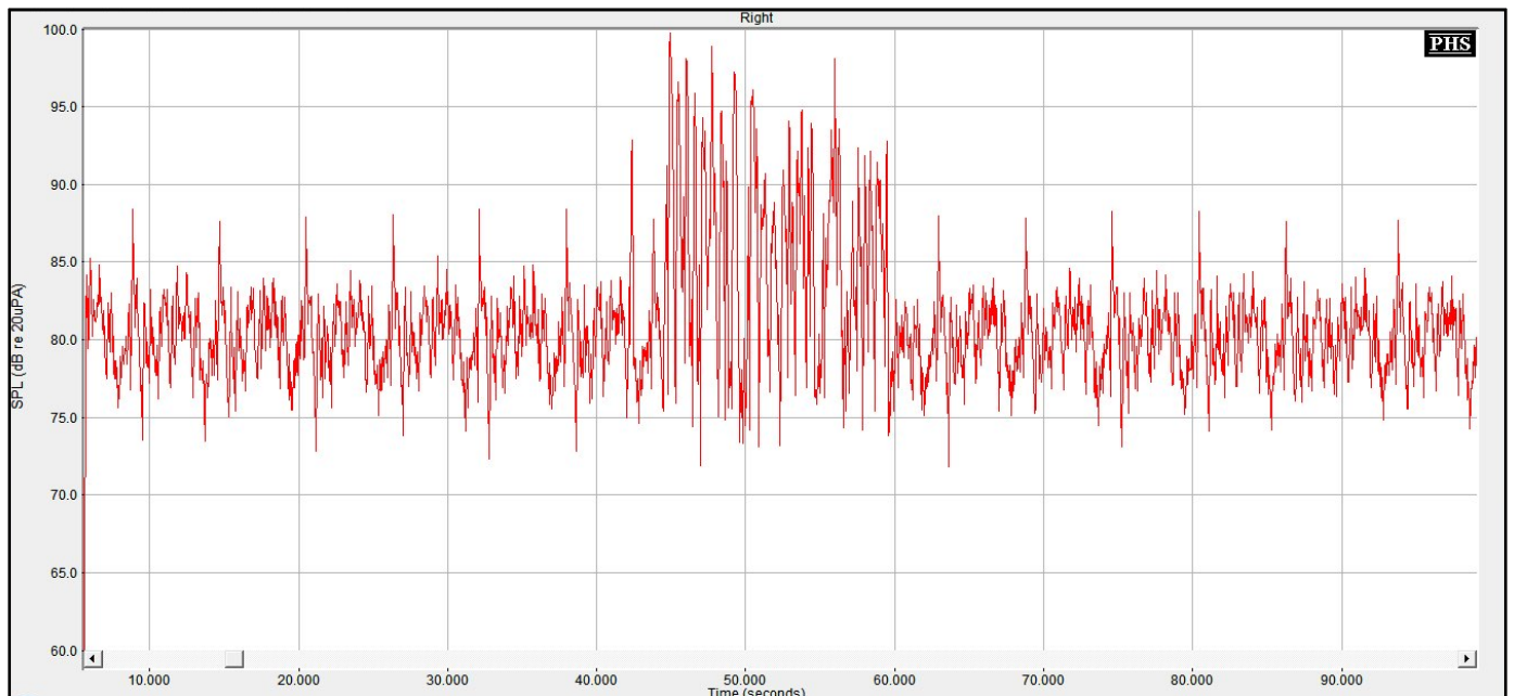
Figure n°324 : Représentation temporelle du bruit de salle de jeux d'enfants émis à 55 dB et d'un signal de parole de 15 s à voix forte, provenant tous deux de l'azimut 0°, obtenue avec le programme P1, Dual et Ck dégressifs, Réducteur de bruit réglé désactivé
