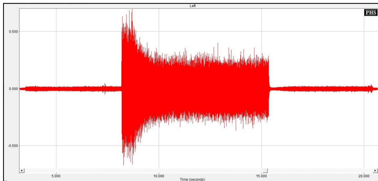
Figure n°164 : Représentation temporelle d'un bruit blanc émis de façon continue à 30, 60 puis 30 dB SPL, obtenue avec l'appareil réglé en Dual avec des seuils d'enclenchement dégressifs, P1 du 2nd jeu de programmes
