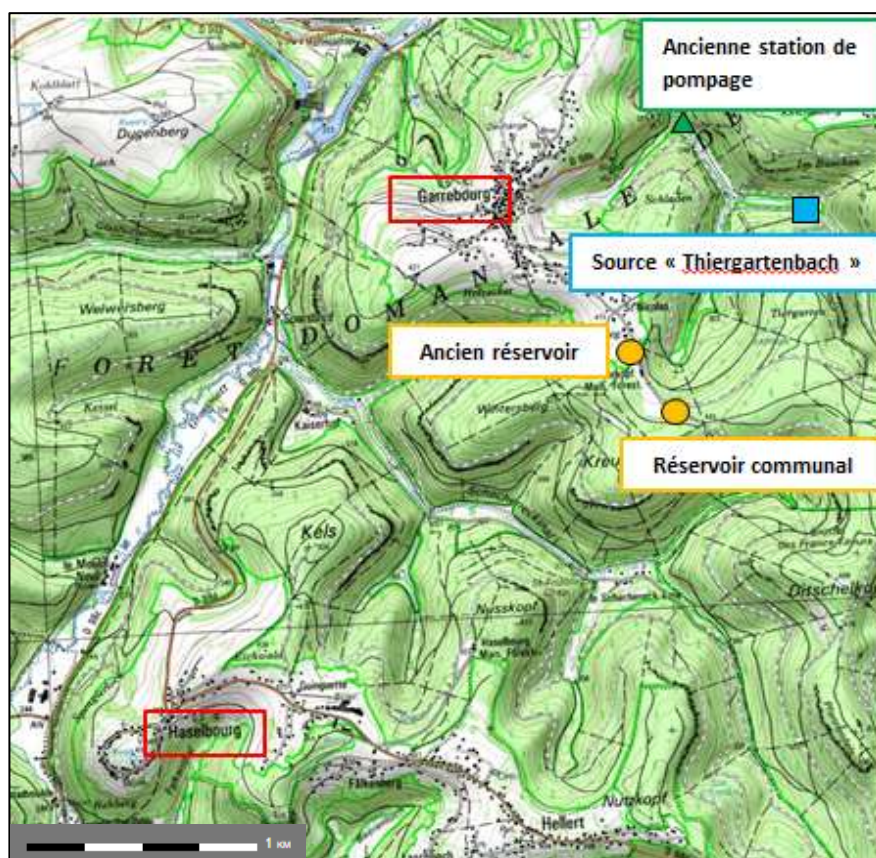
Figure 4 Localisation des ouvrages du système AEP de la commune de Garrebourg (échelle 1/25 000)
