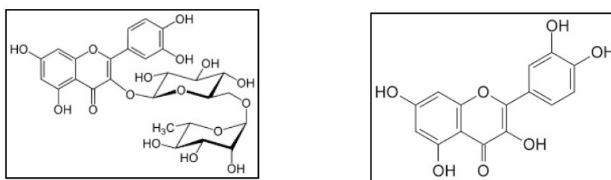
Figure 4: Structure chimique de deux flavonols : a) Structure chimique de la rutine ; b) Structure chimique de la quercetine (Vikas, 2011).
