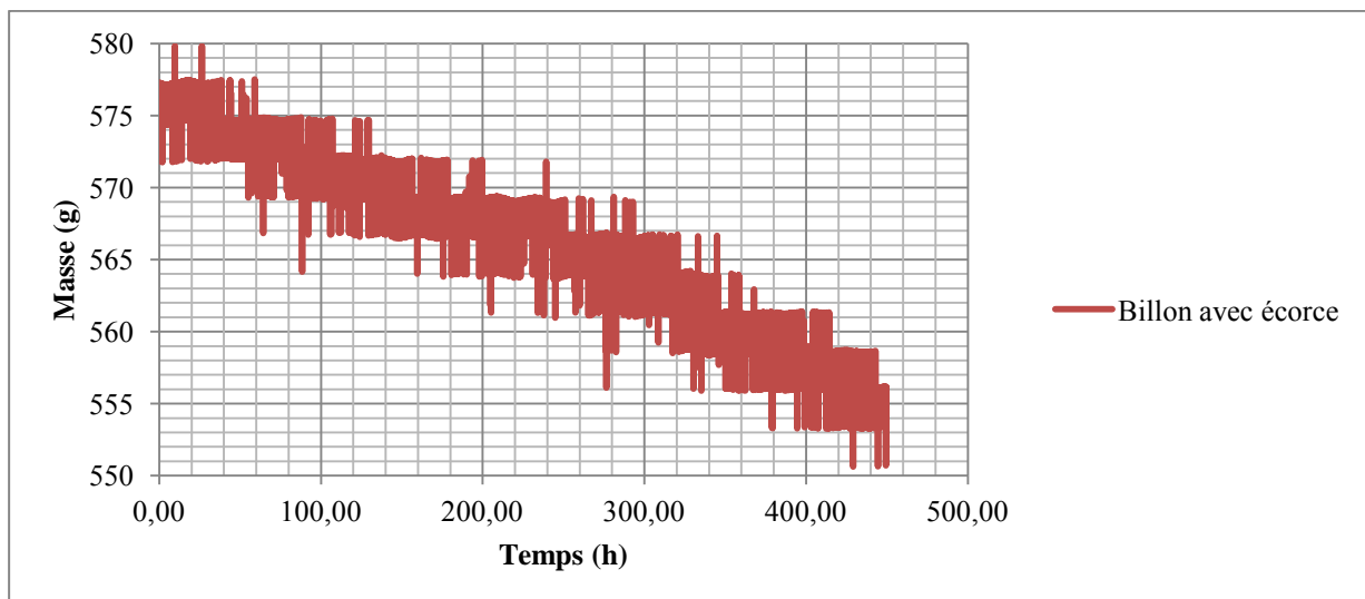
Figure 24 : variation de la masse du billon d'épicéa avec écorce en fonction du temps pendant la première expérience
