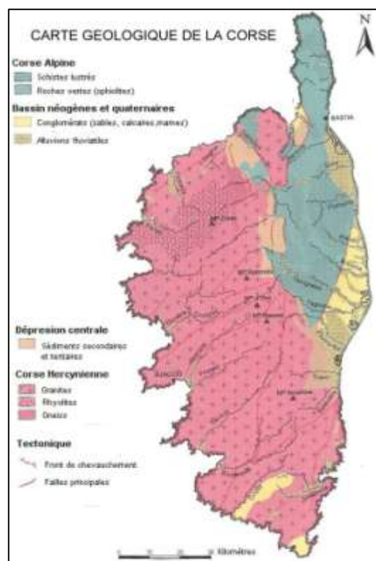
Figure 3 – Carte géologique de la Corse (Source : cartograf.fr/regions/corse.php )
