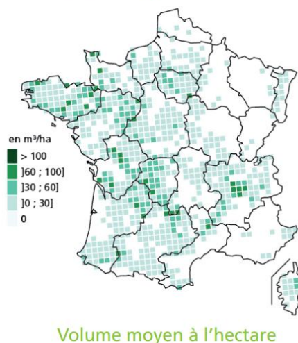
Figure 2 : aire de répartition du châtaignier en France (source IFN : 2011)
