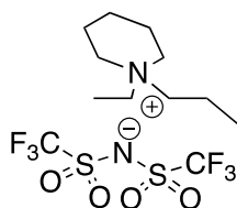
Figure 6. Liquide ionique bis(trifluorométhylsulfonyl)imide de 1-butyl-1-éthylpipéridinium (BEPipNTf 2 )
