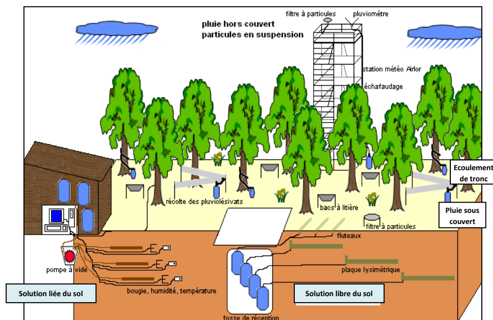
Figure 5 - Schématisation du dispositif expérimental des stations du site de Montiers.
