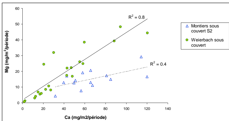
Figure 7 – Corrélation entre les flux de Ca et Mg dans les pluviolessivats à Montiers (station S2) et au Weierbach.
