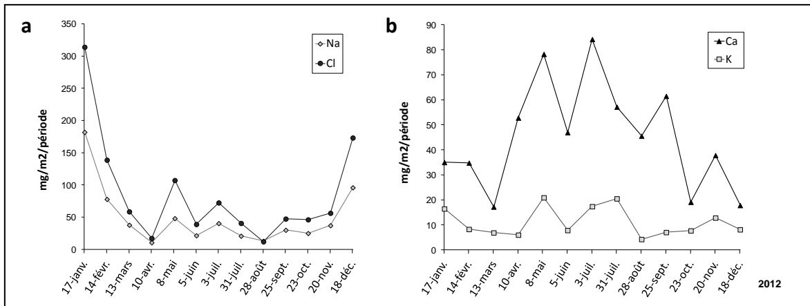
Figure 9 – Evolution temporelle des dépôts humides de Na et Cl (a) et de Ca et K (b) au cours de l'année 2012.
