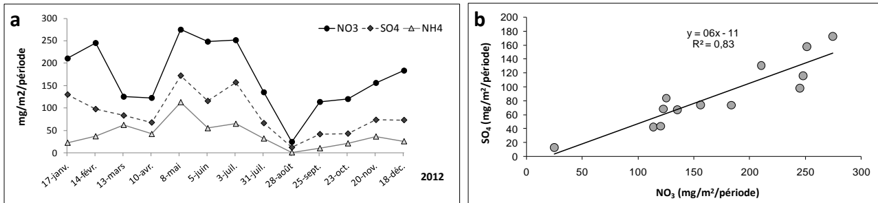
Figure 10 – Evolution temporelle des dépôts humides de \text{SO}_4 , \text{NO}_3 , et \text{NH}_4 (a) et corrélation entre les apports de \text{NO}_3 et \text{SO}_4 (b).
