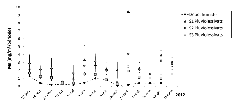
Figure 15 - Flux mensuels de Mn hors couvert (dépôt humide) et sous couvert (pluiolessivats des trois stations).
