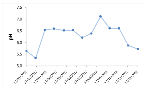
Figure 8 – Evolution temporelle du pH des dépôts humides à Montiers (janvier 2012 – décembre 2012).
