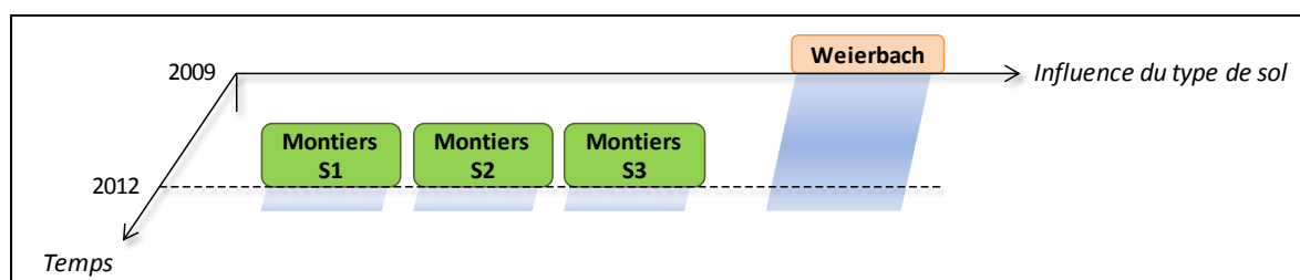
Figure 2 – Principe de l'étude comparative dans le cadre du projet LORLUX.
