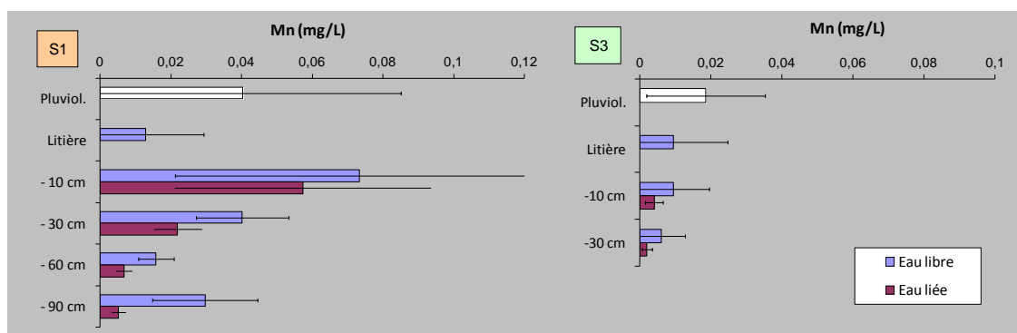
Figure 22 - Moyennes annuelles (2012) des teneurs en Mn dans les pluviolésivats (en blanc), l'eau des litières et les solutions liées et libres prélevées à différentes profondeurs du sol dans les stations S1 et S3.
