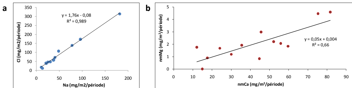
Figure 11 – Corrélation entre les dépôts humides de Na et Cl (a) et des parts non marines de Ca et Mg (b).
