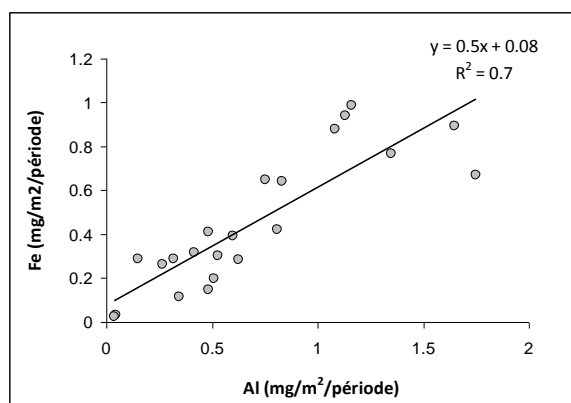
Figure 6 – Corrélation entre les flux de Fe et Al dans les pluviolessivats de la placette expérimentale du Weierbach.
