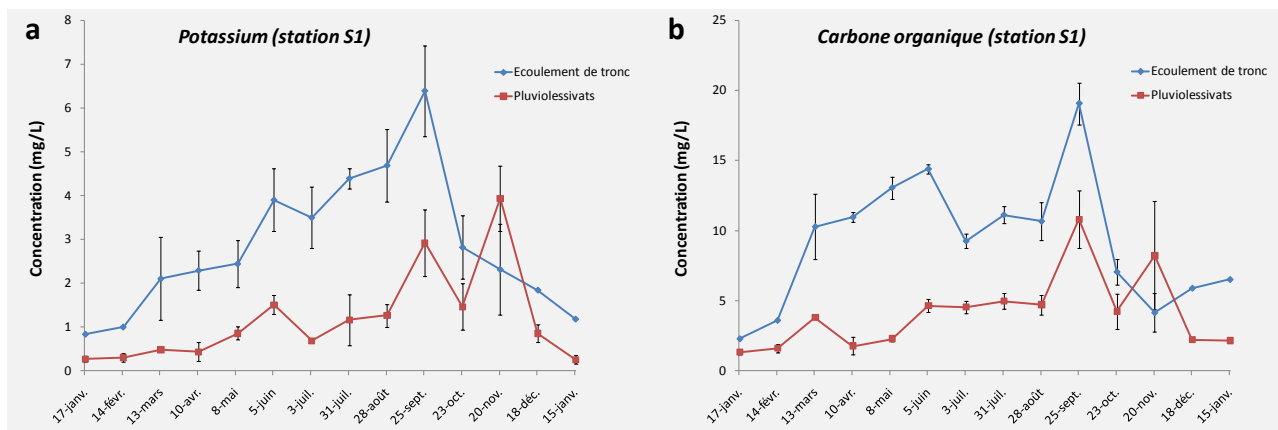
Figure 17 – Comparaison des teneurs en K (a) et COD (b) dans les pluviolessivats et les écoulements de tronc de la station S1 de janvier 2012 à janvier 2013.
