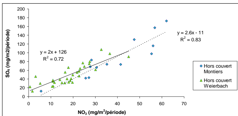
Figure 2 – Corrélations entre les flux de SO 4 et NO 3 dans les dépôts humides à Montiers (Fr.) et au Weierbach (Lux.).
