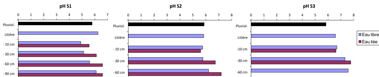
Figure 18 – Moyennes annuelles (2012) des valeurs de pH des pluviolessivats (en noir), de l'eau des litières et des solutions liées et libres prélevées à différentes profondeurs du sol dans les trois stations.
