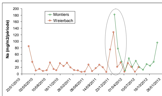
Figure 3 – Evolution temporelle des flux de sodium dans les dépôts humides à Montiers (Fr.) et au Weierbach (Lux.).
