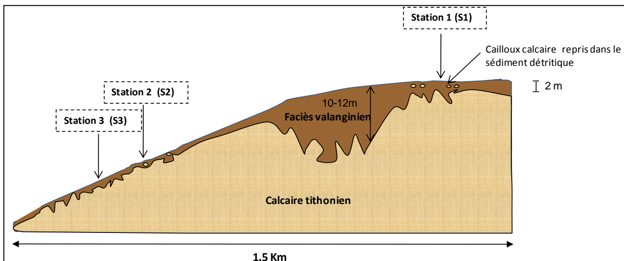
Figure 4 – Représentation schématique de la coupe géologique de la toposéquence de Montiers.
