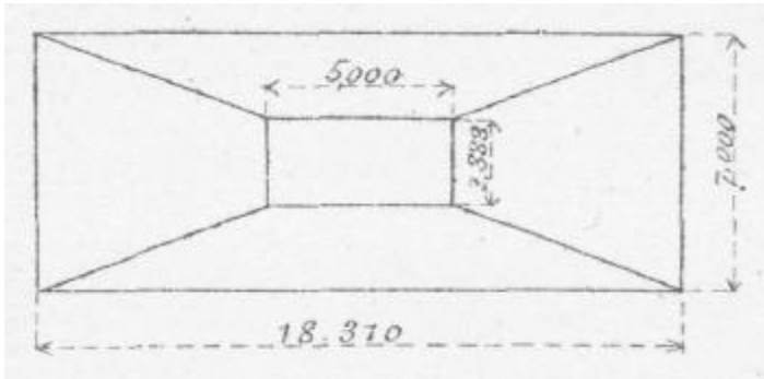
Figure 14 : vue de dessus d'une pile
