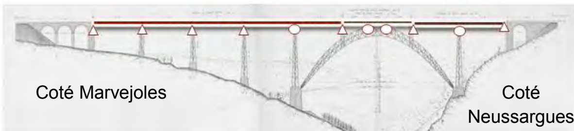
Figure 10 : Explication des tabliers
