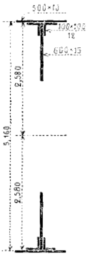
Figure 16 : profil d'une poutre du tablier
