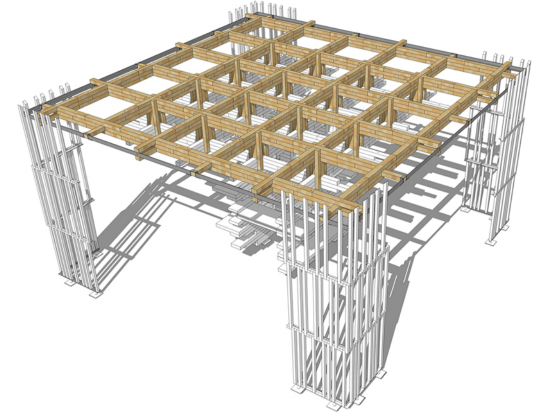
INSTALLATION DE LA TROISIEME NAPPE
