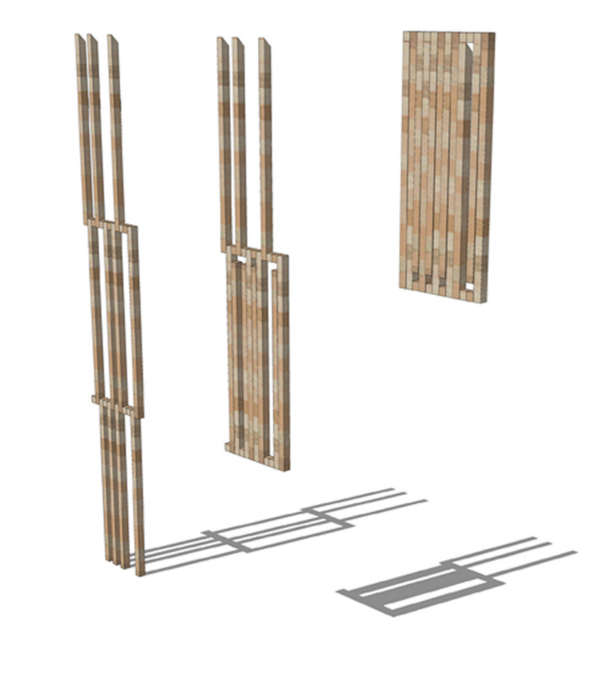
CROQUIS DE LA PEAU PLIABLE
