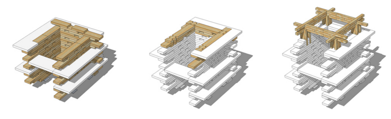
INSTALLATION DU NOYAU ET DE LA PREMIERE NAPPE
