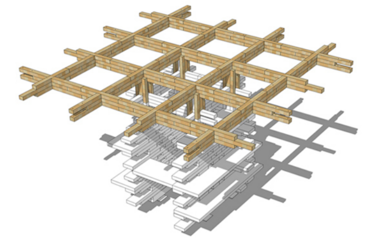
INSTALLATION DE LA DEUXIEME NAPPE
