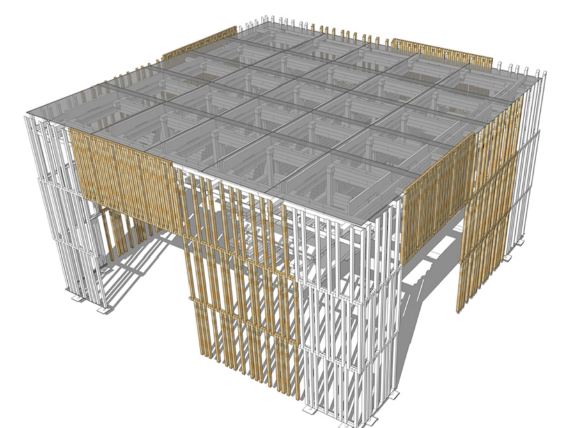
INSTALLATION DES RIDEAUX
