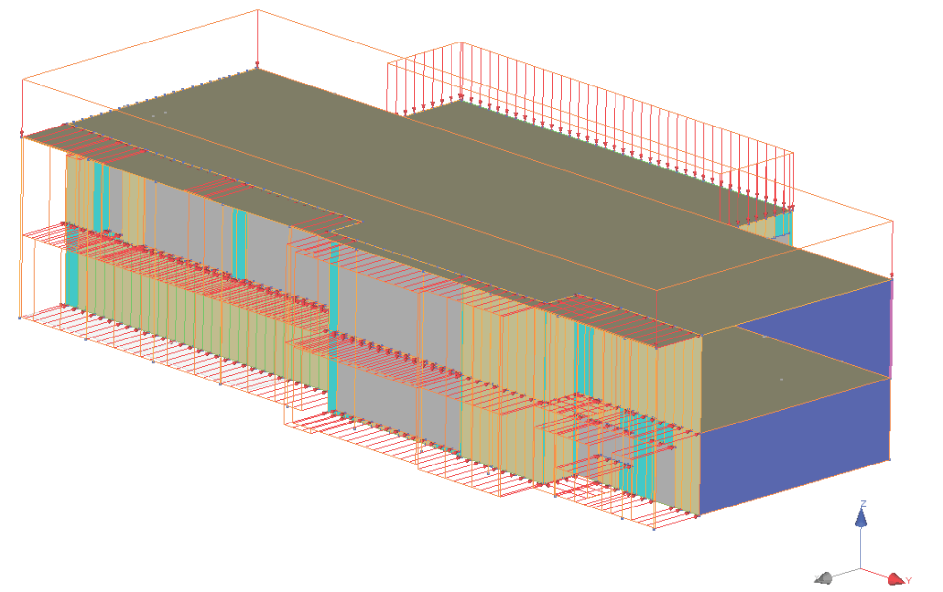
MODELE STRUCTUREL ET CHARGEMENTS / Axonométrie
