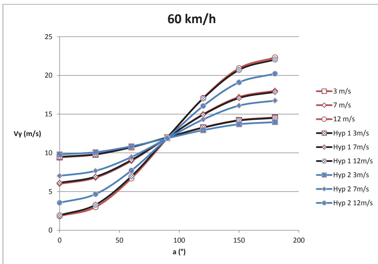
Figure 33c : V_y mesure à V_{véhicule} = 60 km/h
