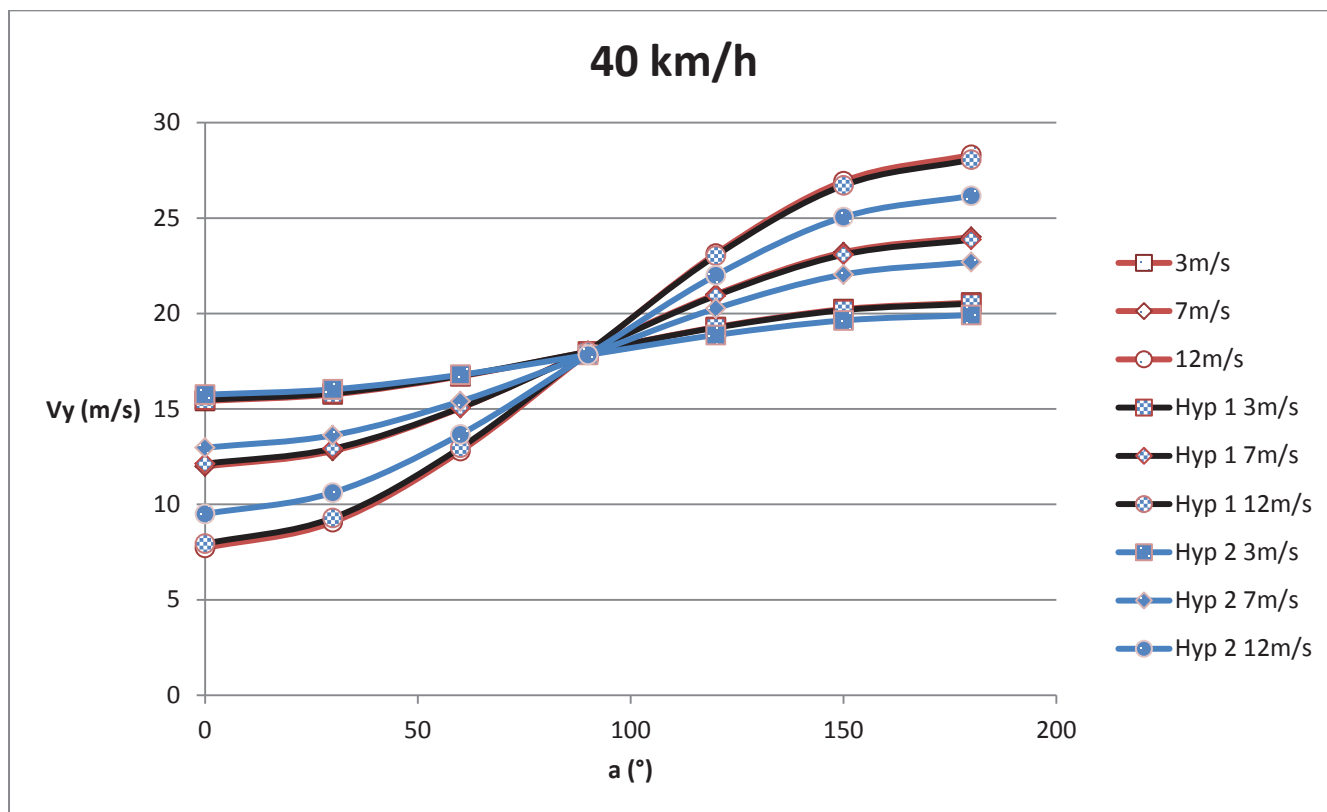
Figure 33b : V_y mesure à V_{véhicule} = 40 km/h
