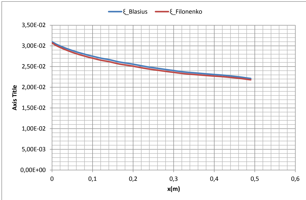
Figure IV-7 : variation du coefficient de frottement le long du tube
