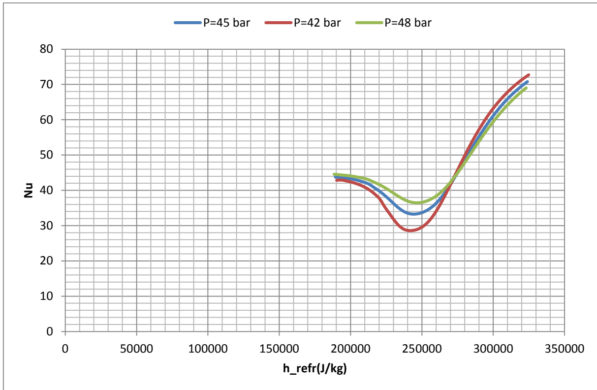
Figure III-5 : Evolution du nombre de NUSSELT avec la corrélation de KRASNOSHCHEKOV
