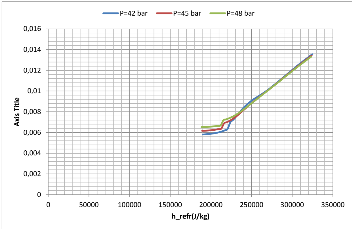
Figure III-13 : Evolution du coefficient de perte de pression avec la corrélation de POPOV
