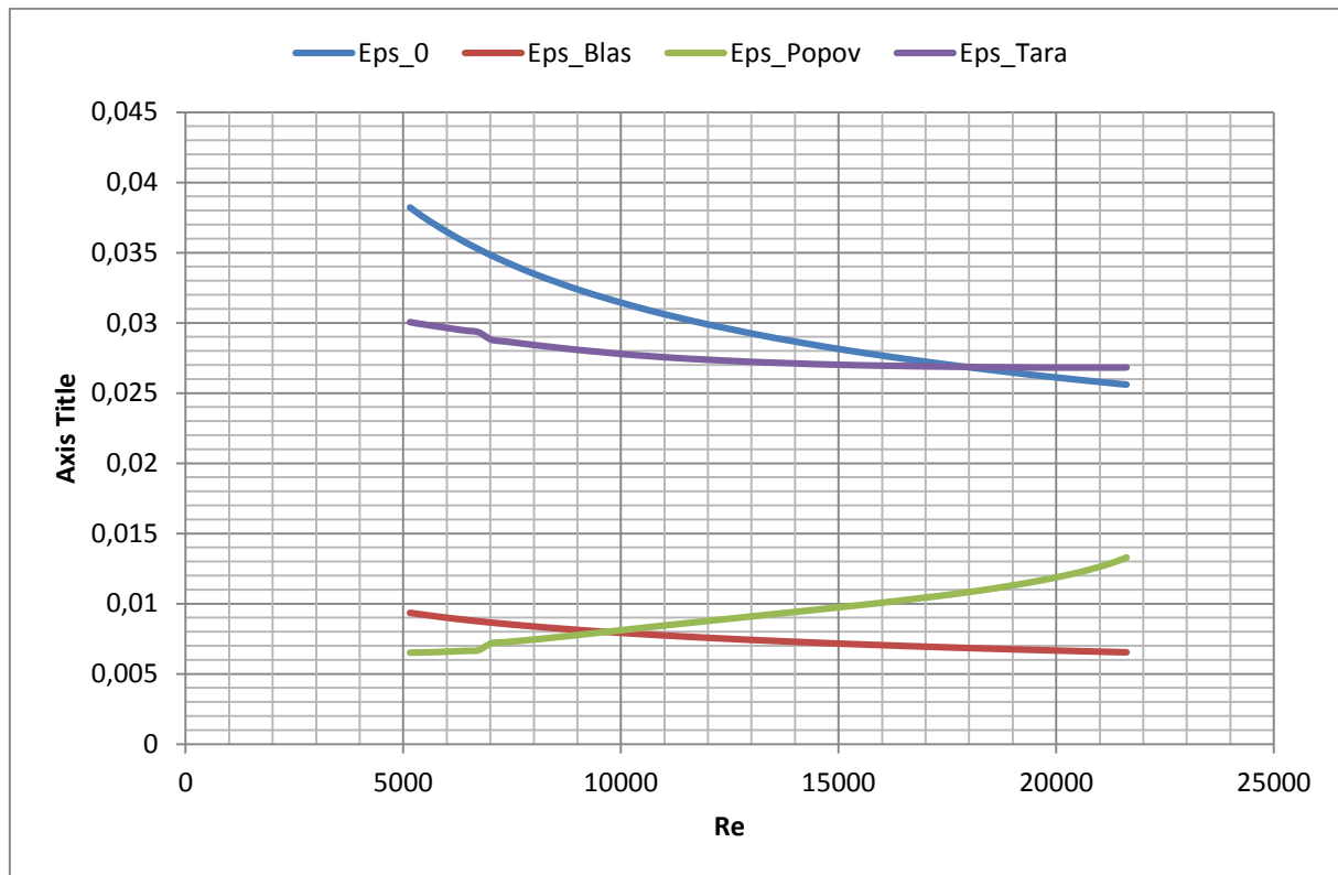
Figure III-15 : évolution des différents coefficients de pertes de pression en fonction du nombre de REYNOLDS
