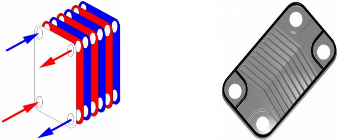
Figure VI-4: schéma d'un échangeur à plaques et une plaque avec profil Chevron (WIKIPEDIA)
