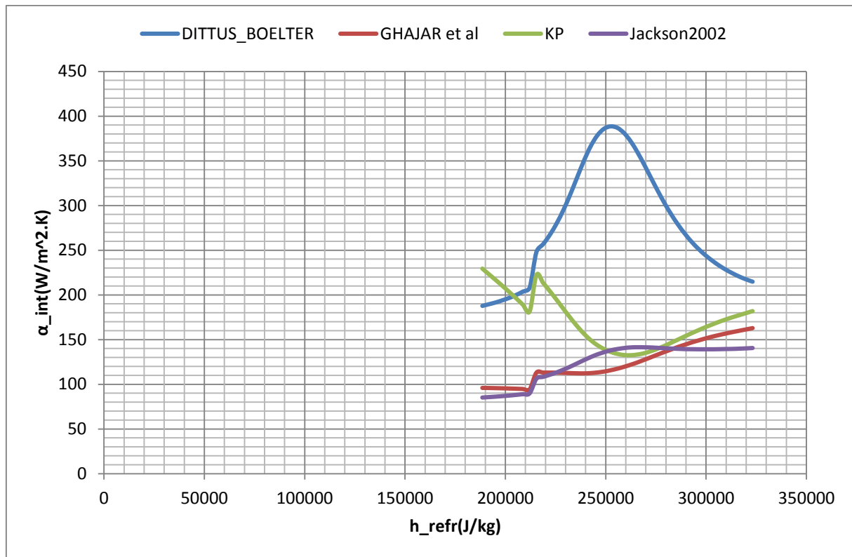
Figure III-10 : Evolution du coefficient d'échange convectif avec différentes corrélations à la pression P = 48\text{bar} .
