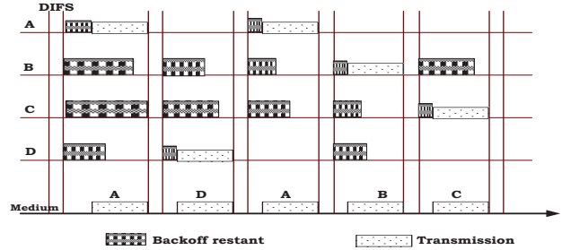
Fig.6 : Opération basique du CSMA/CA
