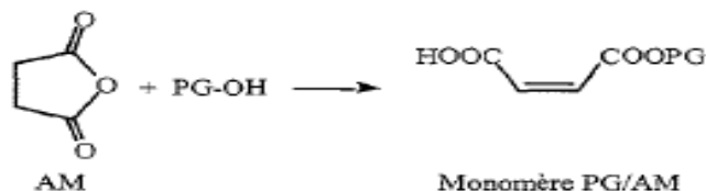
Figure 1. Réaction entre le polyglycérol et l'anhydride maléique
