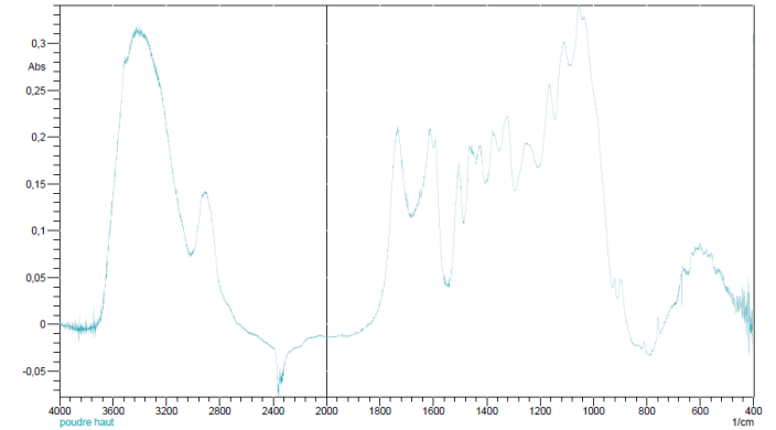
Spectre avec ligne de base modifiée (haut)
