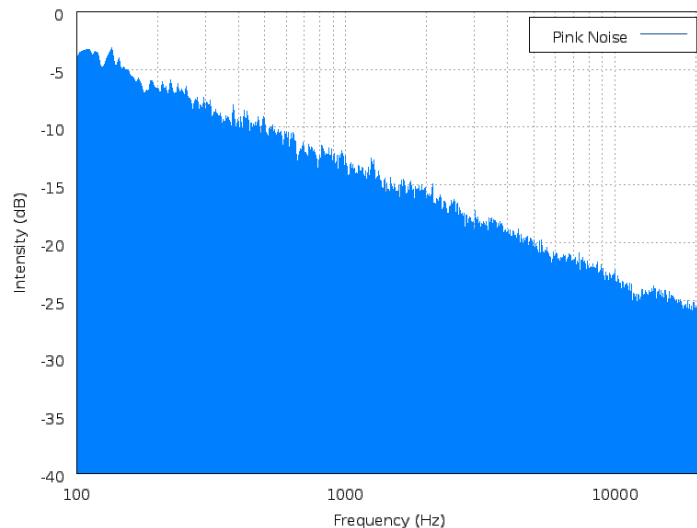
Figure 34 : Spectre du bruit rose [89] Abscisse : fréquence (Hz) ; ordonnée : niveau sonore (dB/Hz)
