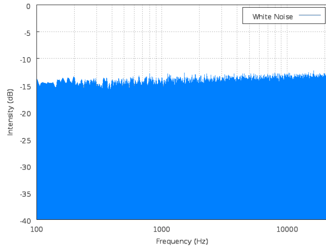
Figure 33 : Bruit blanc [89] Abscisse : fréquence (Hz) ; ordonnée : niveau sonore (dB/Hz)
