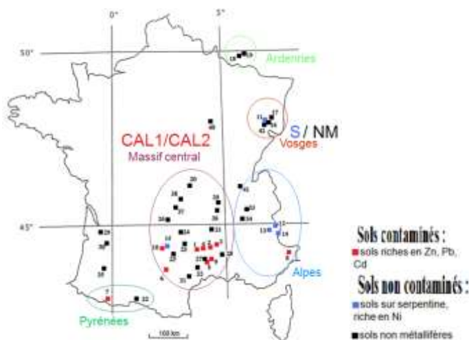
Figure 2 : Localisation des populations de Noccaea caerulescens sur le territoire français (d'après Reeves et al. , 2001)
