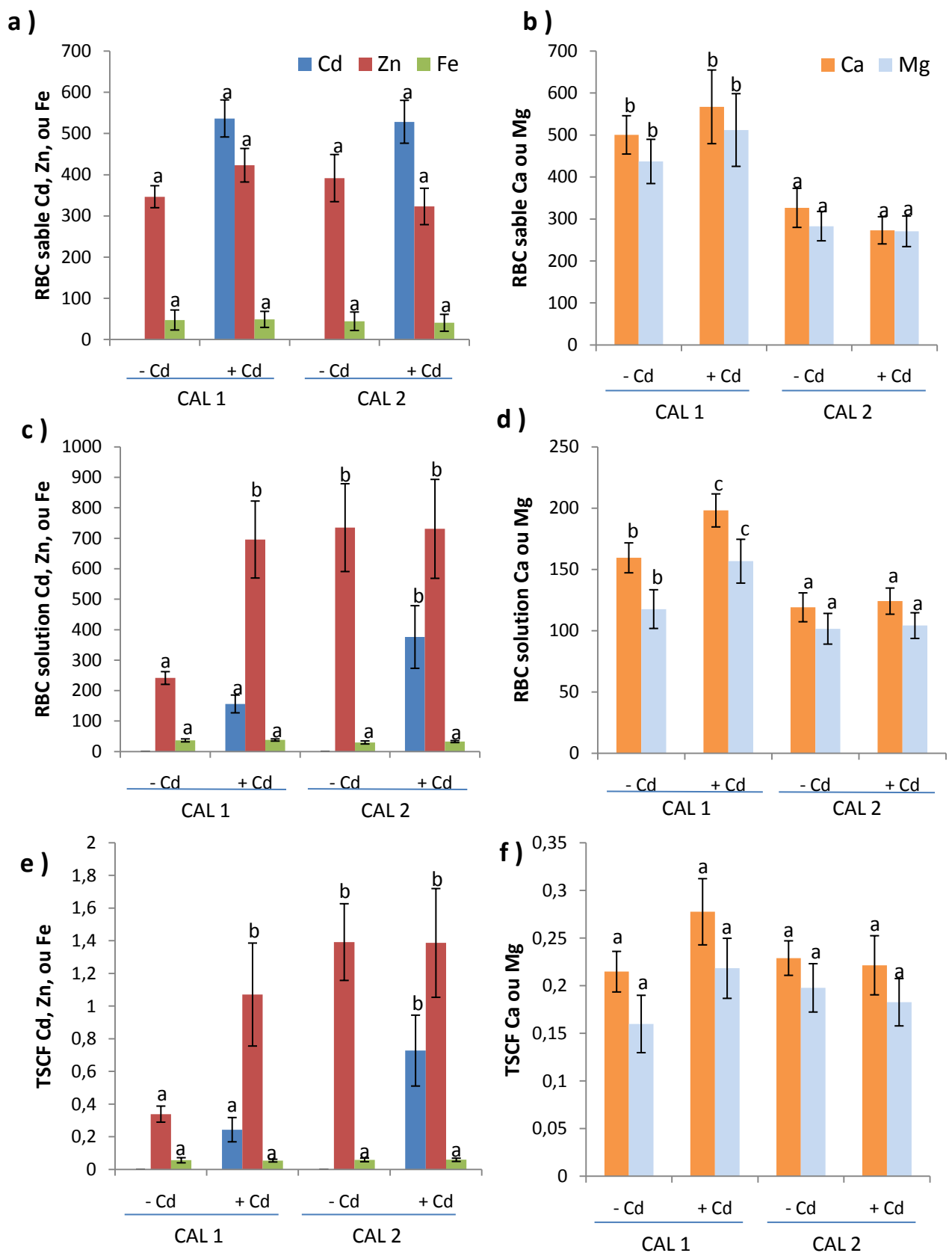
Figure 13 : Facteurs de bioconcentration des métaux Cd, Zn, Fe (a, c, e) et des éléments nutritifs Ca et Mg (b, d, f) dans les feuilles des populations de N. caerulescens CAL1 et CAL2 cultivées sur du sable fertilisé avec (+Cd) et sans (-Cd) cadmium.
