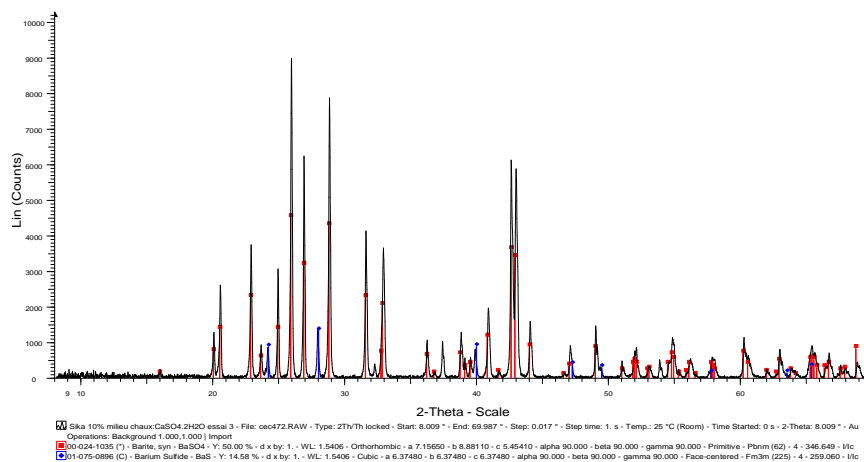
Figure 7: Diffractogramme du précipité Gypse + SP1 à 10% + CaO : présence de BaS
