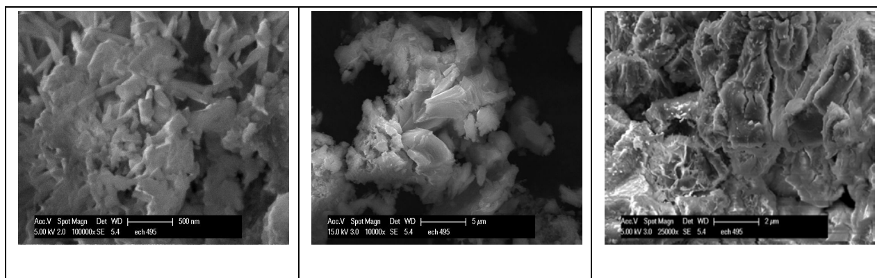
Figure 27 : Micrographies du mélange C_3A cubique + CaSO_4 après 15 min d'hydratation dans de l'eau distillée
