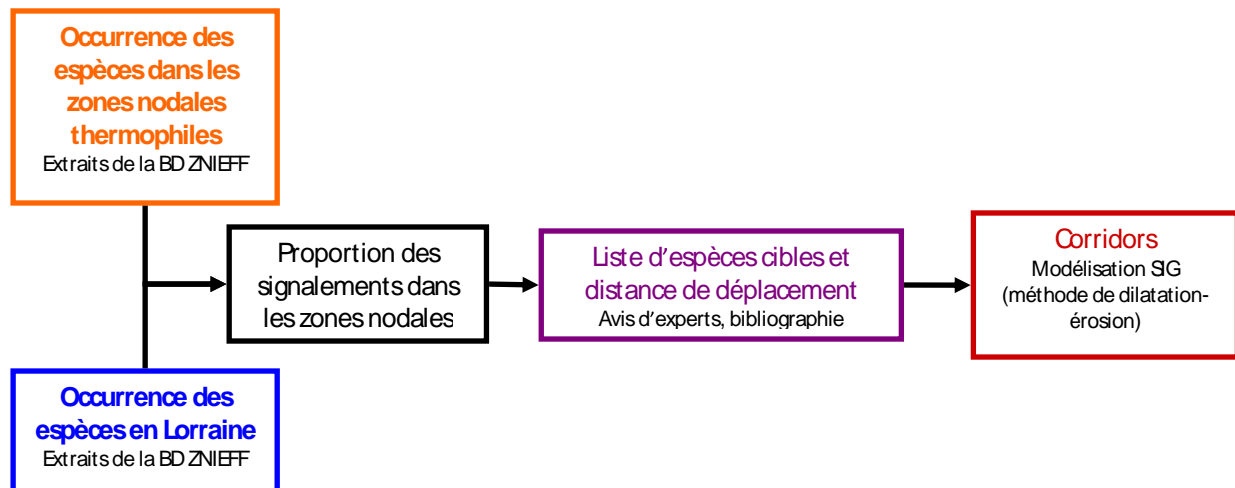
Figure 8: Schéma des étapes de définition des corridors écologiques thermophiles
