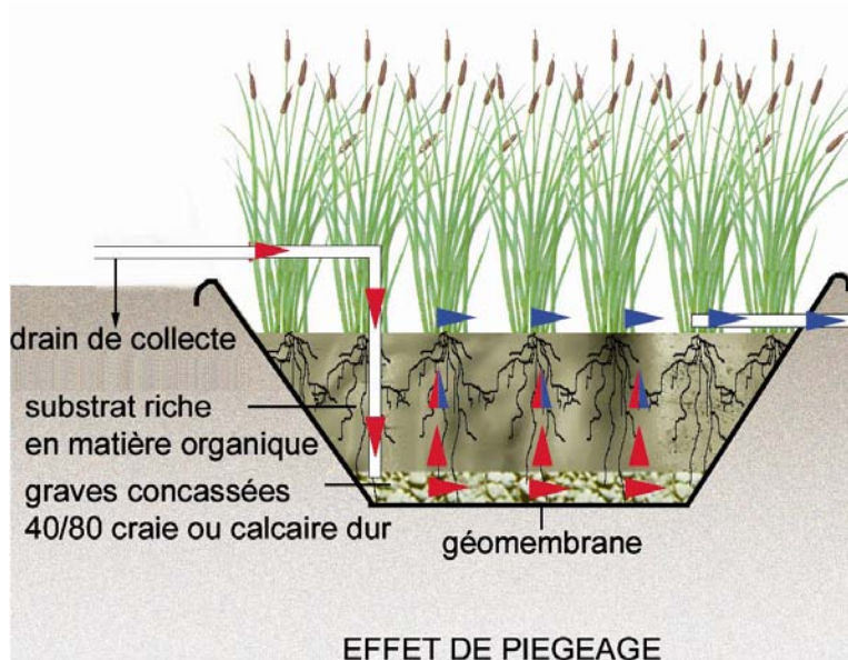
Figure 32 : Filtre de piégeage ascendant (source Phytorestore )
