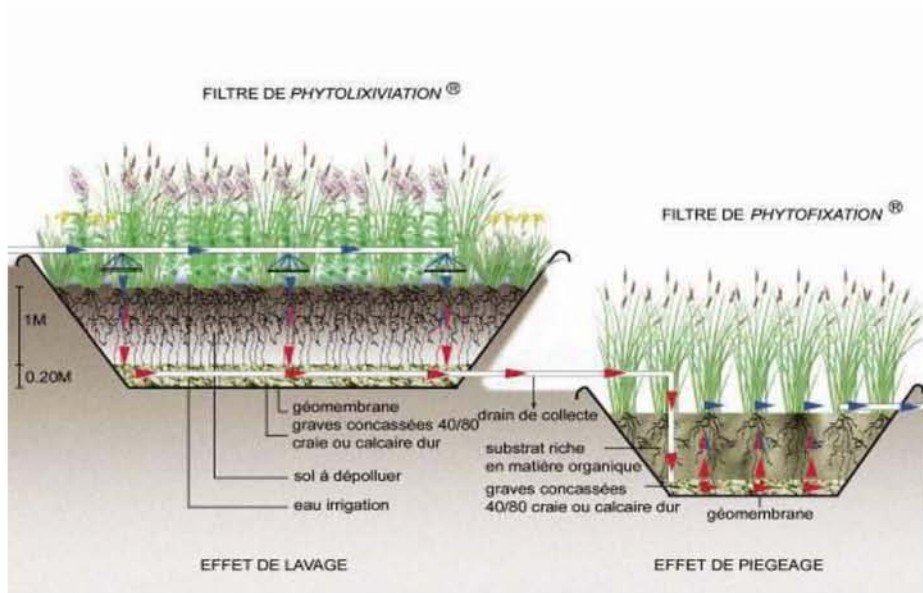
Figure 2 : Coupe type de Jardins Filtrants® boues et Filtre de piégeage (source Phytorestore)
