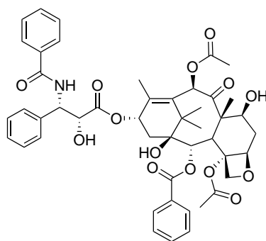
FIGURE 5 – Structure du paclitaxel (taxol).
