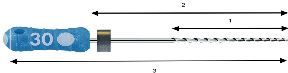
Figure 3 : Représentation des différentes parties qui constituent un instrument manuel de préparation canalair : 1. Lame active, 2. Tige + lame active, 3. Longueur totale de l'instrument (Document personnel).
