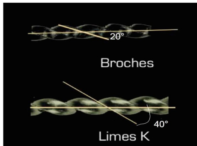
Figure 4 : Représentation de l'angle d'hélice pour les broches et limes K (d'après www.dentalespace.com ).
