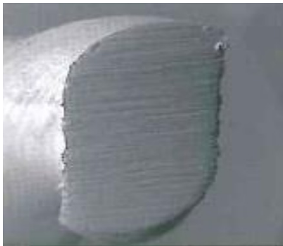
Figure 29 : Section asymétrique du Reciproc® avec deux angles de coupe, observée en microscopie électronique à balayage (Dentsply-VDW®).
