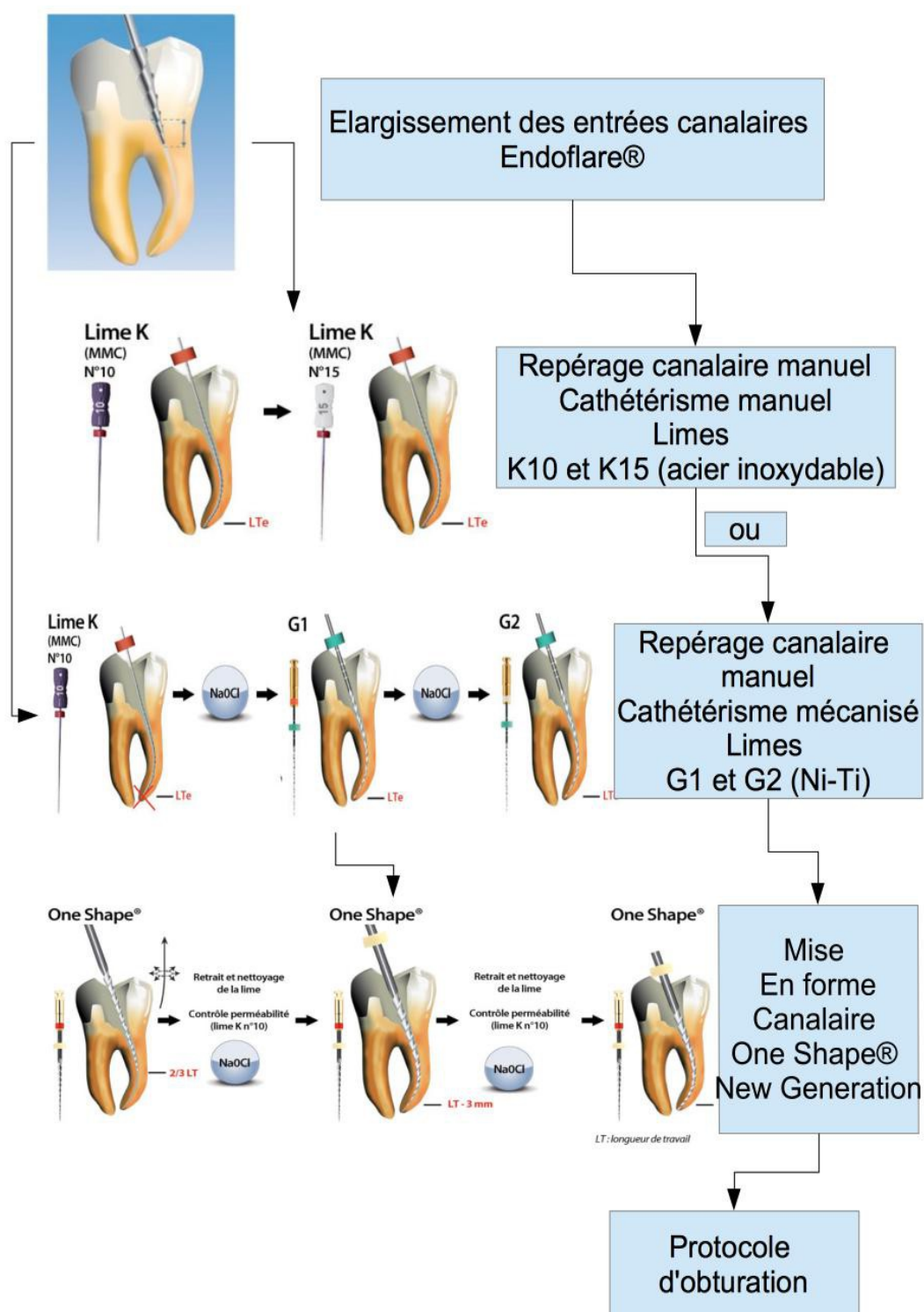
Figure 26 : Schéma récapitulatif du protocole d'utilisation du système One Shape® New Generation (D'après MICRO-MEGA®).
