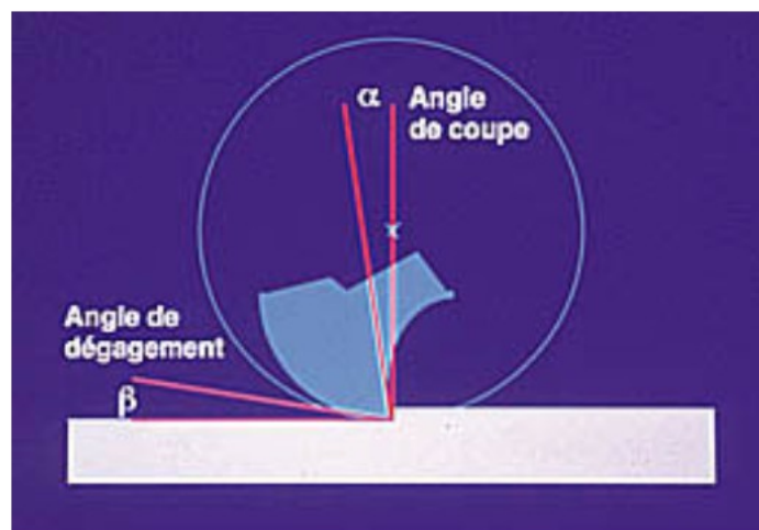
Figure 5: Schéma de l'angle de coupe (Benkirane et coll. , 2001).
