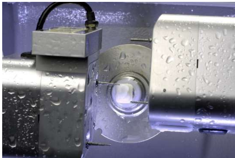
Figure 41: Usinage d'un onlay pour molaire par l'usineuse Mc inlab XI
