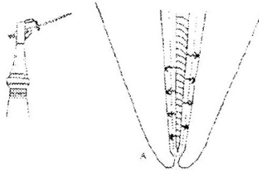
Figure 10 : Mode d'action des instruments soniques (source : Marmotte 2000)
