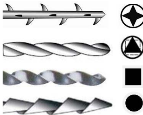
Figure 4 : Les différents instruments manuels et leur section respective (de haut en bas : le tire-nerf, la broche, la lime K et MMC®, la lime H ou racleur et MME®)
