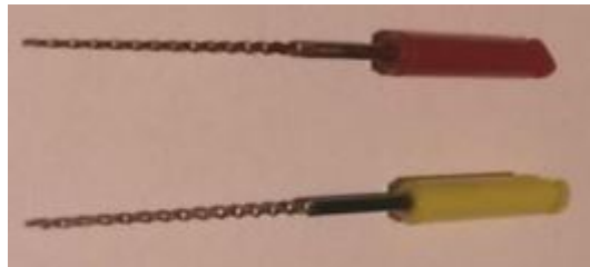
Figure 28 : Photo des broches MICRO-MEGA® en CuAlBe monocristallin (au-dessus) et NiTi polycristallin (en dessous)
