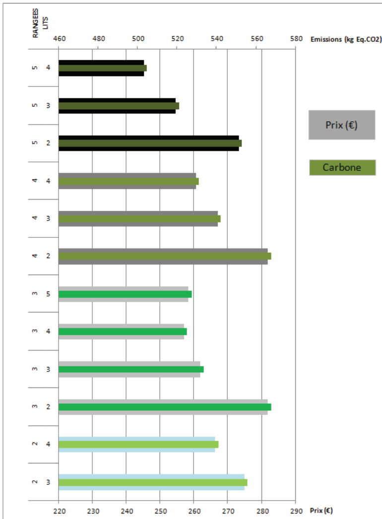
Émissions et prix de la poutre en fonction du nombre de rangées et de lits de barres.
