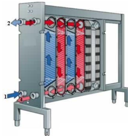
Figure 11 : Principe de fonctionnement d'un échangeur à plaques
