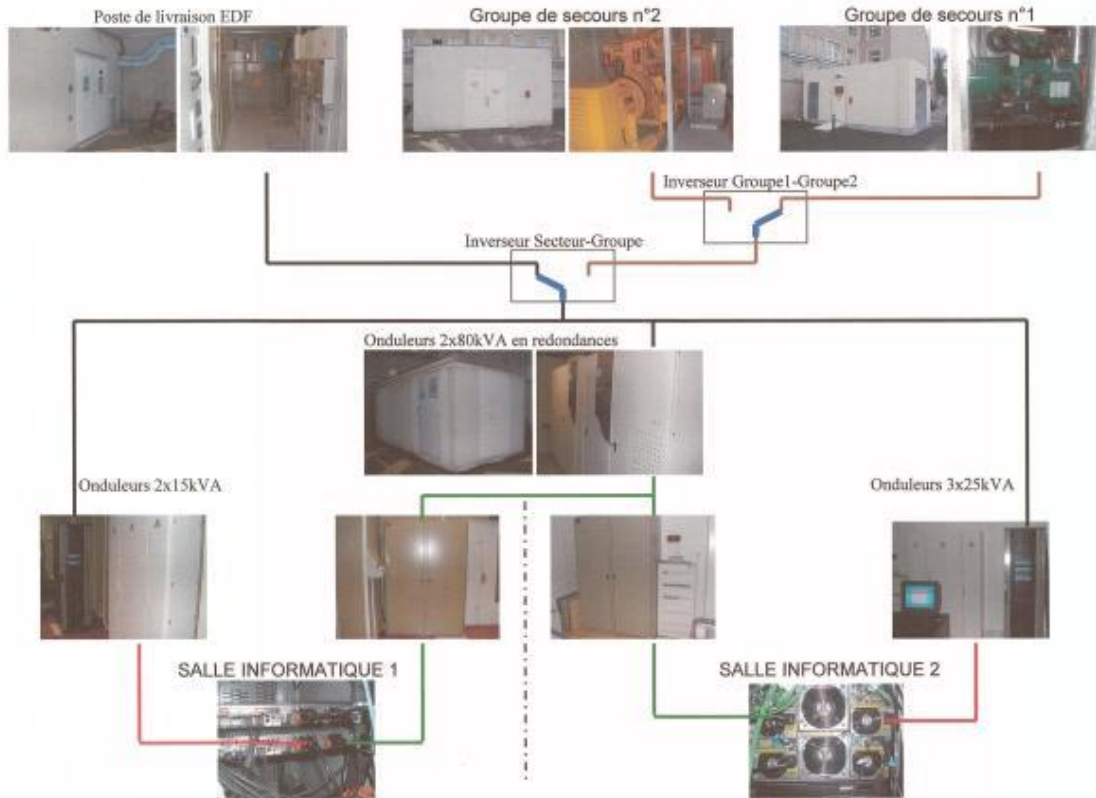
Schéma de l'installation électrique à Marin
