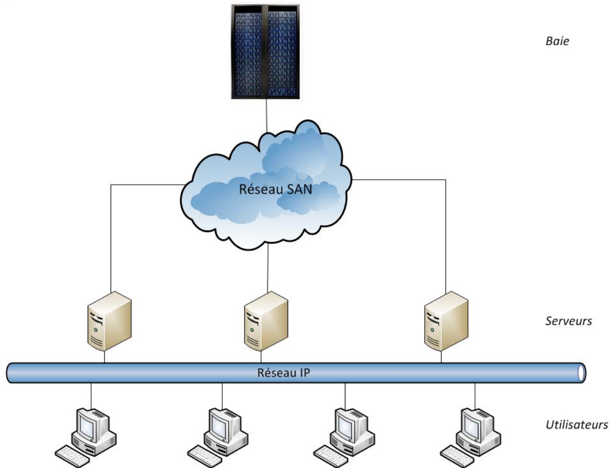
Schéma de principe d'une architecture SAN
