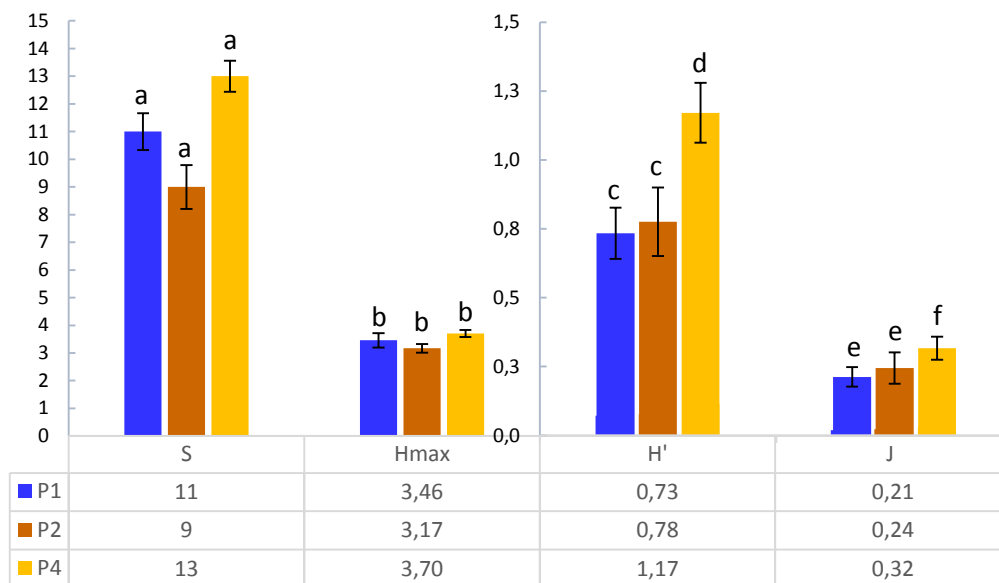
Figure 7 : Histogrammes des indices de diversité (+/- SEM), calculés pour le passage 1 (juin-juillet 2013) : Richesse spécifique ( S ), Indices de diversité de Shannon-Weaver ( H' ) et de diversité maximale ( H_{max} ), Indices d'équitabilité de Pielou ( J ).
