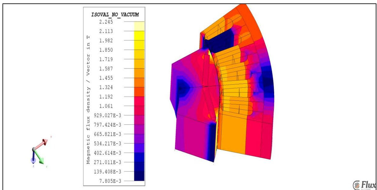
Fig4.5 Dégradé d'induction
