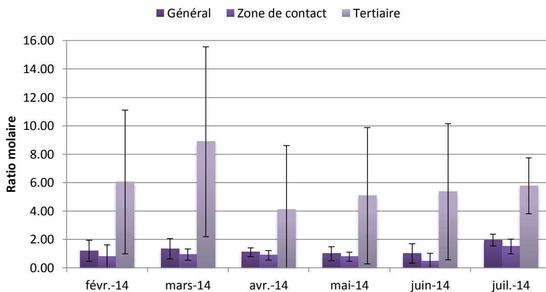
Figure 12: Ratio molaire Fe/P entre les mois de février et juillet 2014.
