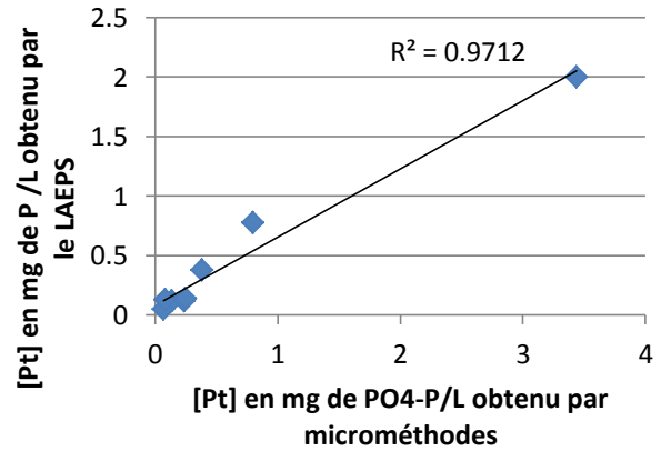
Figure 10: Concentrations en Pt en sortie de station.
