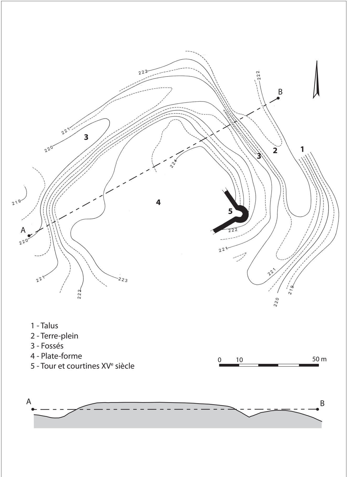
Fig. 7 : Haboudange, château XII e -XV e siècle (plan réalisé par G. Giuliano et Cl. Voignier, 1992)
