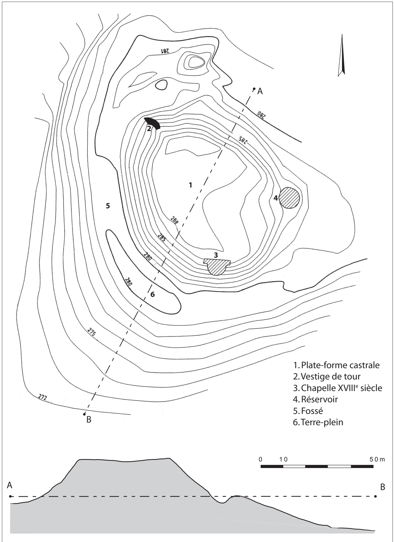
Fig. 8 : Château de Marimont-lès-Bourdonnay, XII e -XV e siècle (plan réalisé par G. Giuliano et P. Rholes, 1992)
