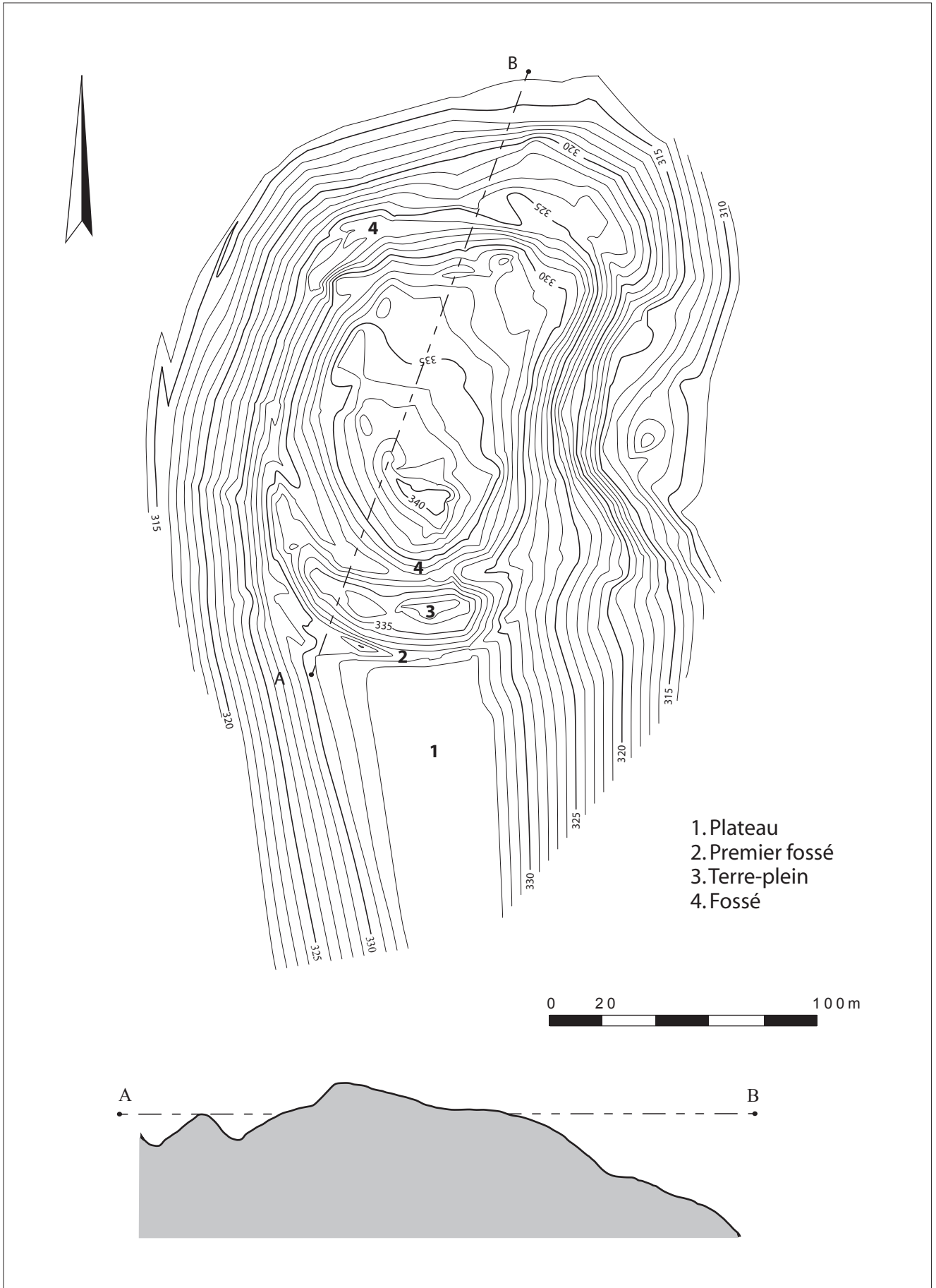
Fig. 9 : Marimont-lès-Bénéstroof, château XI e -XV e siècle, (plan réalisé par G. Giuliano, Ch. Kraemer et Cl. Voignier, 1998)
