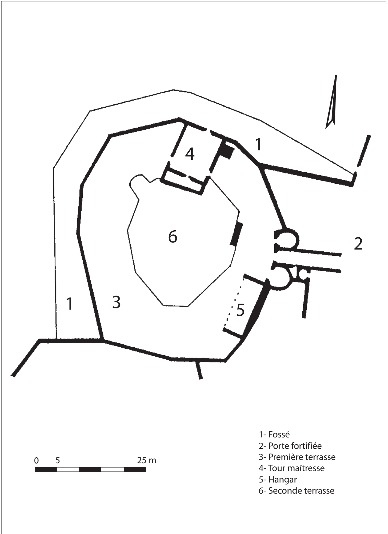
Fig. 6 : Château de Dombasle, plan d'après Henri Lepage, 1862 (dessin réalisé par G. Giuliano, 1992)
