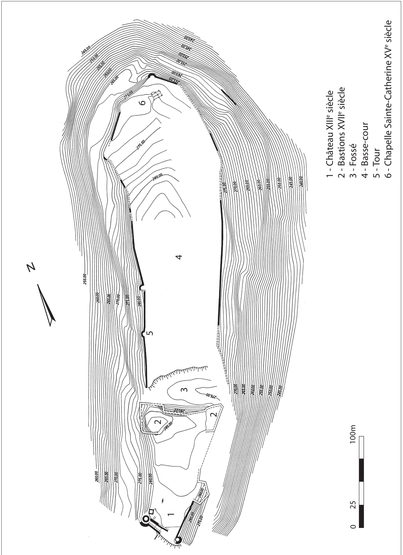
Fig. 12 : Hombourg-Haut, château XIII e -XVII e siècle (plan réalisé par G. Giuliano et Cl. Voignier, 1992)
