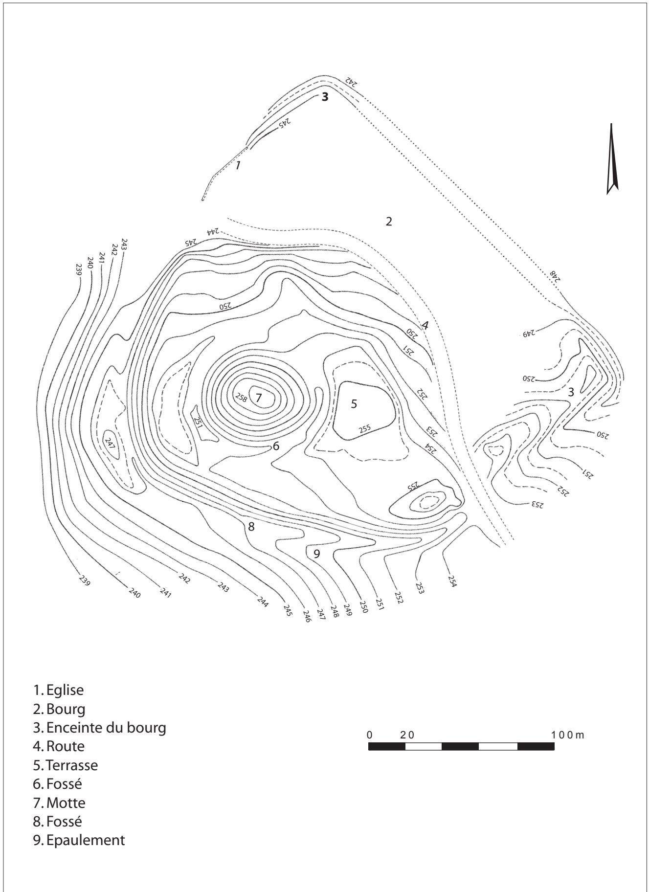
Fig. 2 : Fribourg, motte et enceinte villageoise (plan réalisé par Cl. Voignier et G. Giuliani, 1992)
