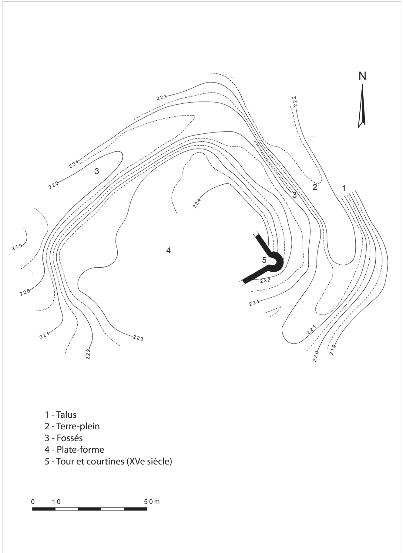
Fig. 13 : Haboudange, château XIII e -XVII e siècle (plan réalisé par G. Giuliano et Cl. Voignier, 1994)
