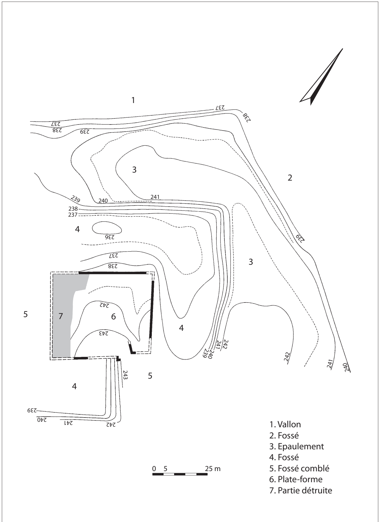
Fig. 14 : Albestroff, château XIII e -XVIII e siècle (plan réalisé par G. Giuliano et Cl. Voignier, 1994)
