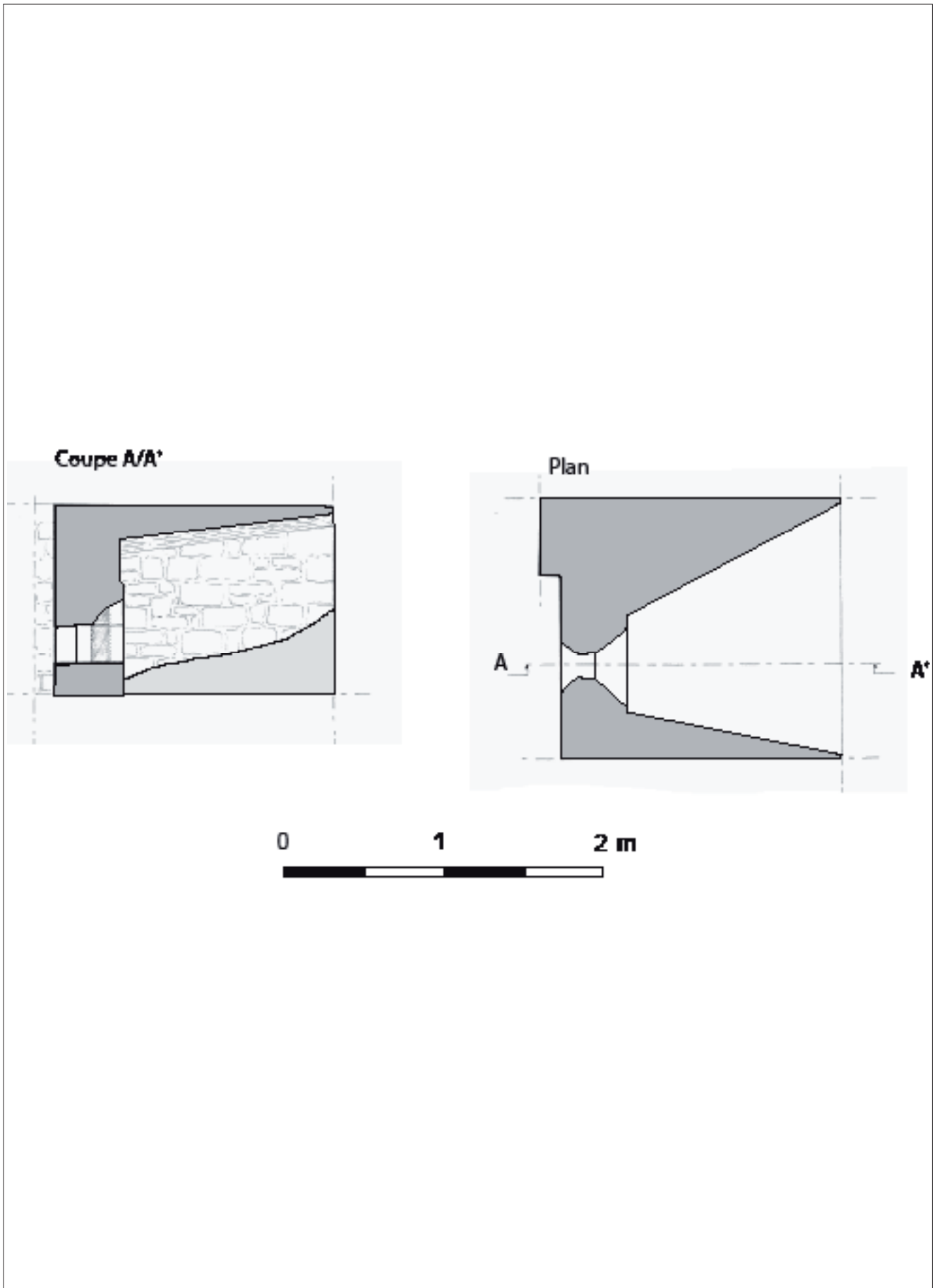
Fig. 6 : Custines, canonnière de la barbancane, XVI e siècle (dessin G. Giuliano, E. Badonnel, 1997)
