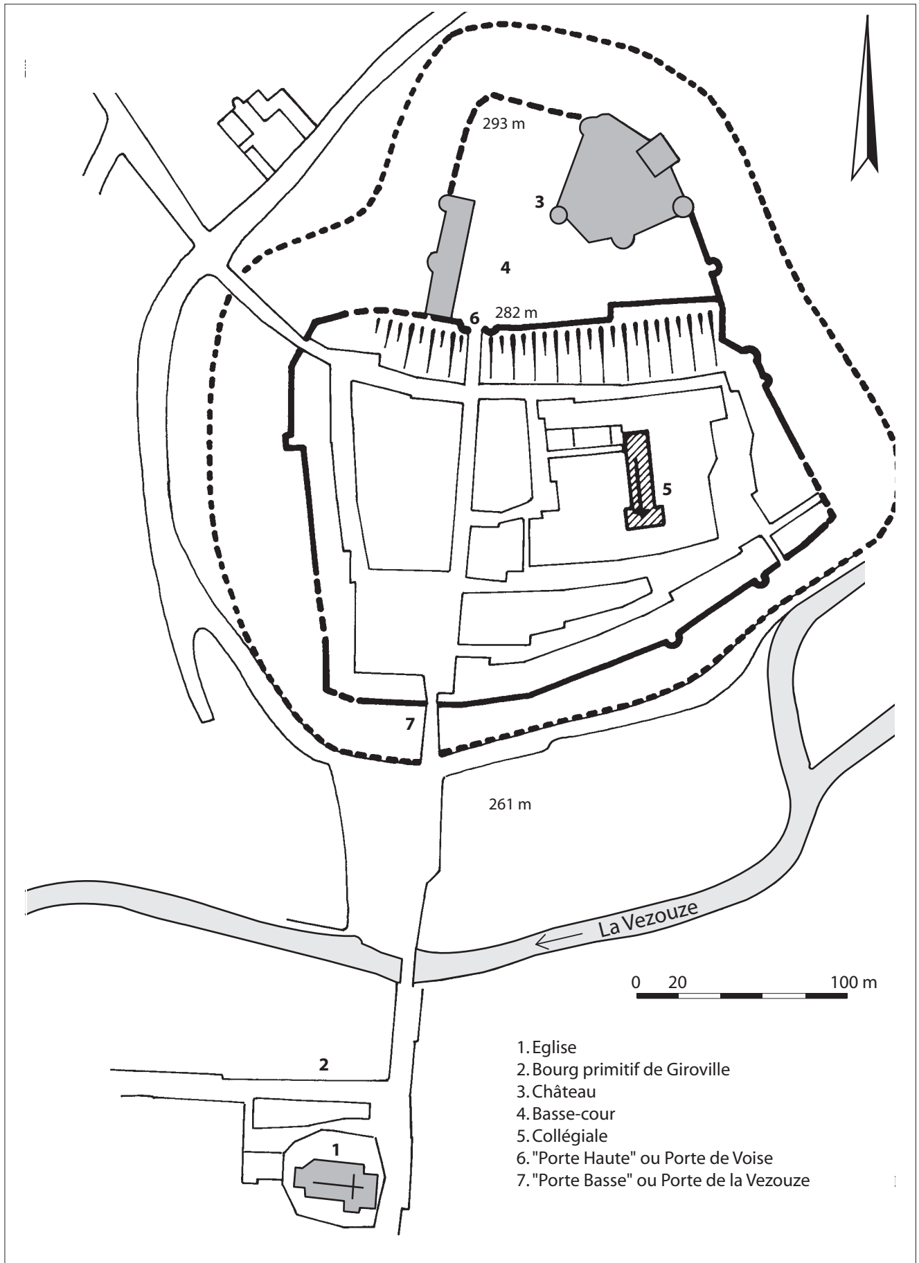
Fig. 2 : Blâmont, plan d'ensemble d'après le cadastre de 1819 (plan réalisé par G. Giuliano)
