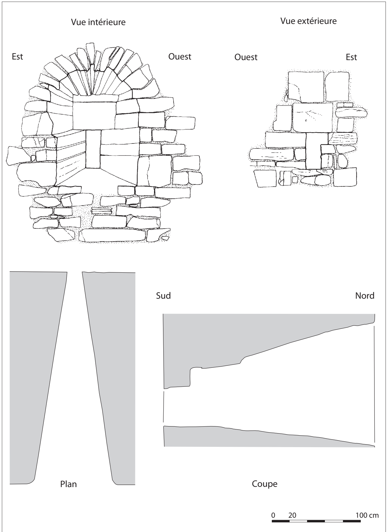
Fig. 6 : Château de Blâmont, donjon XII e siècle, fenêtre sud, premier étage (dessin L.A.M.Est, 2004)
