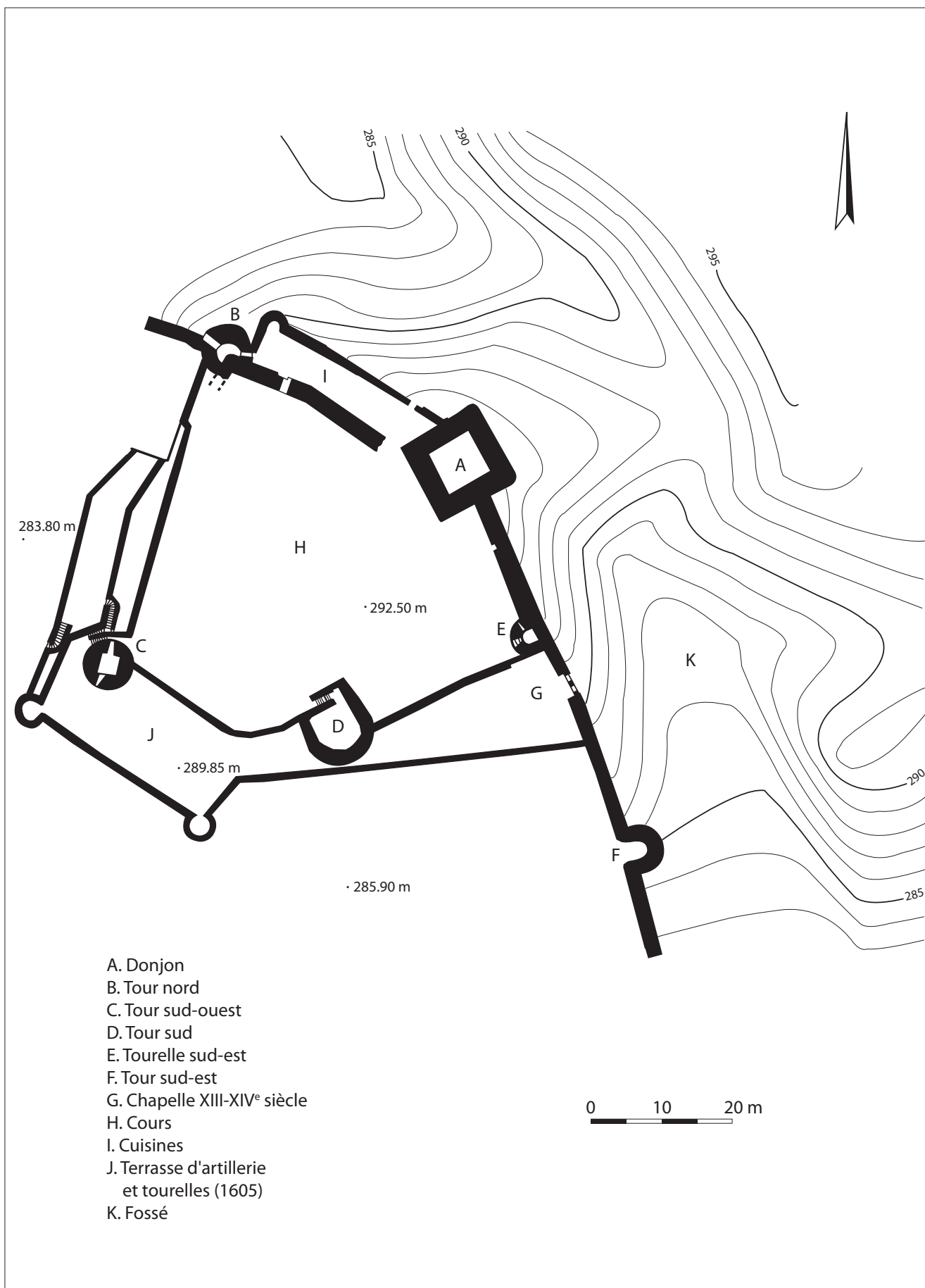
Fig. 4 : Château de Blâmont, XII e -XVII e siècle (plan réalisé par G. Giuliano et Cl. Voignier, 1990)
