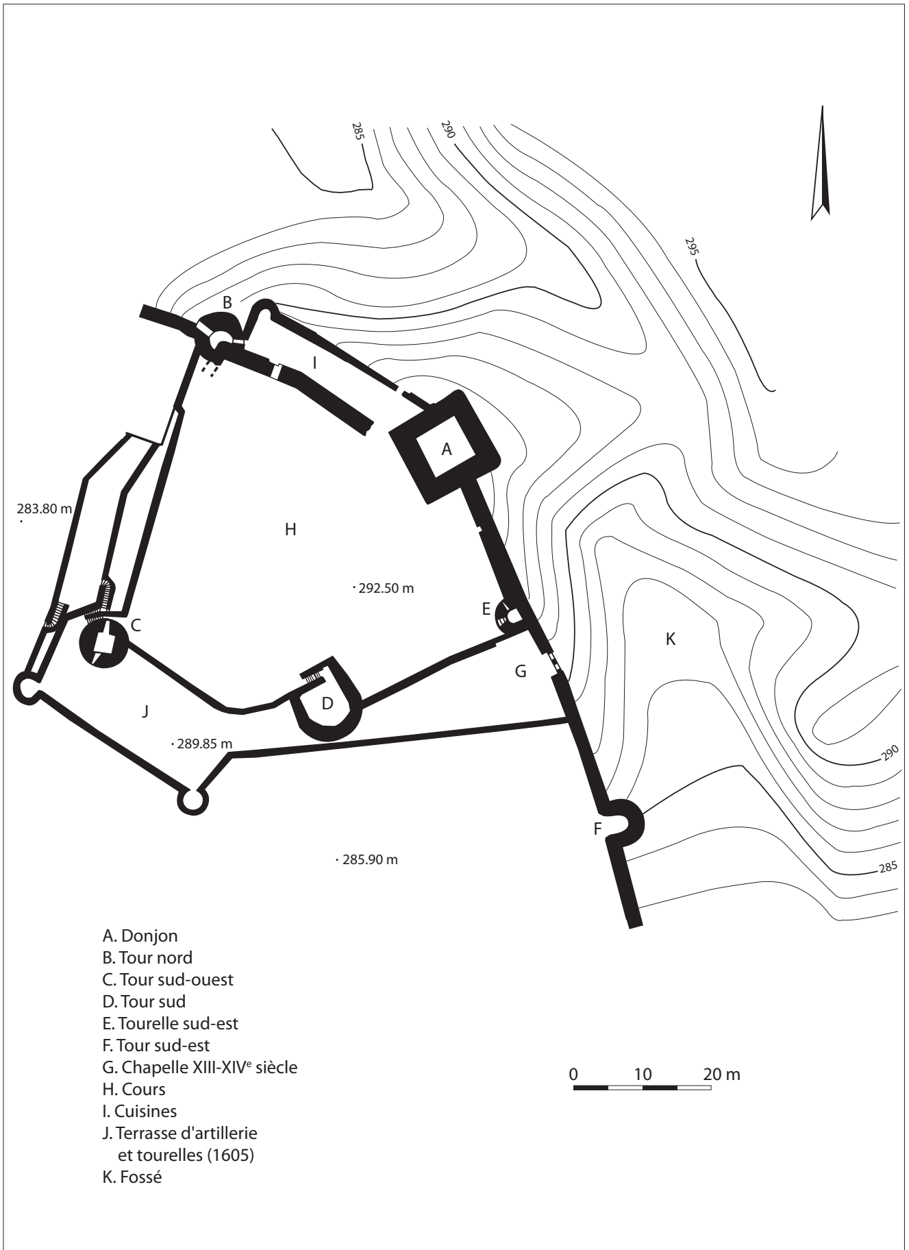
Fig. 4 : Château de Blâmont, XII e -XVII e siècle (plan réalisé par G. Giuliano et Cl. Voignier, 1990)
