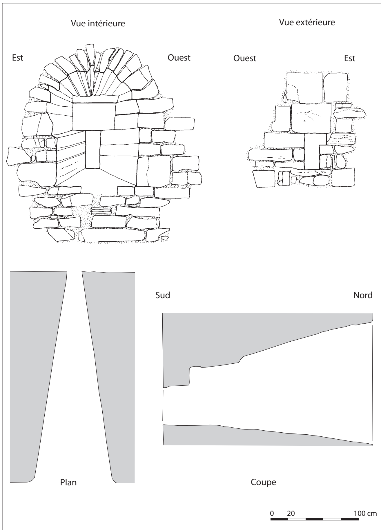
Fig. 6 : Château de Blâmont, donjon XII e siècle, fenêtre sud, premier étage (dessin L.A.M.Est, 2004)
