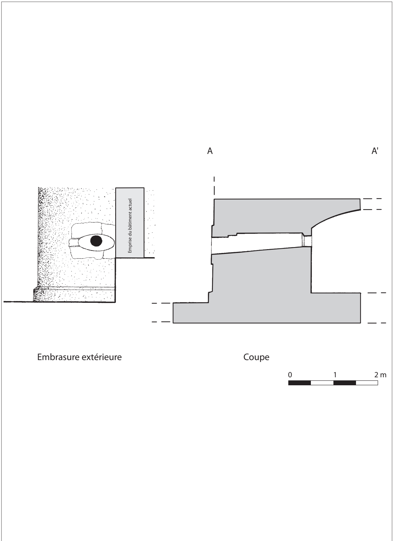
Fig. 11 : Château de Blénod-lès-Toul, canonnière de la tour nord-est (dessin de B. Willaime et G. Giuliani, 2001)
