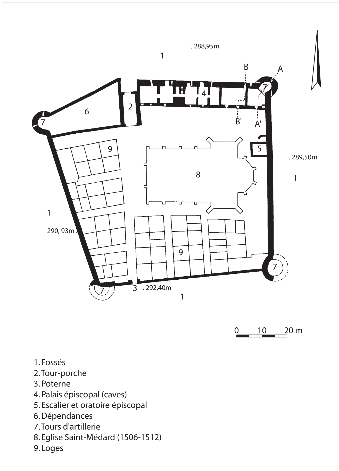
Fig. 5: Château de Blénod-lès-Toul, plan général (plan réalisé par G. Giuliano, Ch. Kraemer, Cl. Voignier et collaborateurs, 1998)
