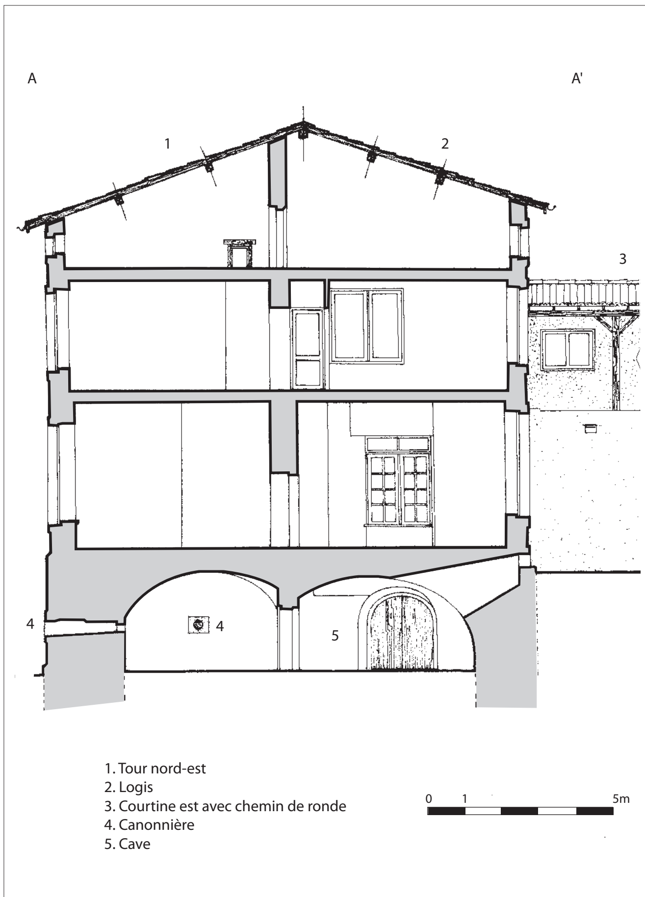
Fig. 10 : Château de Blénod-lès-Toul, palais épiscopal, tour nord-est, coupe AA' (dessin réalisé par B. Willaime et G. Giuliano, 2001)
