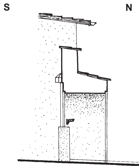
Coupe
