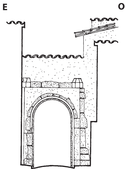
Élévation extérieure
