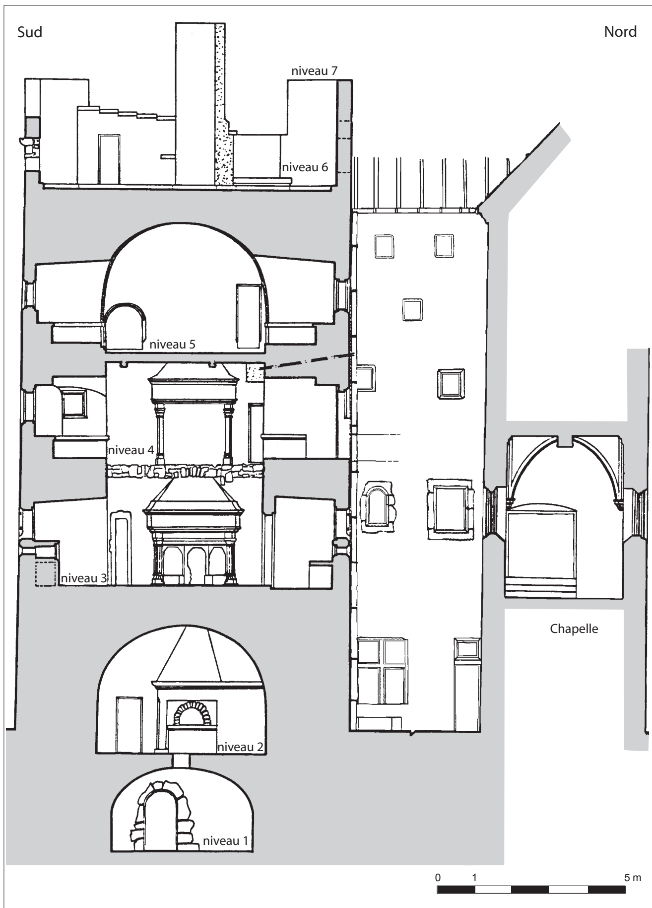
Fig. 22 : Aulnois-sur-Seille, Moselle, maison forte XV e -XVI e siècle, coupe (dessin de B. Willaime et G. Giuliato, 1998)
