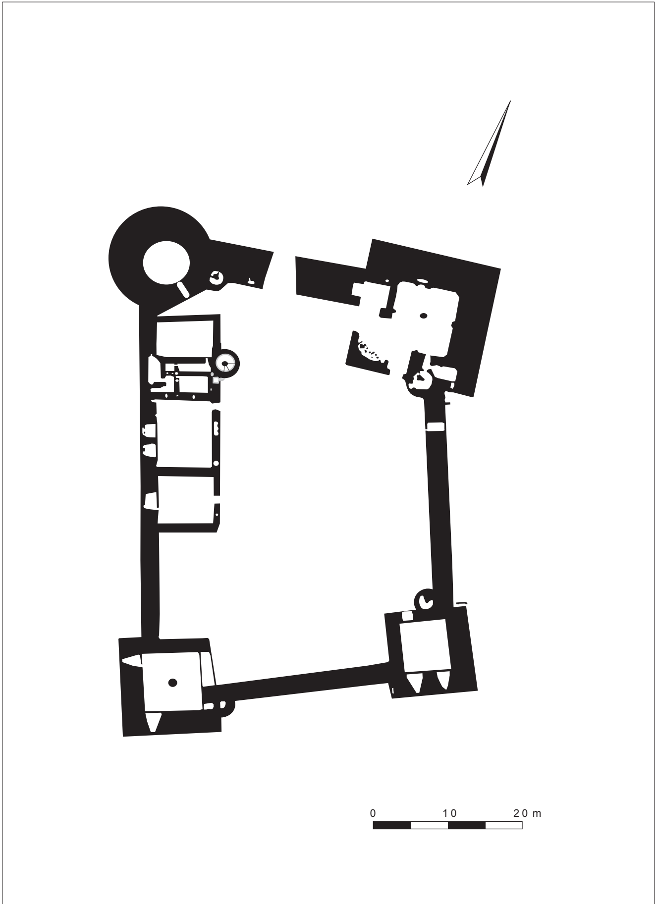
Fig. 16: Manderen, Moselle, plan général (plan réalisé par Ch. Kraemer et B. Fajal, 1986)
