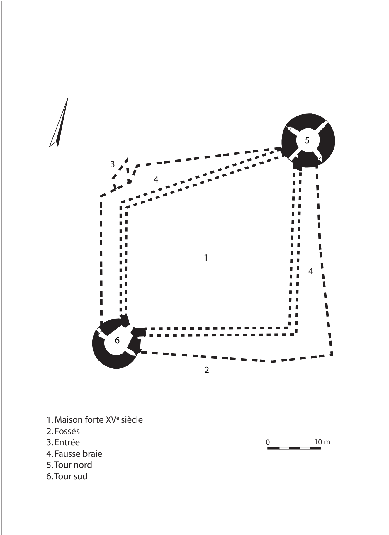
Fig. 24 : Ogeville, Meurthe-et-Moselle, plan général de la maison forte (plan réalisé par Cl. Voignier et G. Giuliani)
