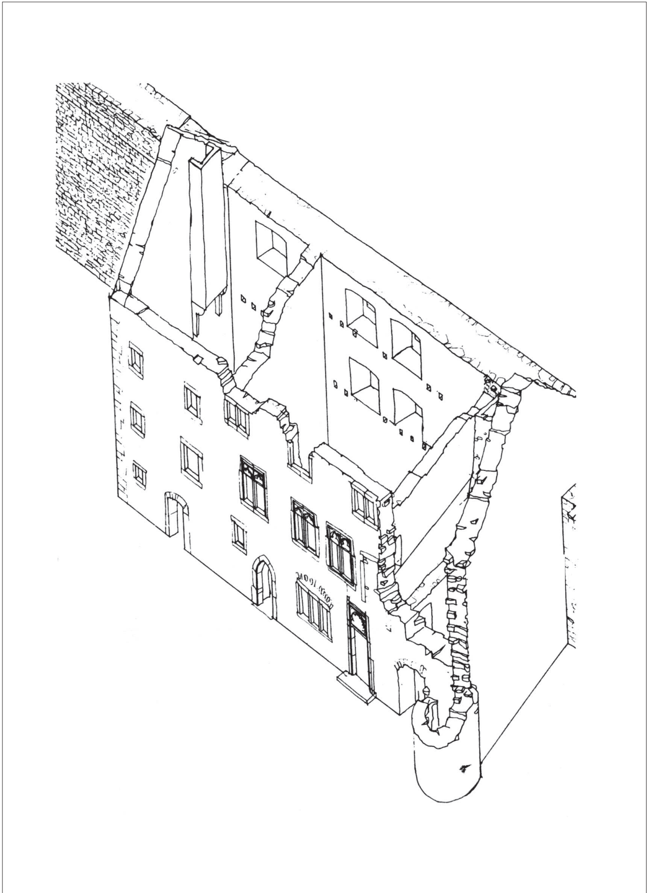
Fig. 18 : Manderen, Moselle, axonométrie du logis oriental d'après D. Gaymard (DRAC Lorraine)
