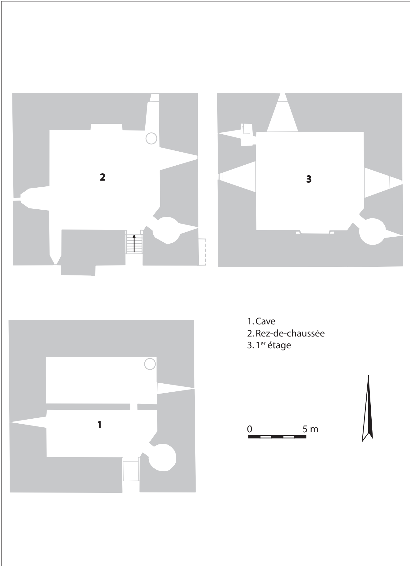
Fig. 19 : Port-sur-Seille, Meurthe-et-Moselle, plans des trois niveaux du donjon (plan réalisé par Cl. Voignier et G. Giuliano, 1980)
